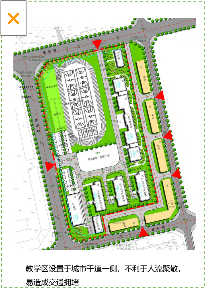
图3-20 出入口反面案例示意
