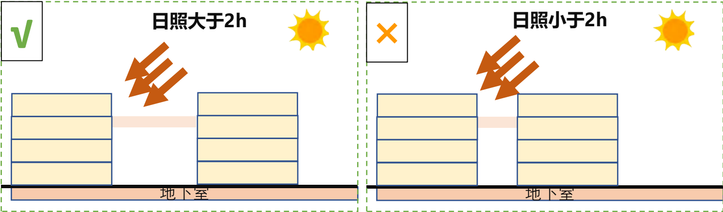
图3-23 日照分析示意图
