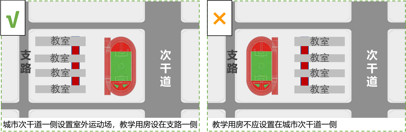
图3-25 运动场布局示意图
