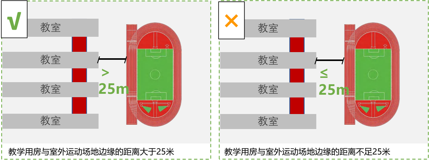
图3-26 运动场与教学楼间距示意图
