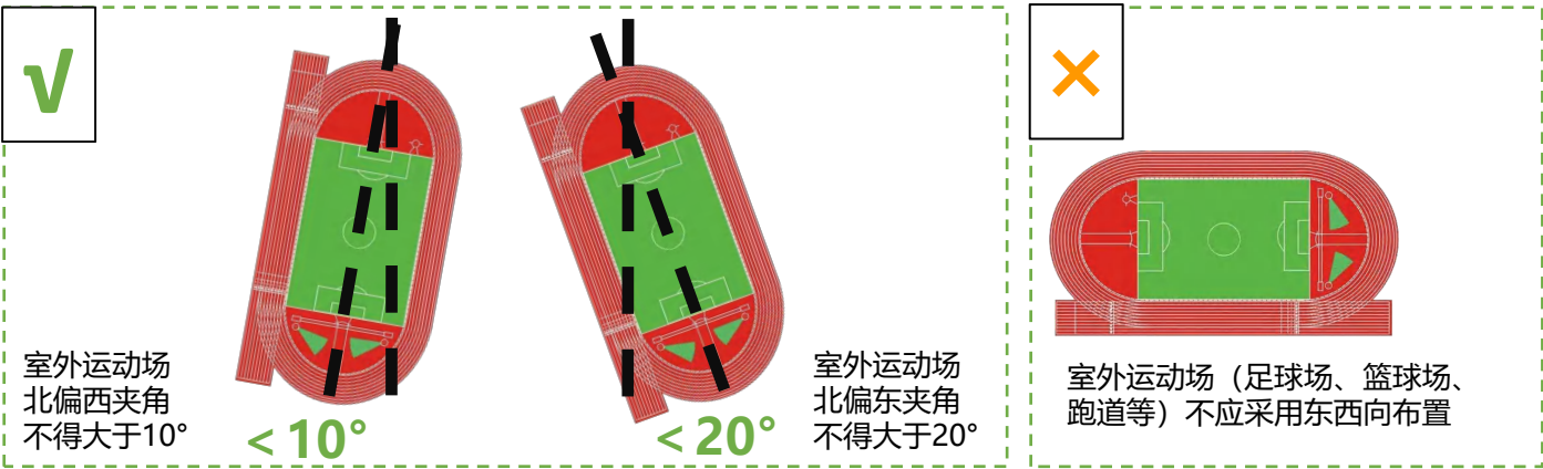
图3-27 运动场朝向示意图
