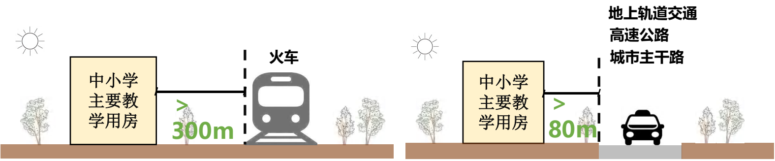
图3-12 教学用房退让道路示意图
