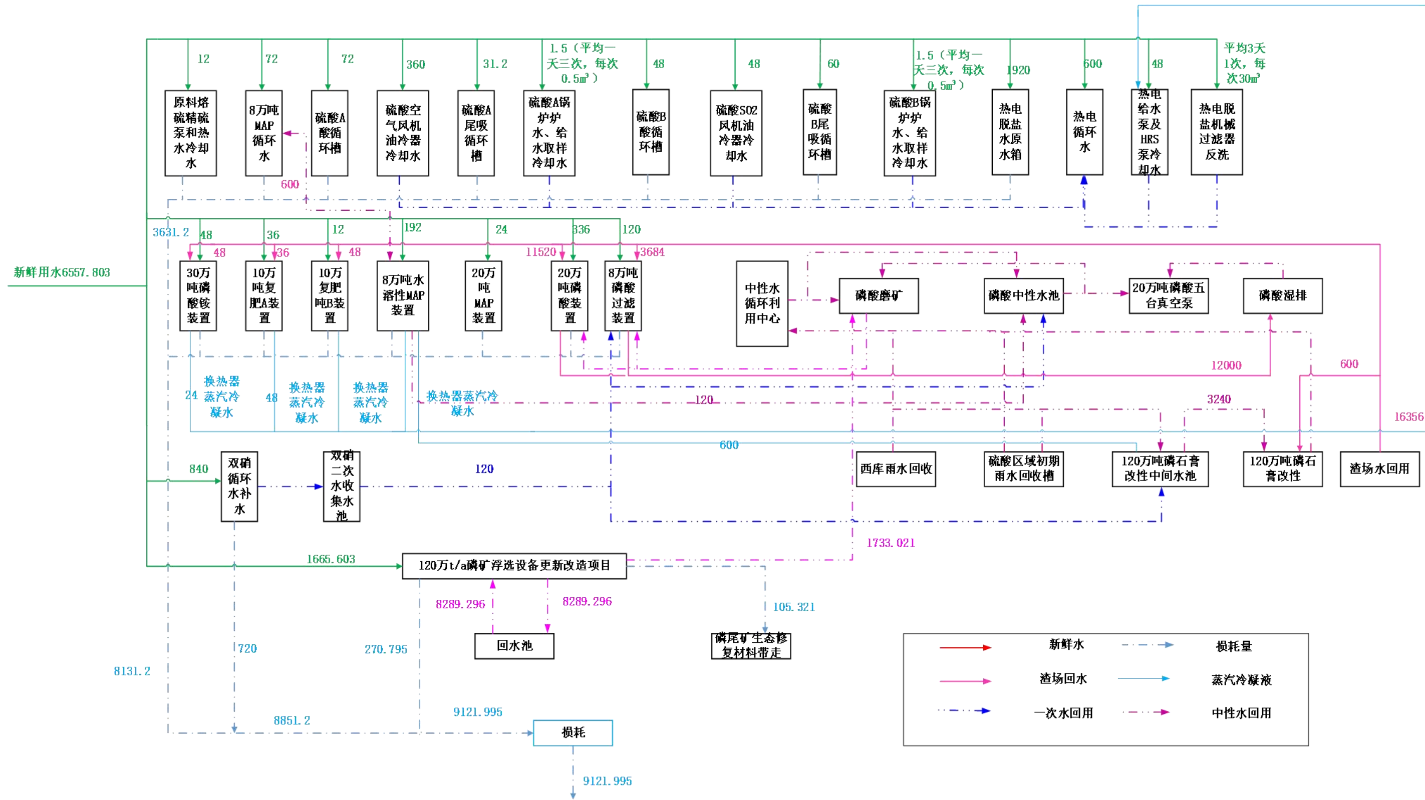
图 4.8.1-1 项目扩建后全厂水平衡 (m³/d)
