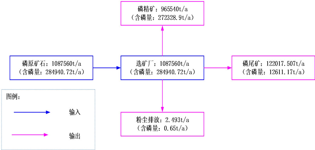
图 4.3.2-2 项目磷平衡图（干基）
