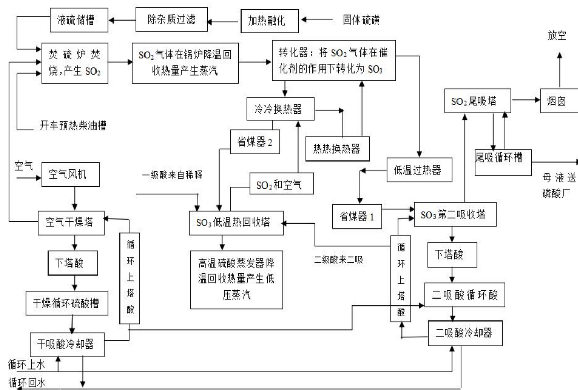
图 2.5.1-2 30 万吨 B 系列硫酸生产工艺流程图
