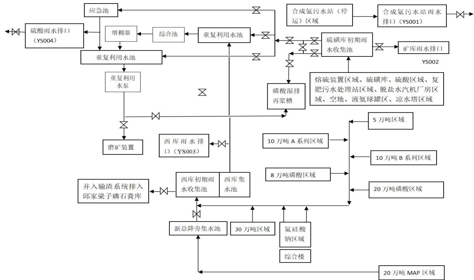
图 2.9.2-1 厂区初期雨水收集管网走向图
