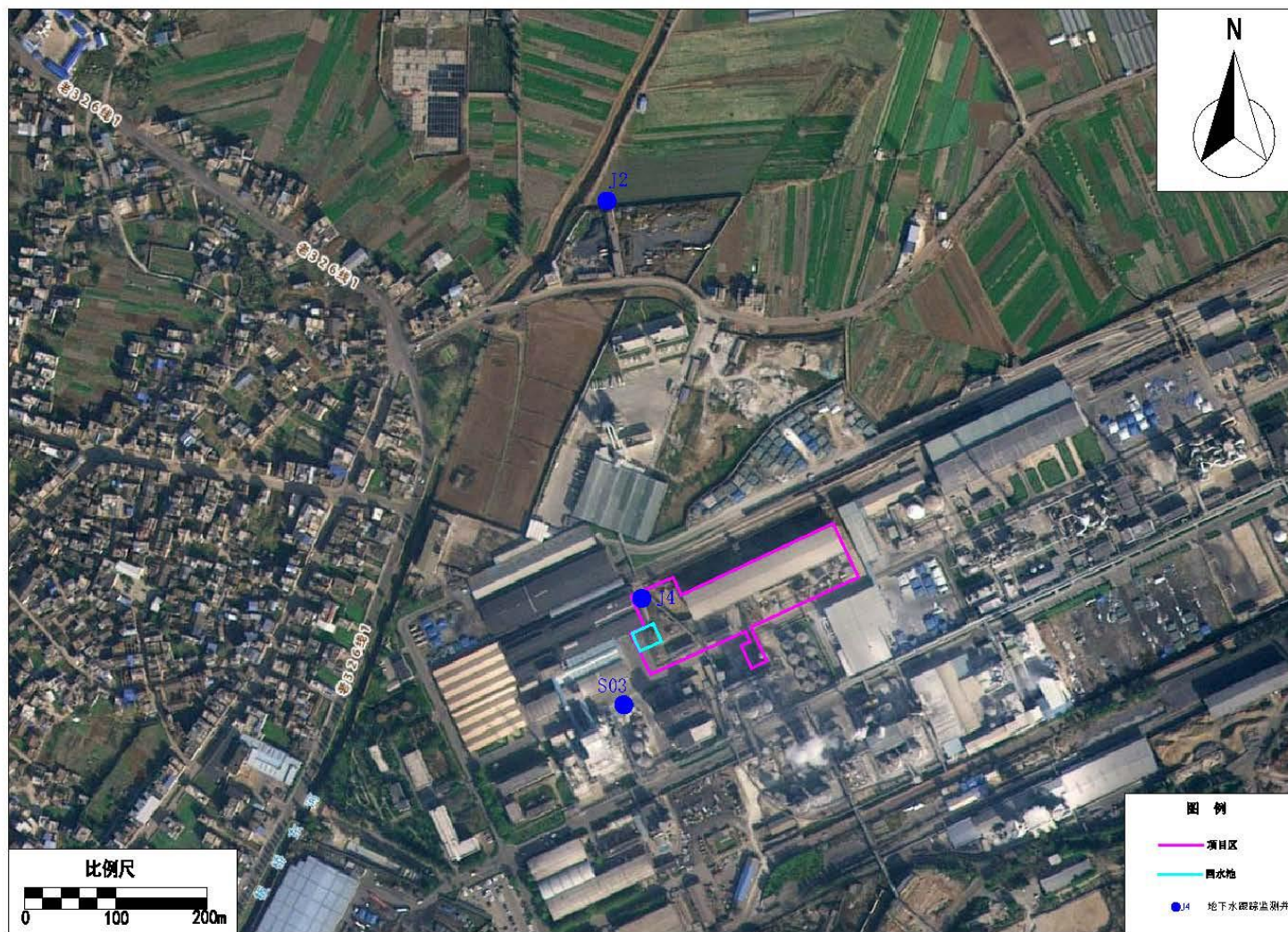
图 6.2.3-12 项目区地下水长期监测井分布图
