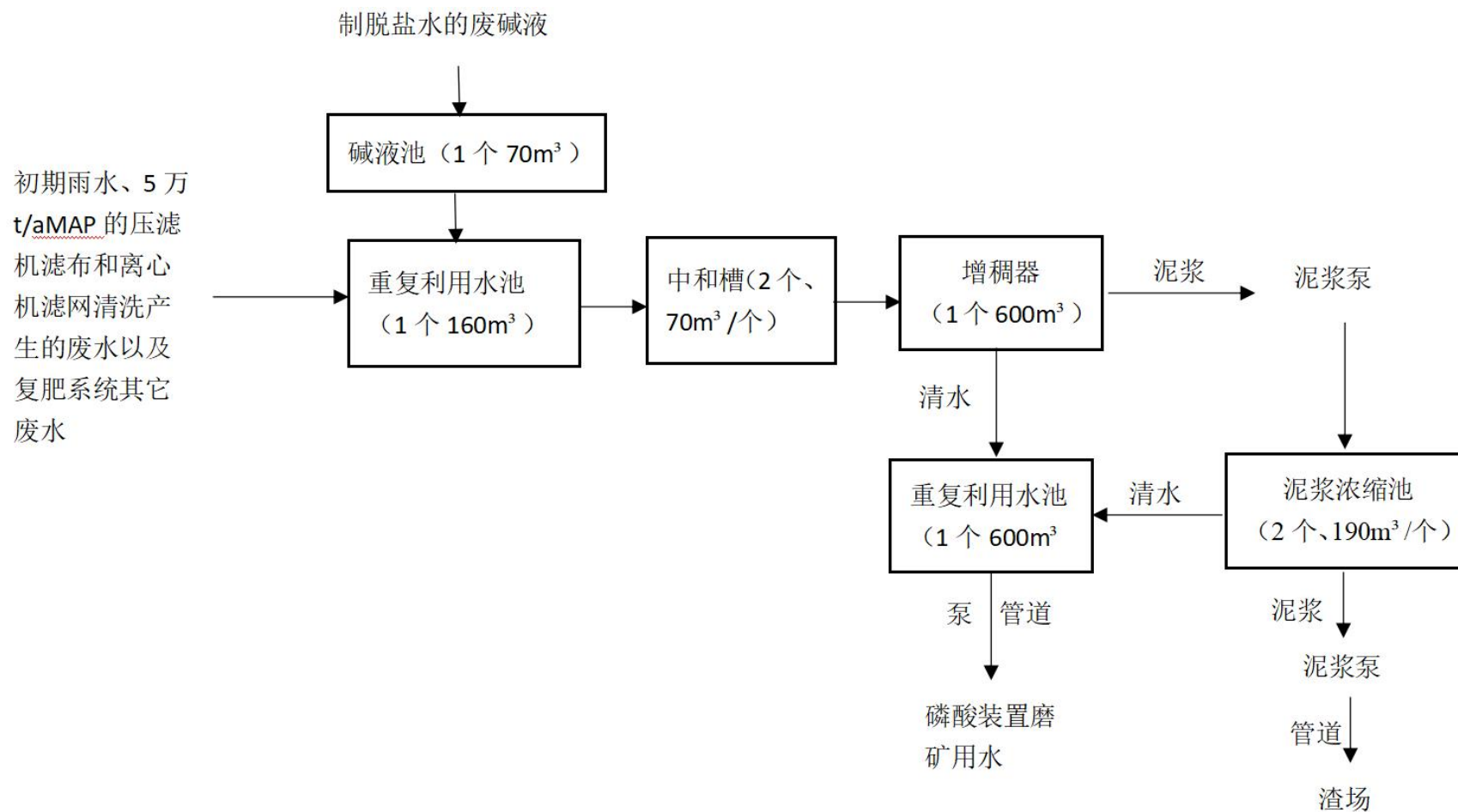
图 2.9.3-1 复肥污水处理站工艺流程图
