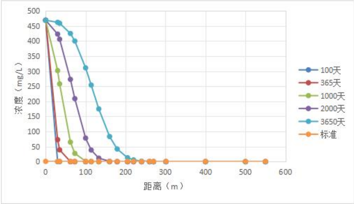
图 6.2.3-6 项目回水池泄漏总磷浓度扩散曲线图
