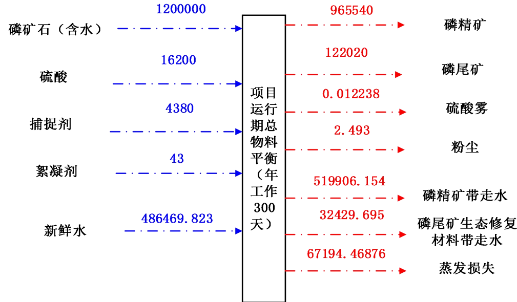
图 4.3.2-1 选厂物料平衡图示意图单位: t/a
