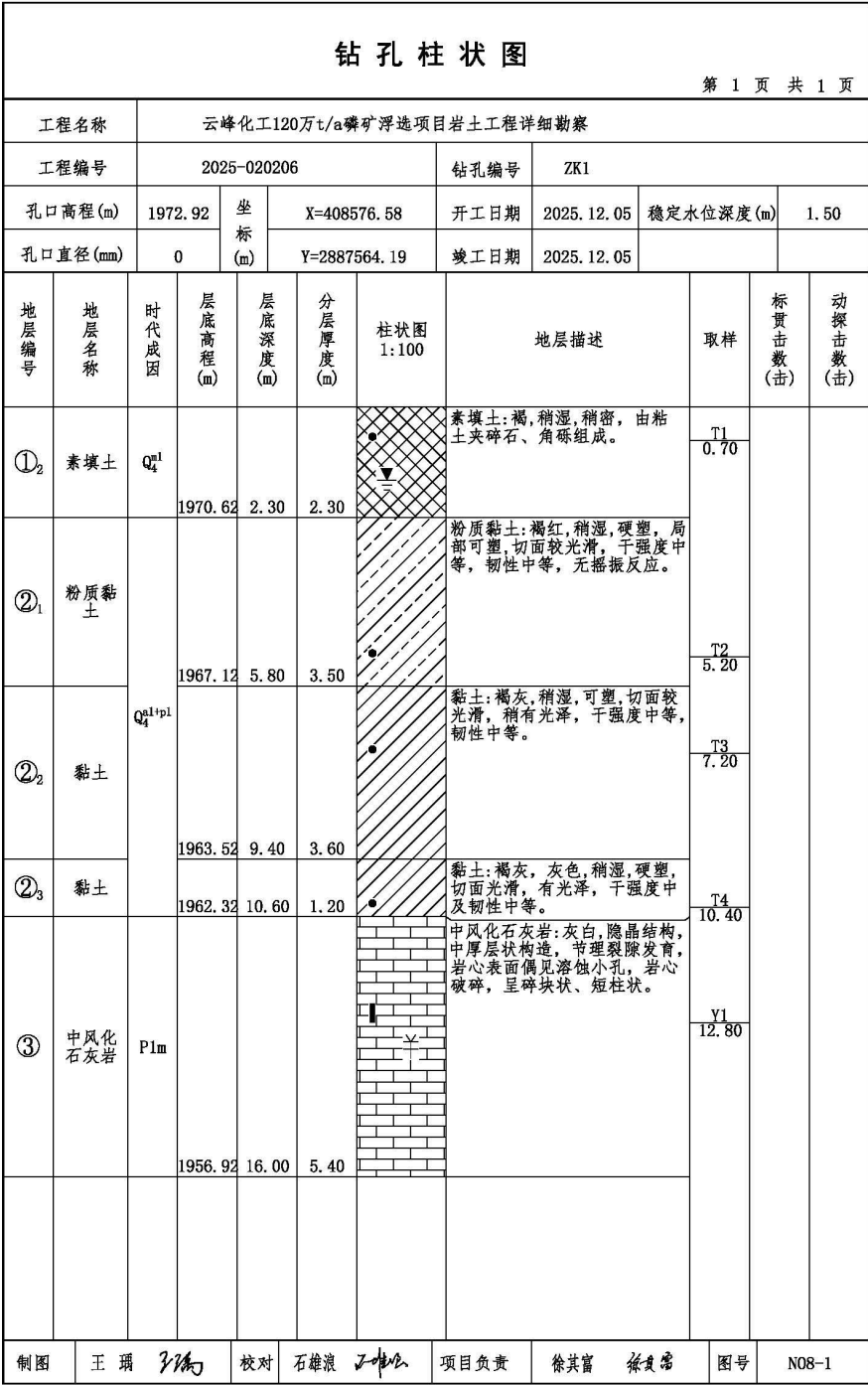
图 6.2.3-5 ZK1 柱状图
