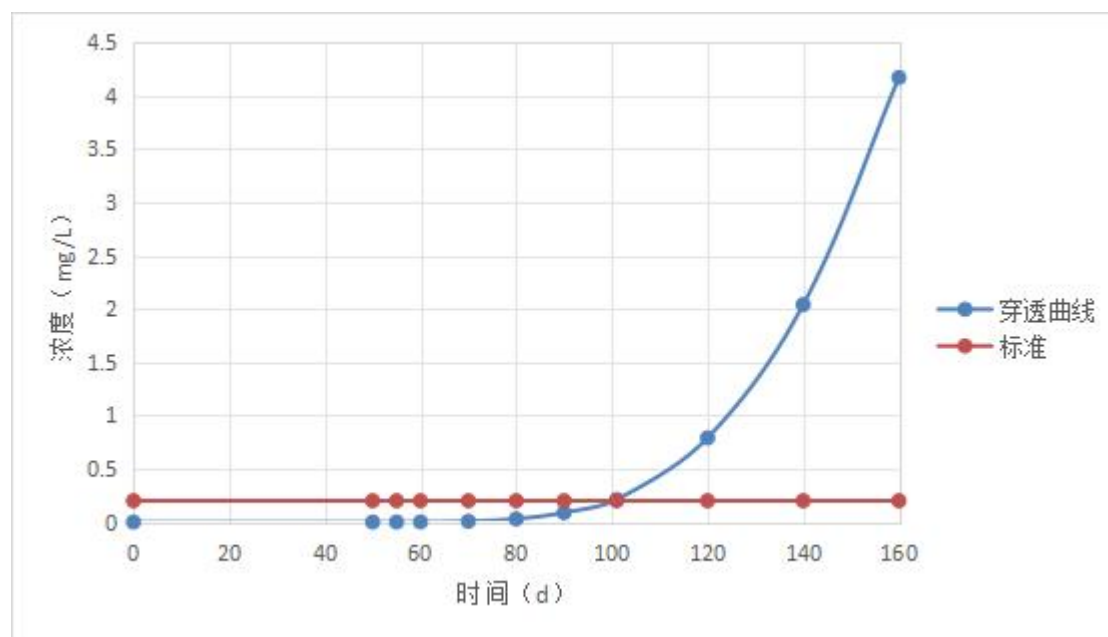
图 6.2.3-10 跟踪监测井中总磷浓度变化曲线图
