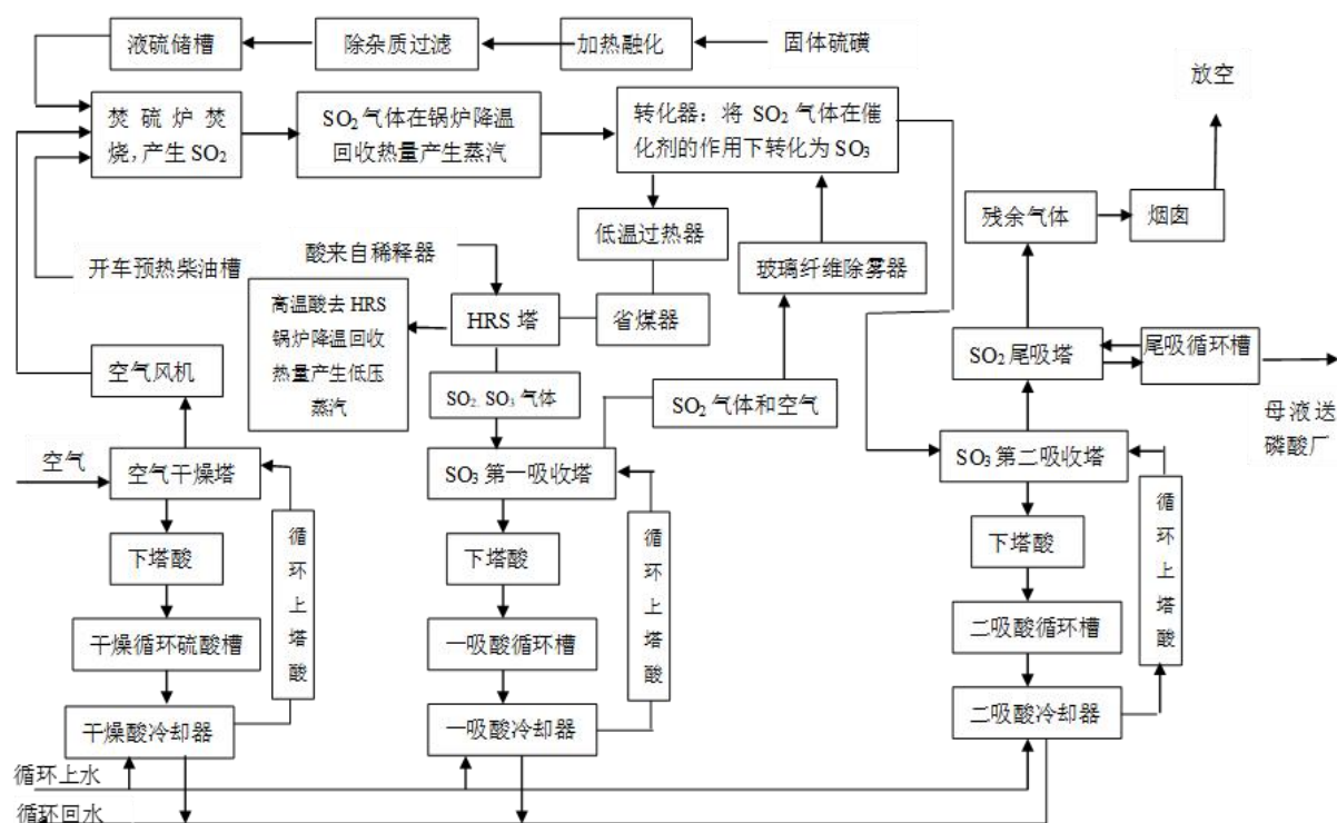
图 2.5.1-1 30 万吨 A 系列硫酸生产工艺流程图
