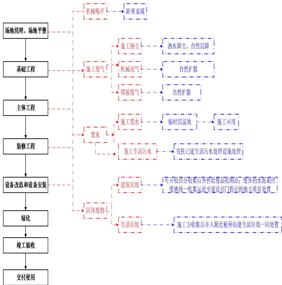
图 4.1.1-1 施工期工艺流程图及产污节点图
