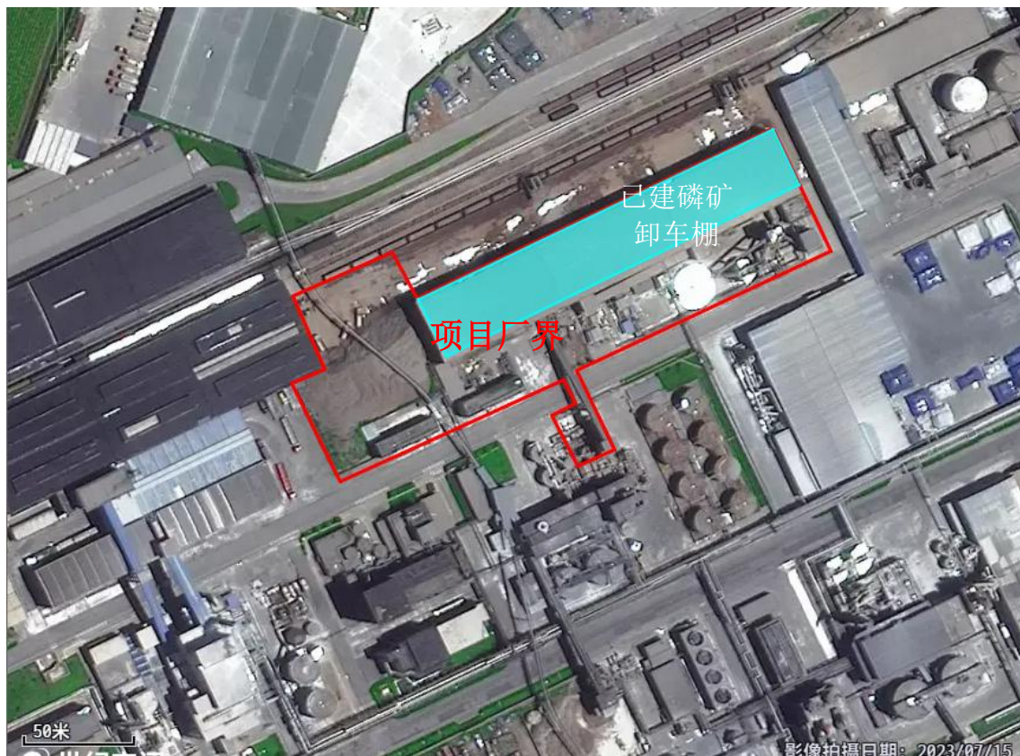
图 3.10.1-1 依托已建磷矿卸车棚现状和项目厂区位置关系图
