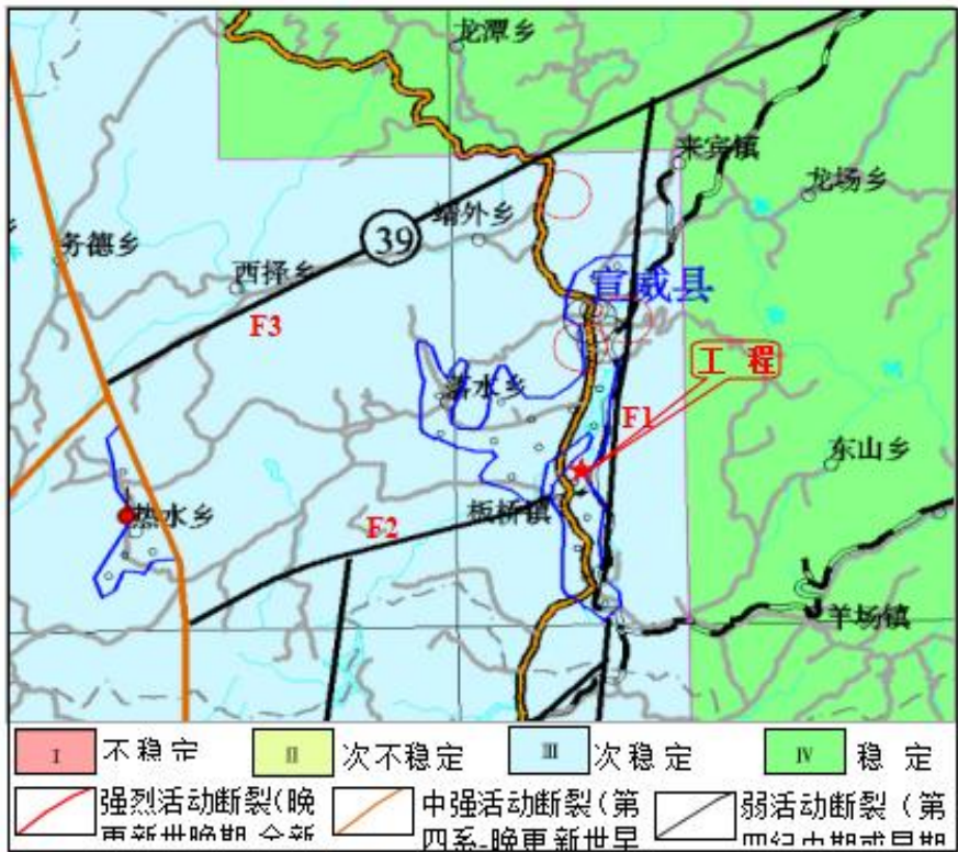
图 6.2.3-3 场地区域地质构造及地壳稳定性分区图
