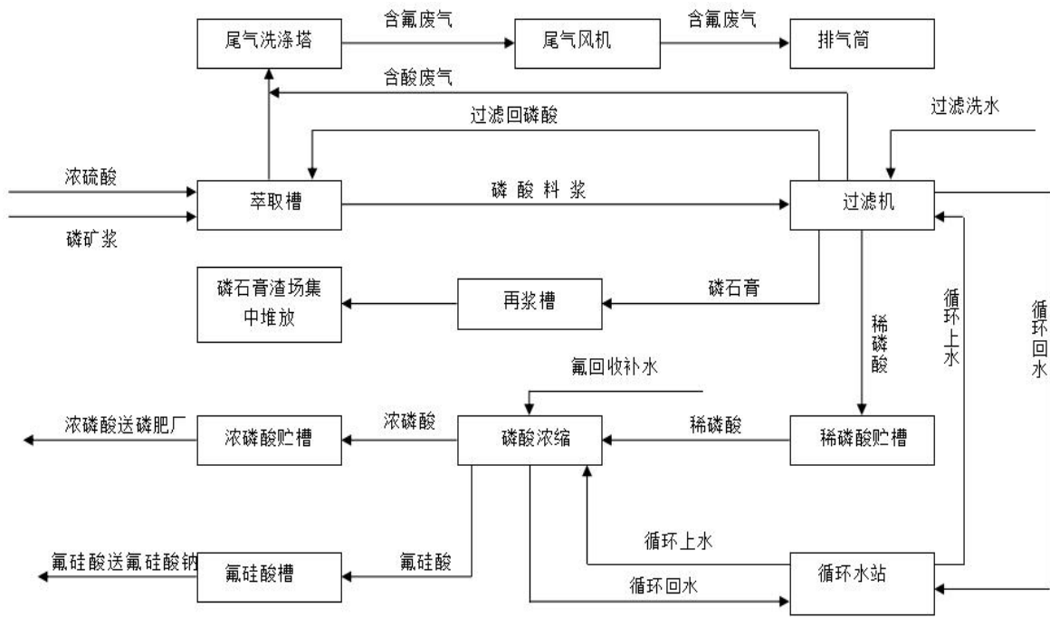
图 2.5.2-3 磷酸装置生产工艺流程图
