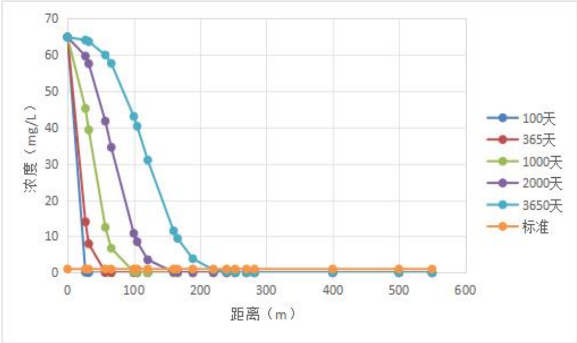
图 6.2.3-7 项目回水池泄漏 Mn 浓度扩散曲线图
