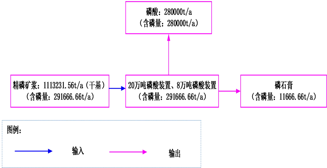
图 2.7-1 云南云天化云峰化工有限公司全厂 P_2O_5 平衡图
