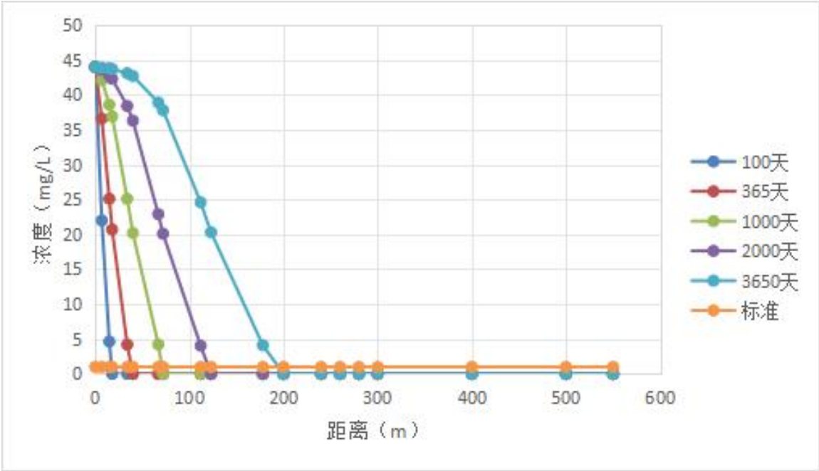
图 6.2.3-9 选厂回水池泄漏 CODcr 浓度扩散曲线图
