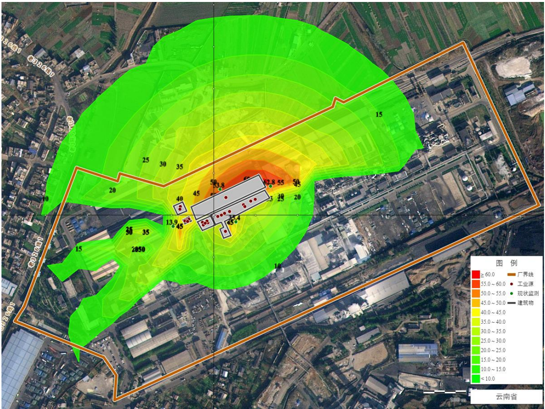
图 6.2.4-1 项目等声值线图
