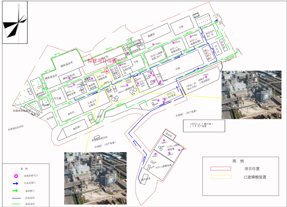
图 2.2-3 项目与磷酸生产装置位置关系示意图
