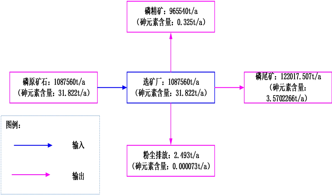
图 4.3.2-3 项目砷元素平衡图（干基）
