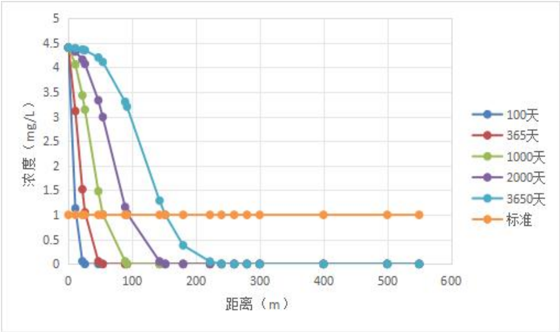
图 6.2.3-8 选厂回水池泄漏氟化物浓度扩散曲线图
