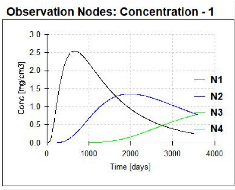
图6.2.6-2 不同深度污染物CODcr的浓度随时间变化曲线图
