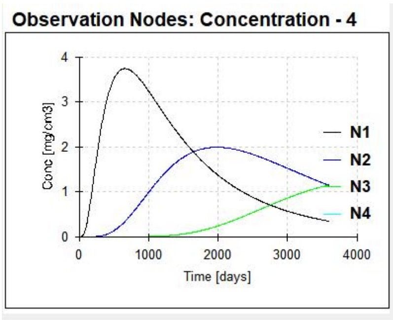
图6.2.6-3 不同深度污染物锰的浓度随时间变化曲线图
