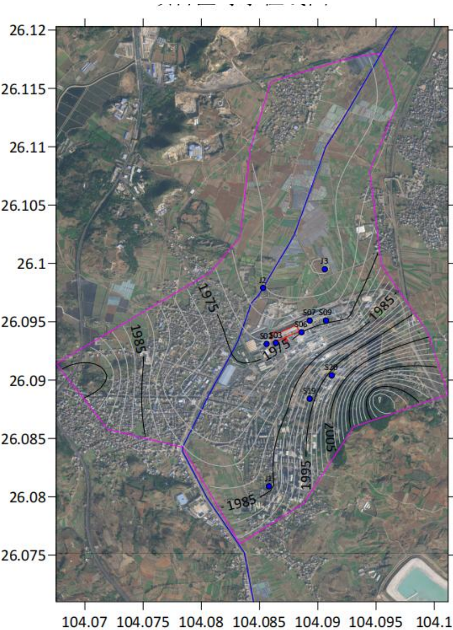
图 6.2.3-2 评价区等水位线图
