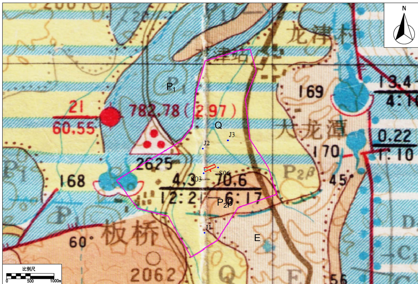
图 6.2.3-1 区域水文地质图
