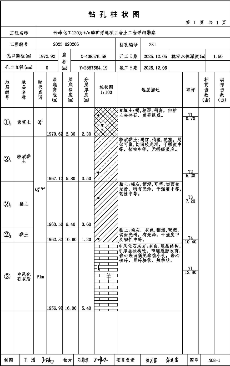
图 6.2.3-7 ZK9 柱状图
