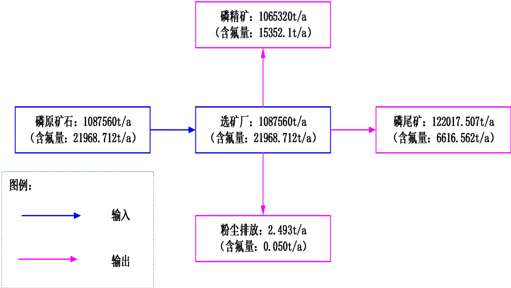
图 4.3.2-3 项目氟平衡图（干基）
