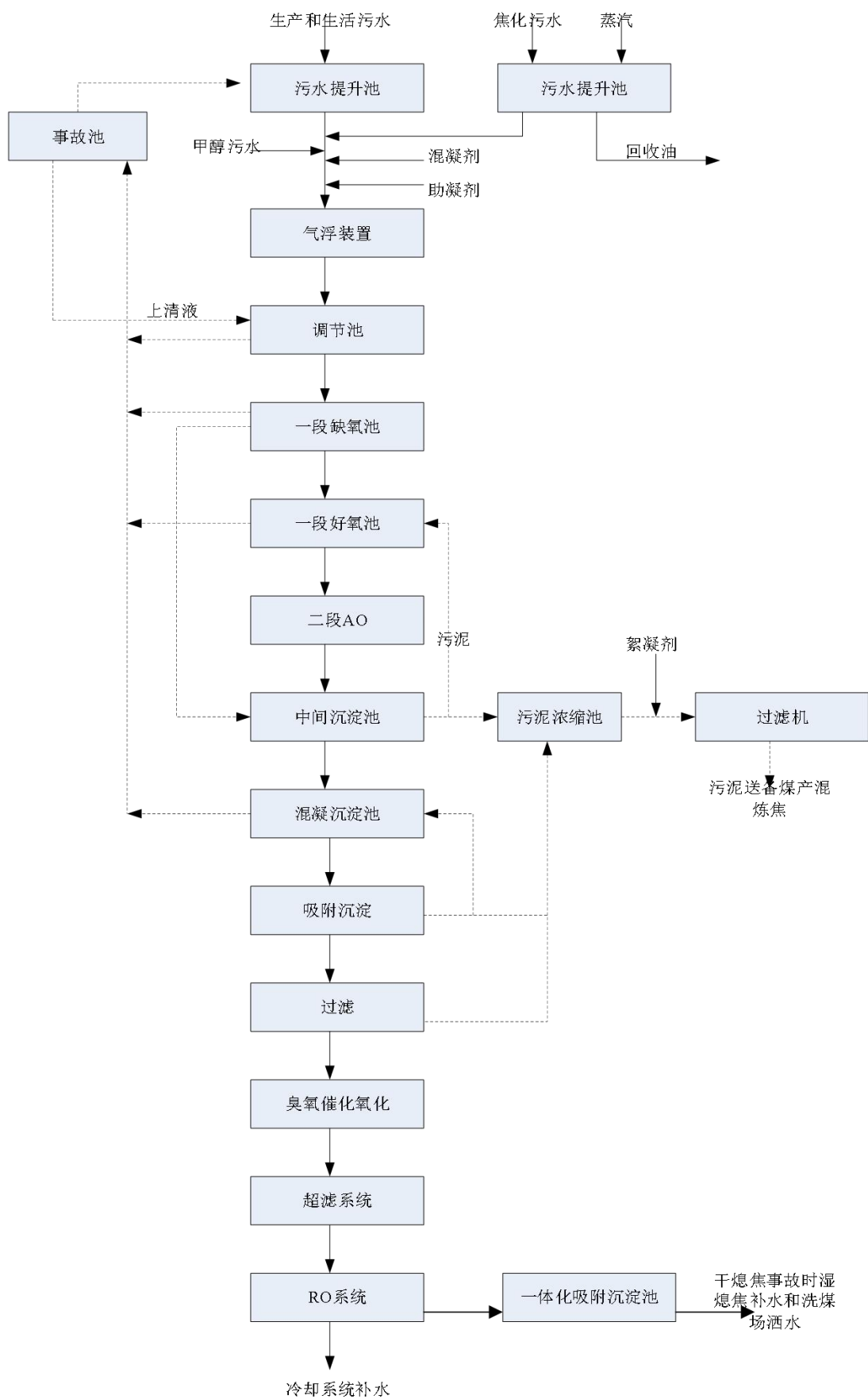
图 6.2-2 改干熄焦后生化处理站工艺流程及产污环节图
