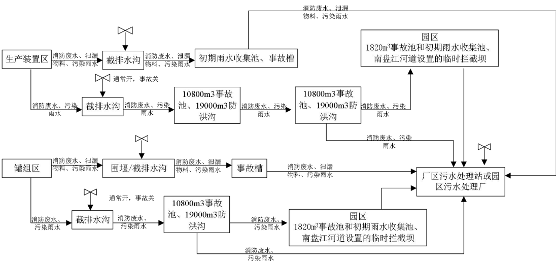
图12.6-85 项目一级、二级和三级事故废水收集处理系统图
