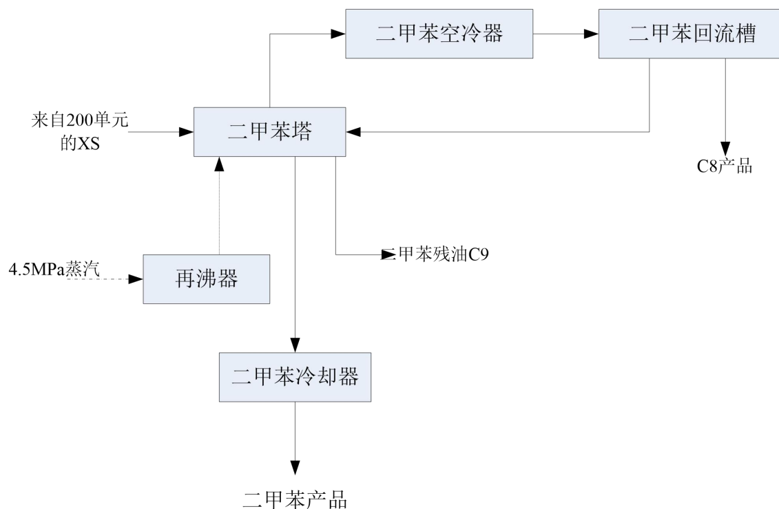
图2.2-4 400单元工艺流程图
