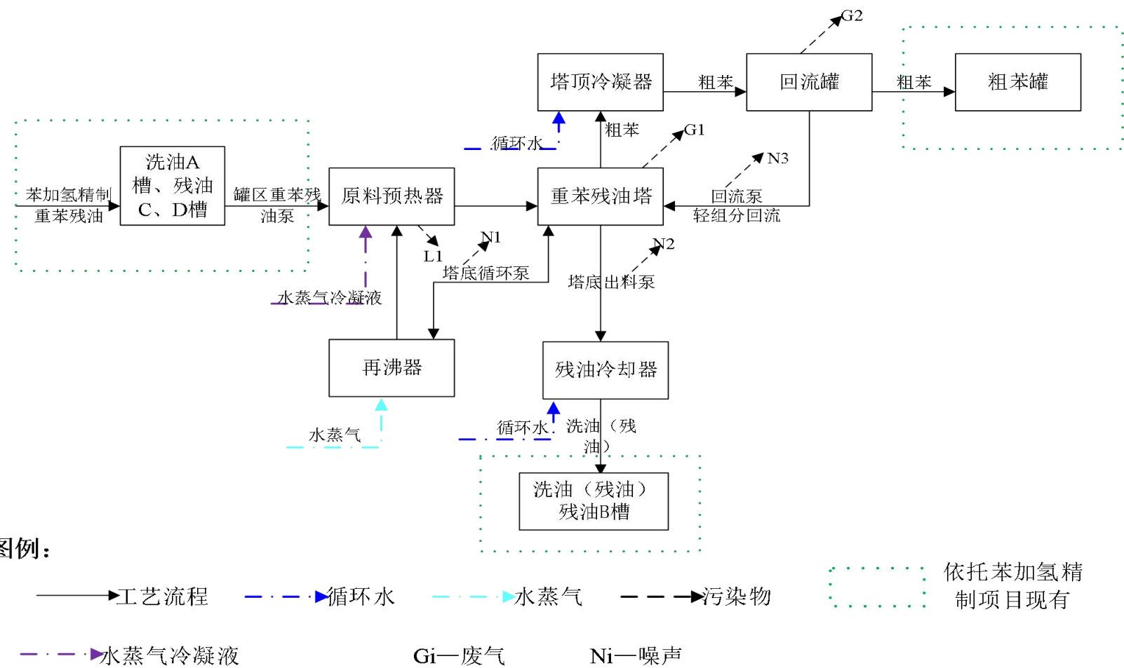
图3.2-1 项目工艺流程及产物环节图
