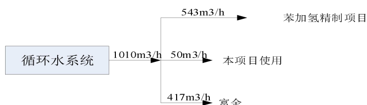
图 2.10-1 循环水系统循环用水平衡图
