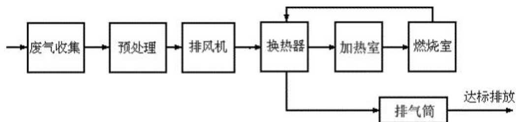
图 2.2-7 焚烧装置示意图
