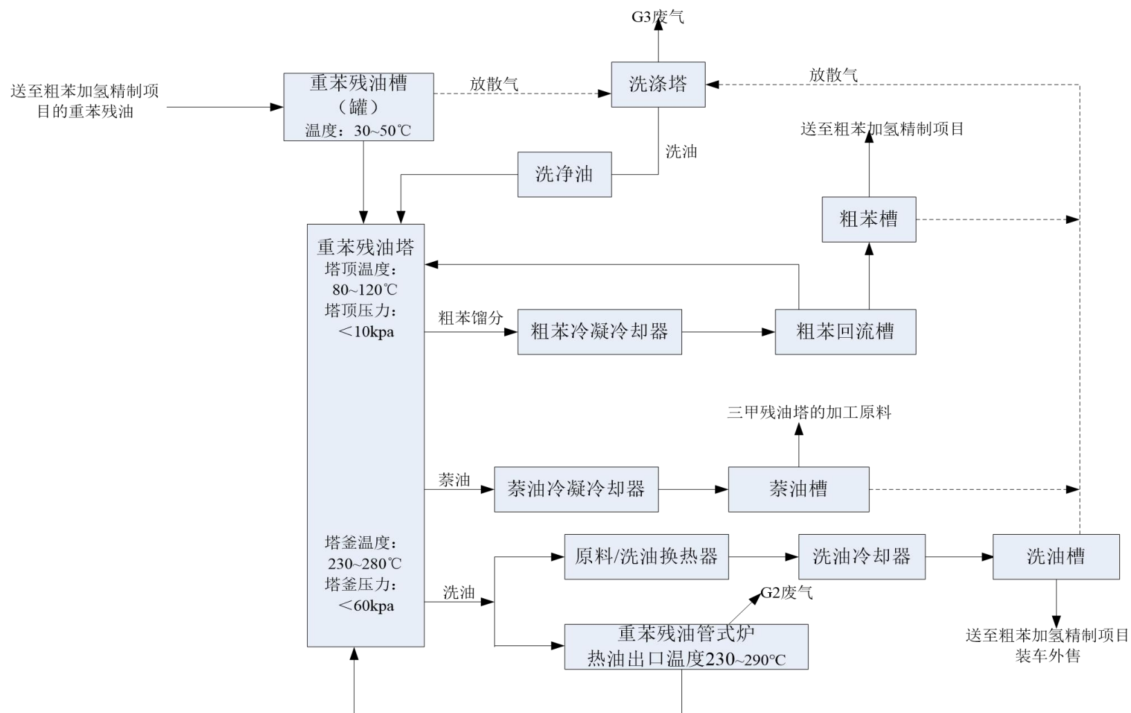
图2.2-11 重苯残油加工系统工艺流程图
