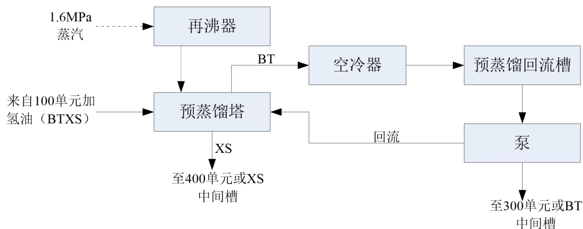
图2.2-2 200单元工艺流程图
