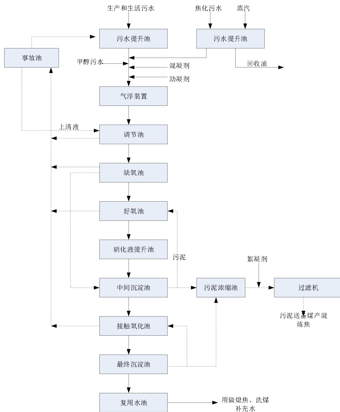
图 6.2-1 现状生化处理站工艺流程及产污环节图
