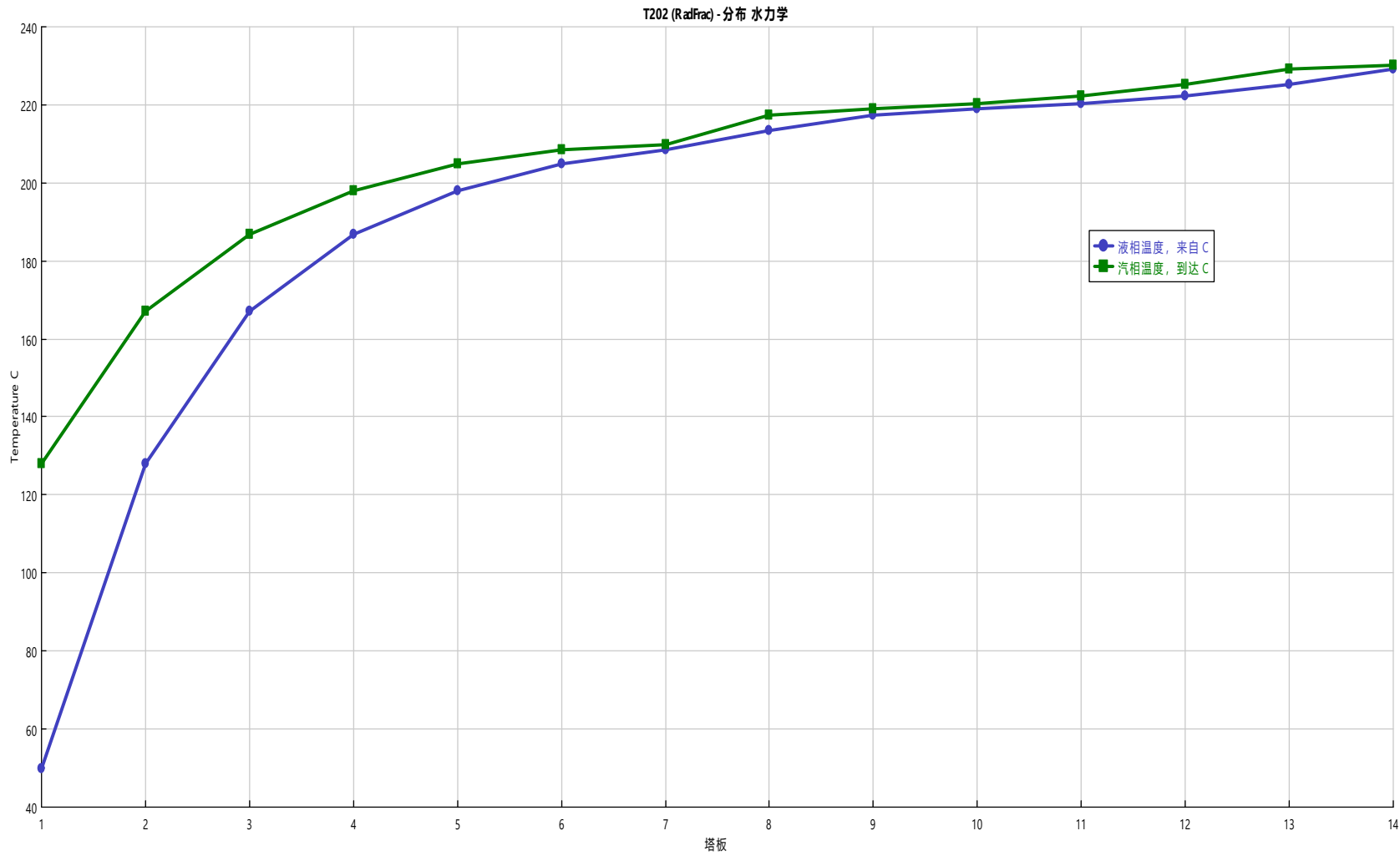
图 3.2-2 塔内温度变化曲线图
