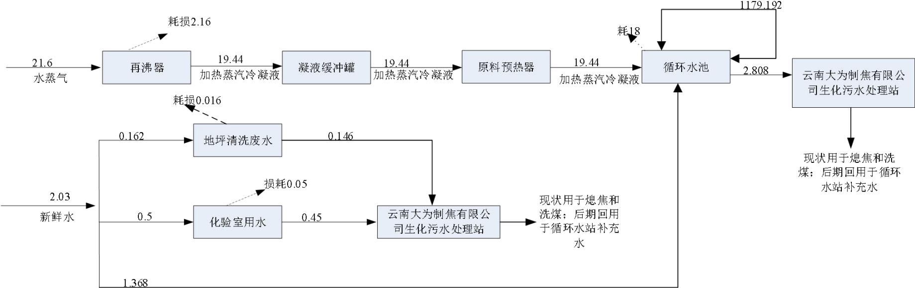
图 3.2-4 项目水量平衡图 单位：m³/d
