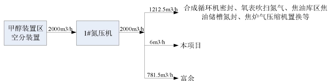
图2.10-3 氮气生产工艺流程及氮气供给平衡图
