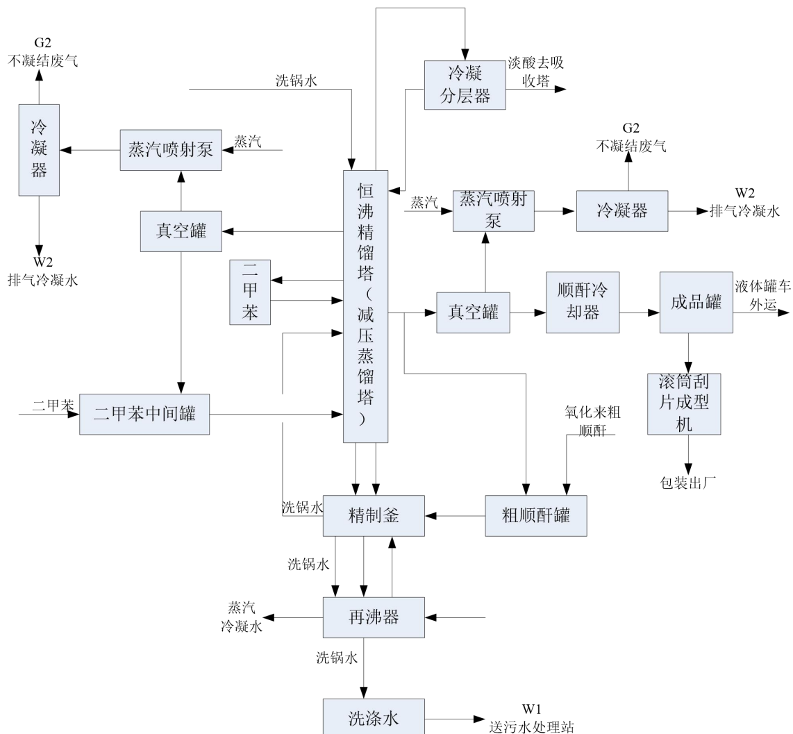
图2.2-6 顺酐精制排污节点工艺流程示意图
