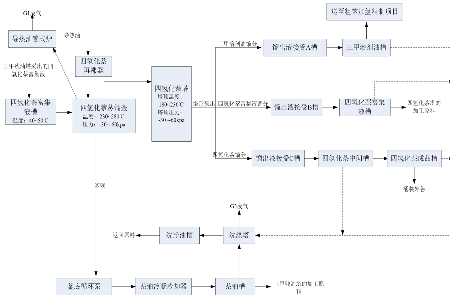
图2.2-10 四氢化萘加工系统工艺流程图
