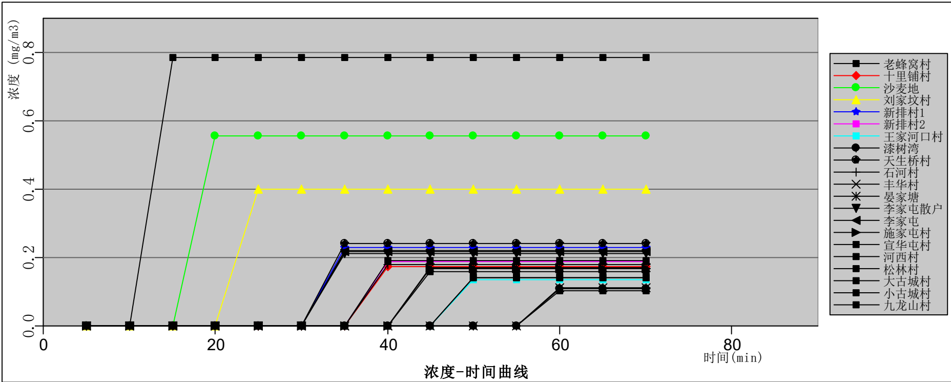
图12.6-7 回流罐泄漏最不利气象条件各敏感点处甲苯浓度随时间变化曲线图
