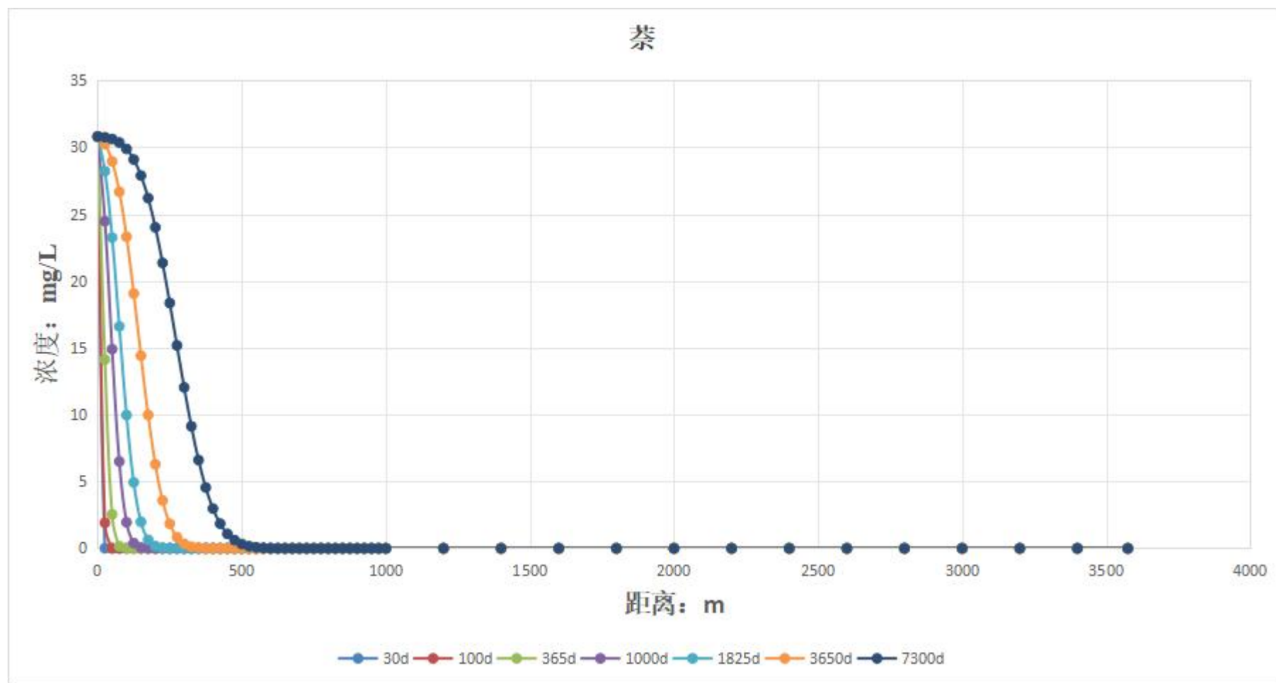
图7.9-4 管道渗漏后萘浓度变化图（标准值为0.1mg/L）
