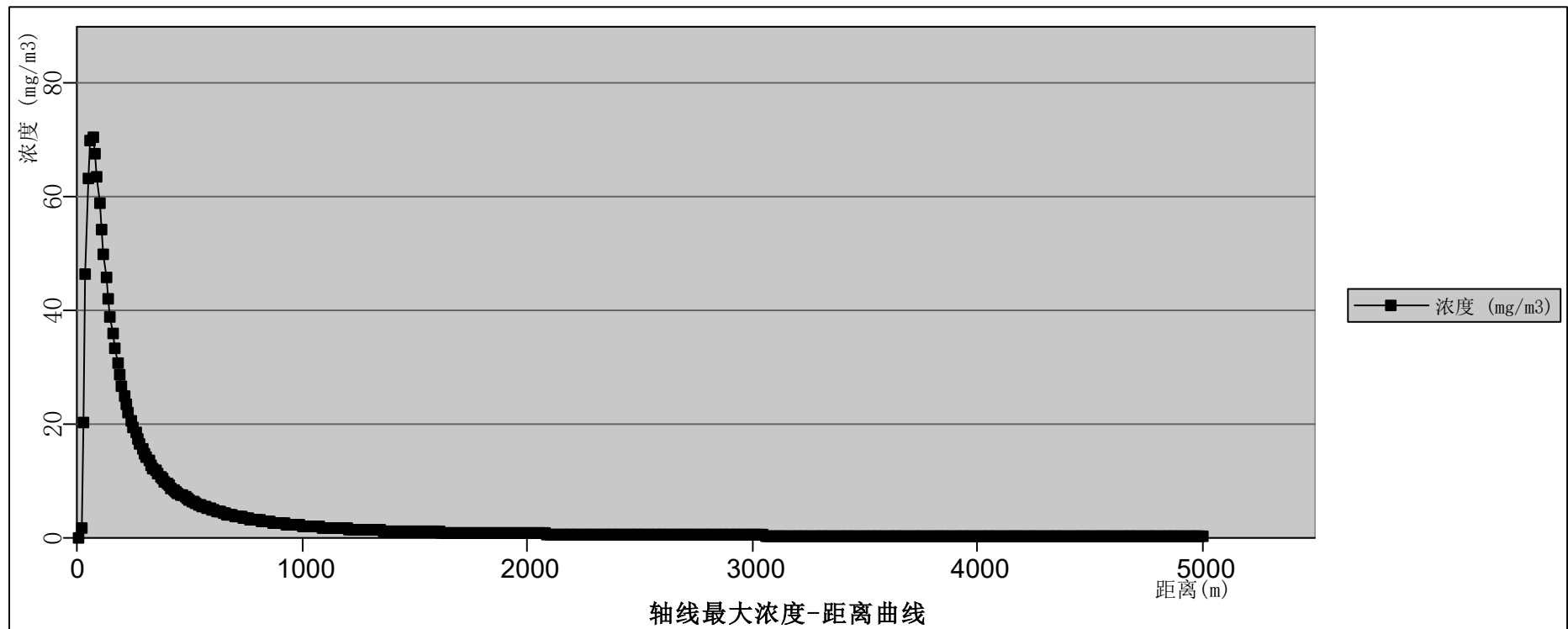
图 12.6-69 粗苯罐泄漏苯扩散轴线最大浓度——距离曲线（最不利气象条件下）
