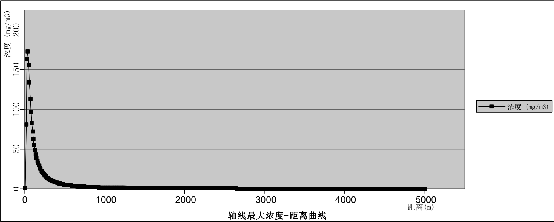
图 12.6-10 回流罐泄漏二甲苯扩散轴线最大浓度——距离曲线（最常见气象条件）
