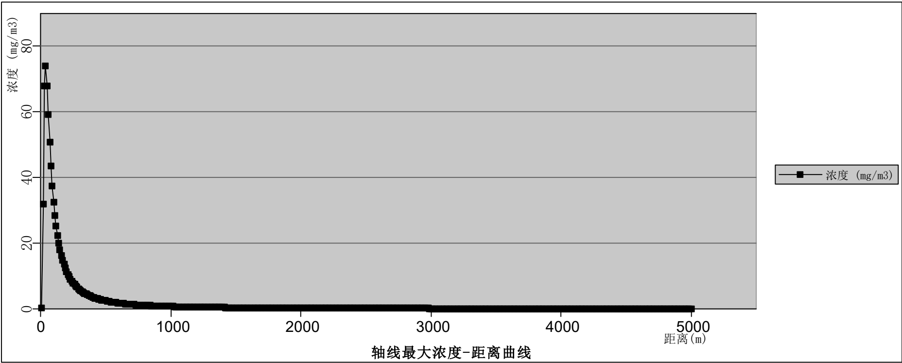
图 12.6-22 回流罐泄漏环己烷扩散轴线最大浓度——距离曲线（最常见气象条件）
