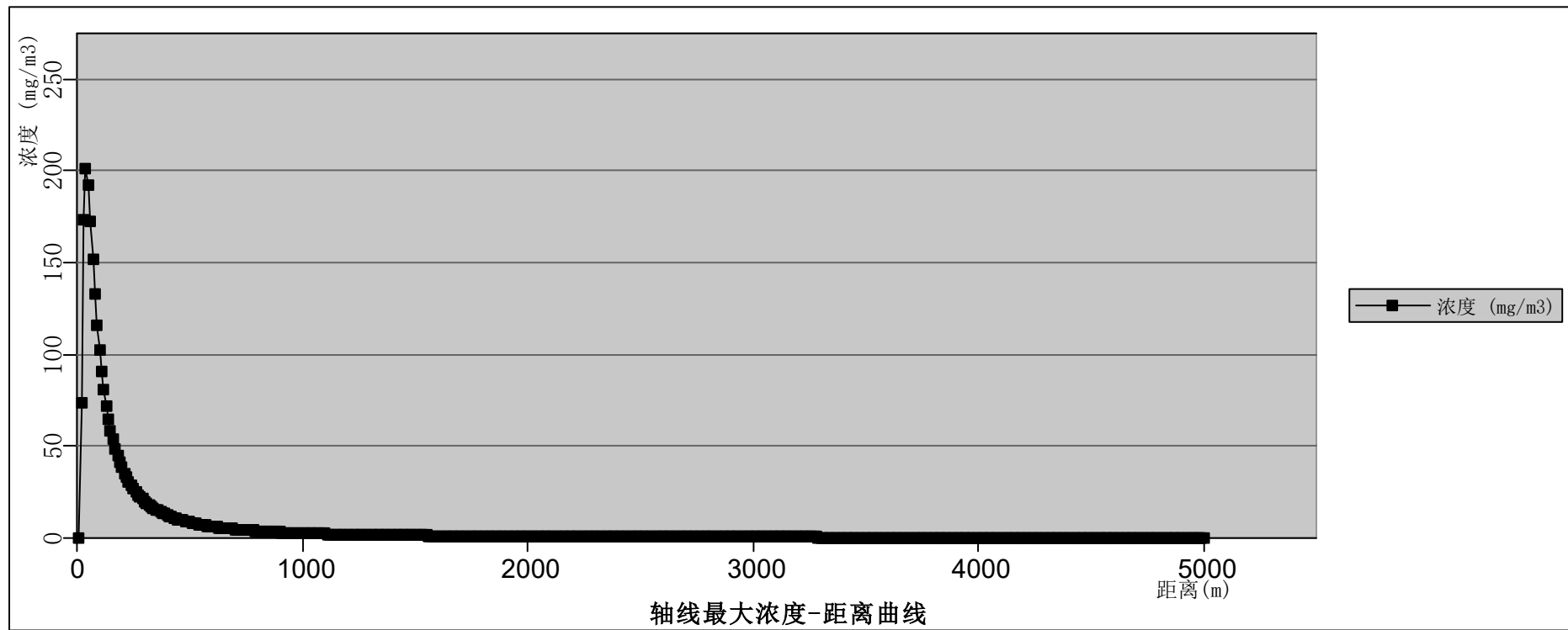
图 12.6-46 粗苯罐泄漏甲苯扩散轴线最大浓度——距离曲线（最常见气象条件）
