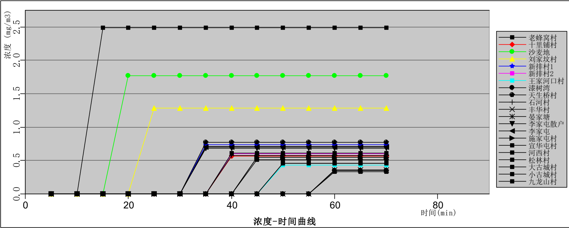
图12.6-57 粗苯罐泄漏最不利气象条件各敏感点处乙苯浓度随时间变化曲线图
