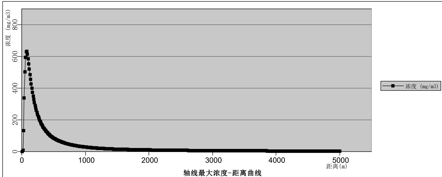
图 12.6-41 粗苯罐泄漏苯扩散轴线最大浓度——距离曲线（最不利气象条件下）
