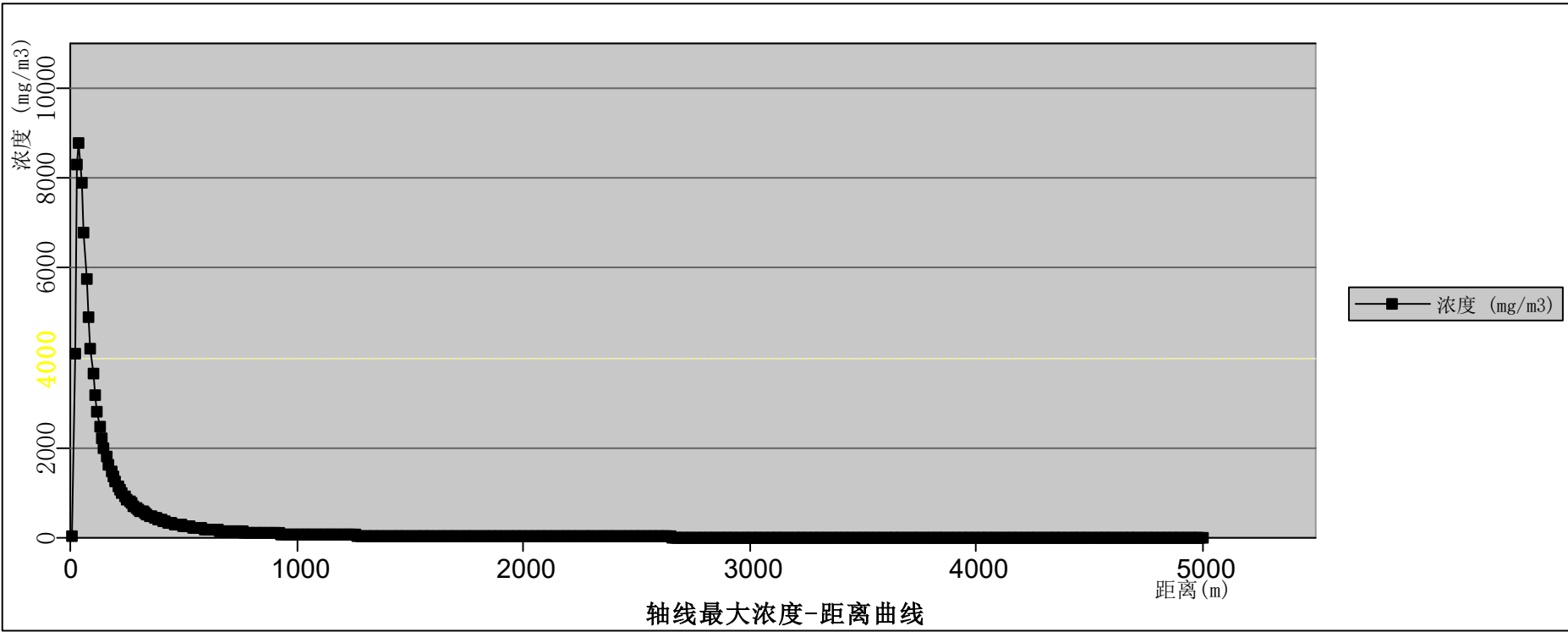
图 12.6-50 粗苯罐泄漏二甲苯扩散轴线最大浓度——距离曲线（最常见气象条件）
