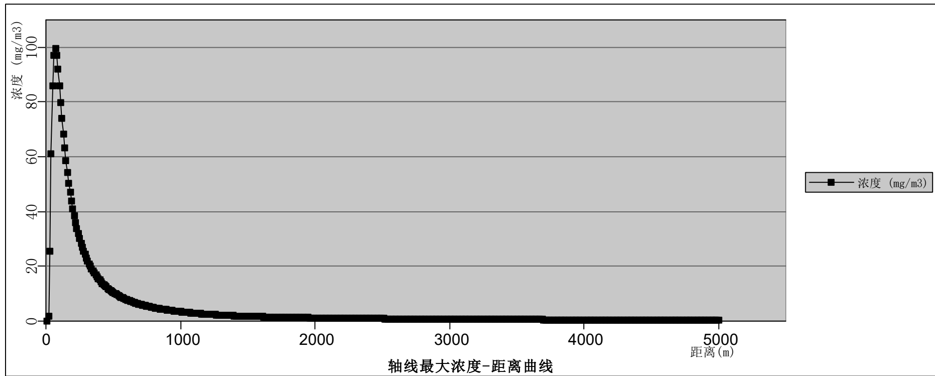
图 12.6-21 回流罐泄漏环己烷扩散轴线最大浓度——距离曲线（最不利气象条件下）
