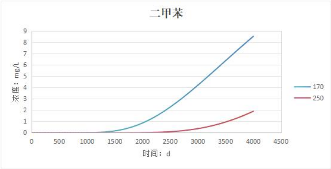
图 7.9-7 固定位置二甲苯（监测井和最近厂界处）污染物浓度穿透曲线图
