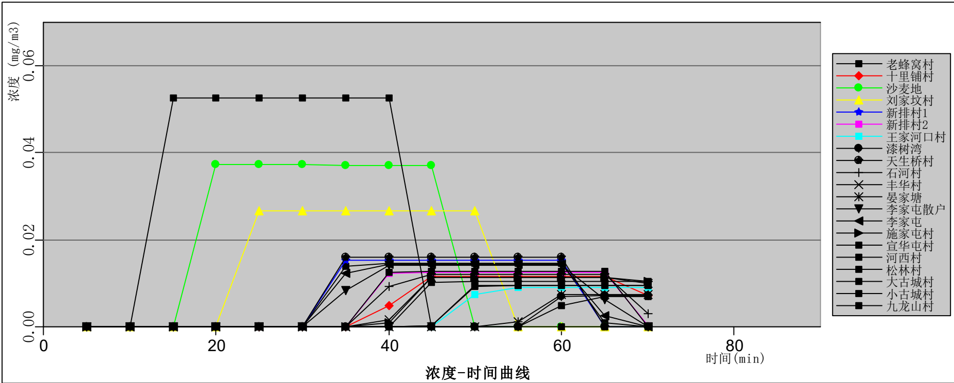
图12.6-27 回流罐泄漏最不利气象条件各敏感点处苯浓度随时间变化曲线图
