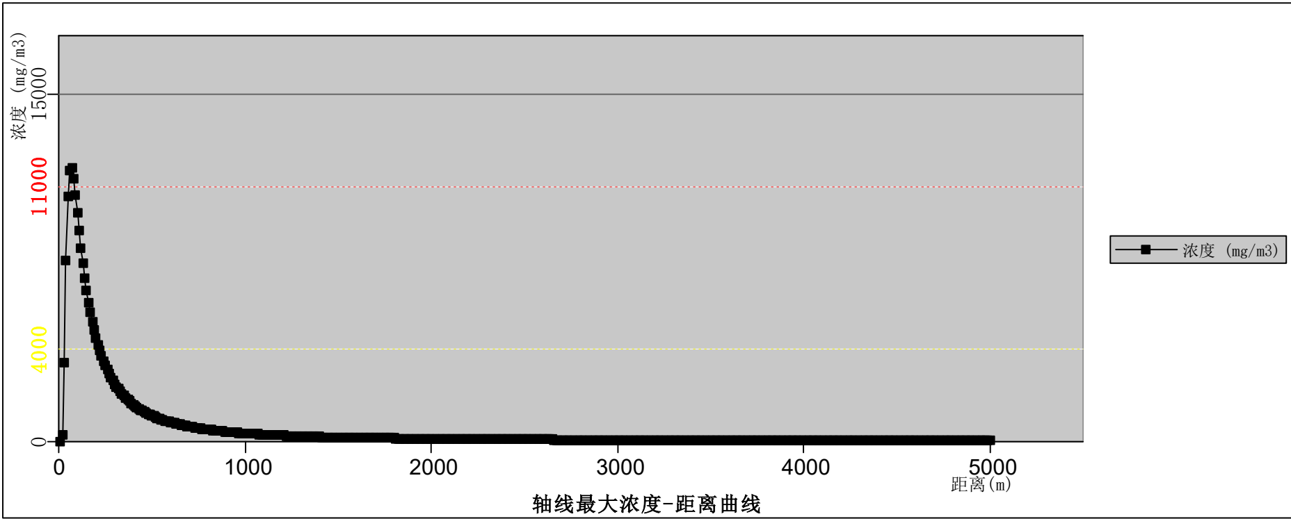
图 12.6-49 粗苯罐泄漏二甲苯扩散轴线最大浓度——距离曲线（最不利气象条件下）
