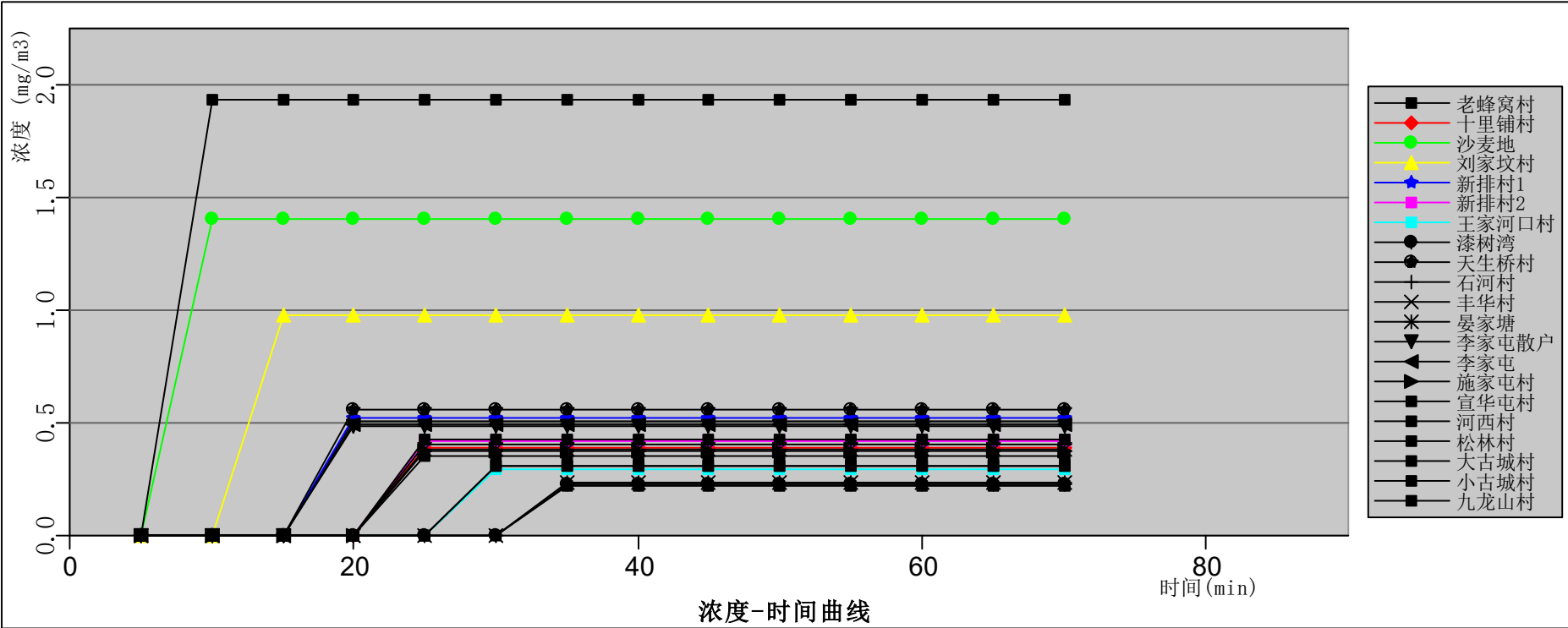
图12.6-48 粗苯罐泄漏最常见气象条件各敏感点处甲苯浓度随时间变化曲线图
