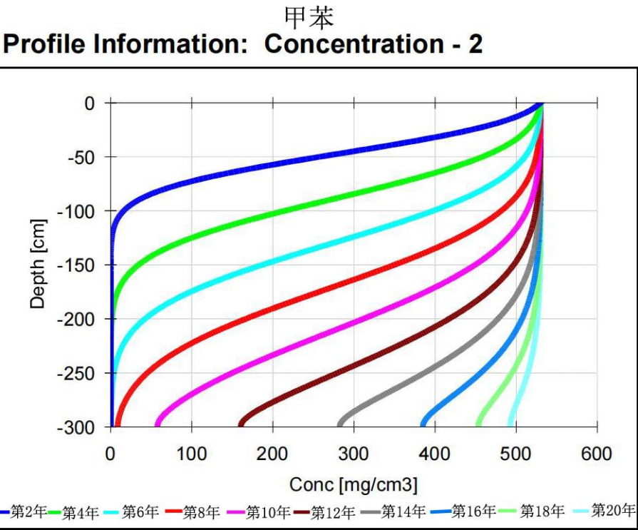
图 10.3-4 土壤不同年份不同深度甲苯浓度变化曲线
