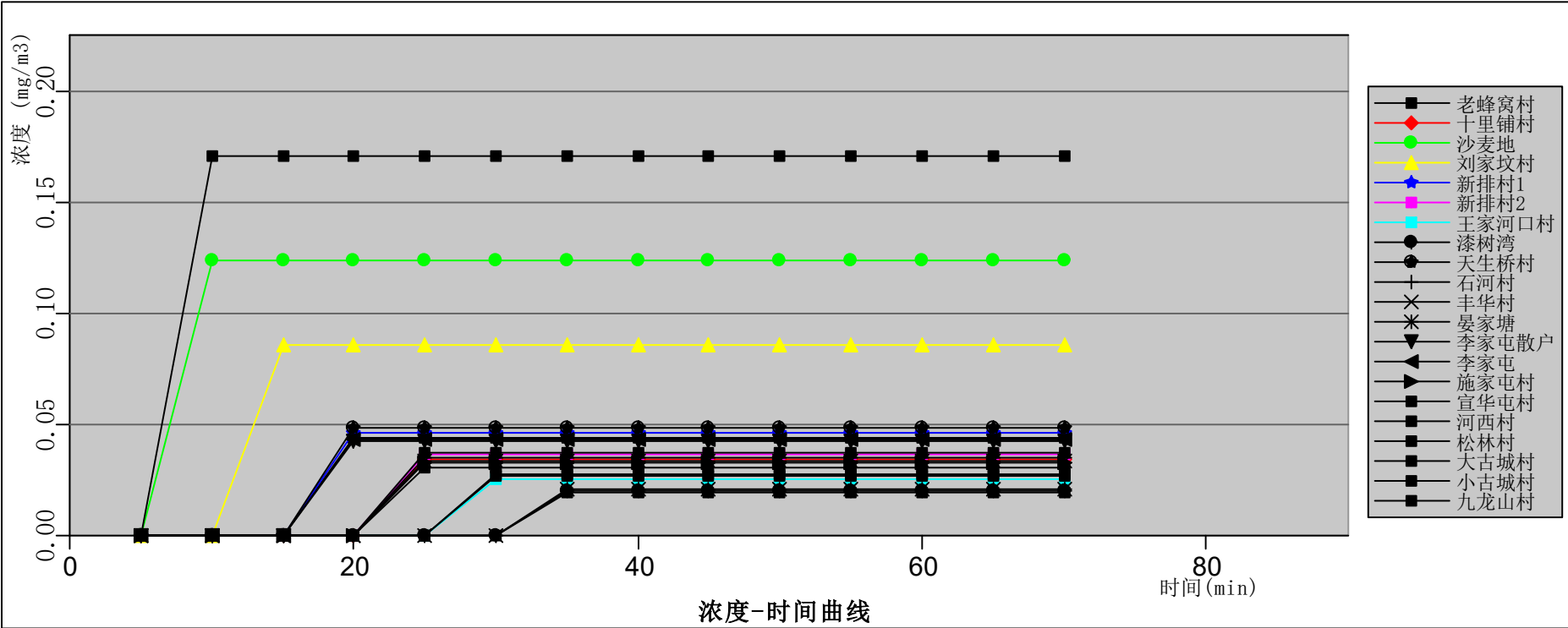
图12.6-8 回流罐泄漏最常见气象条件各敏感点处甲苯浓度随时间变化曲线图
