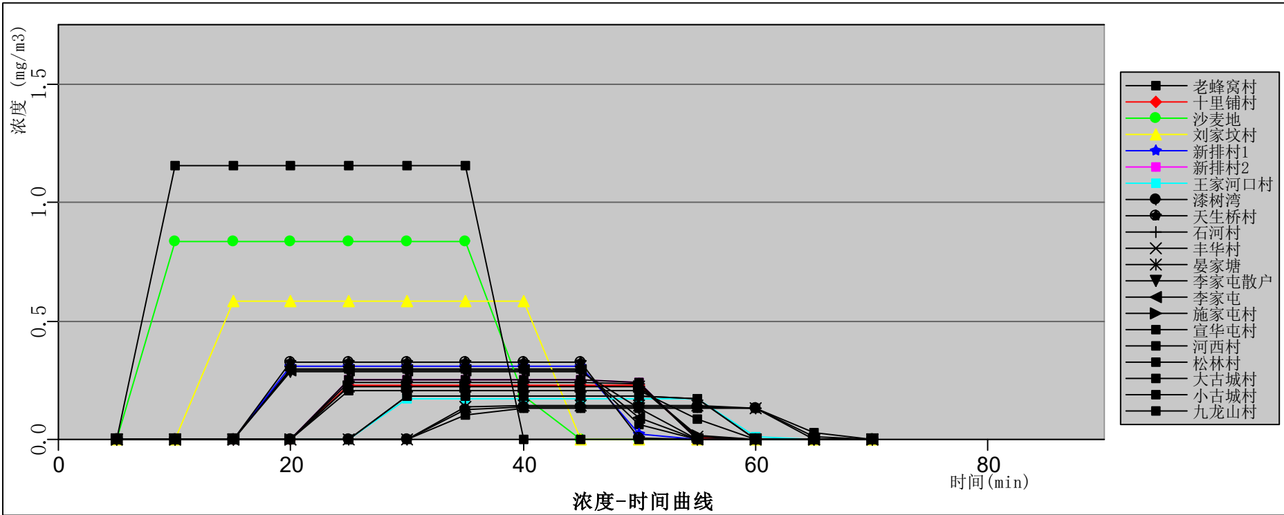
图12.6-12 回流罐泄漏最常见气象条件各敏感点处二甲苯浓度随时间变化曲线图
