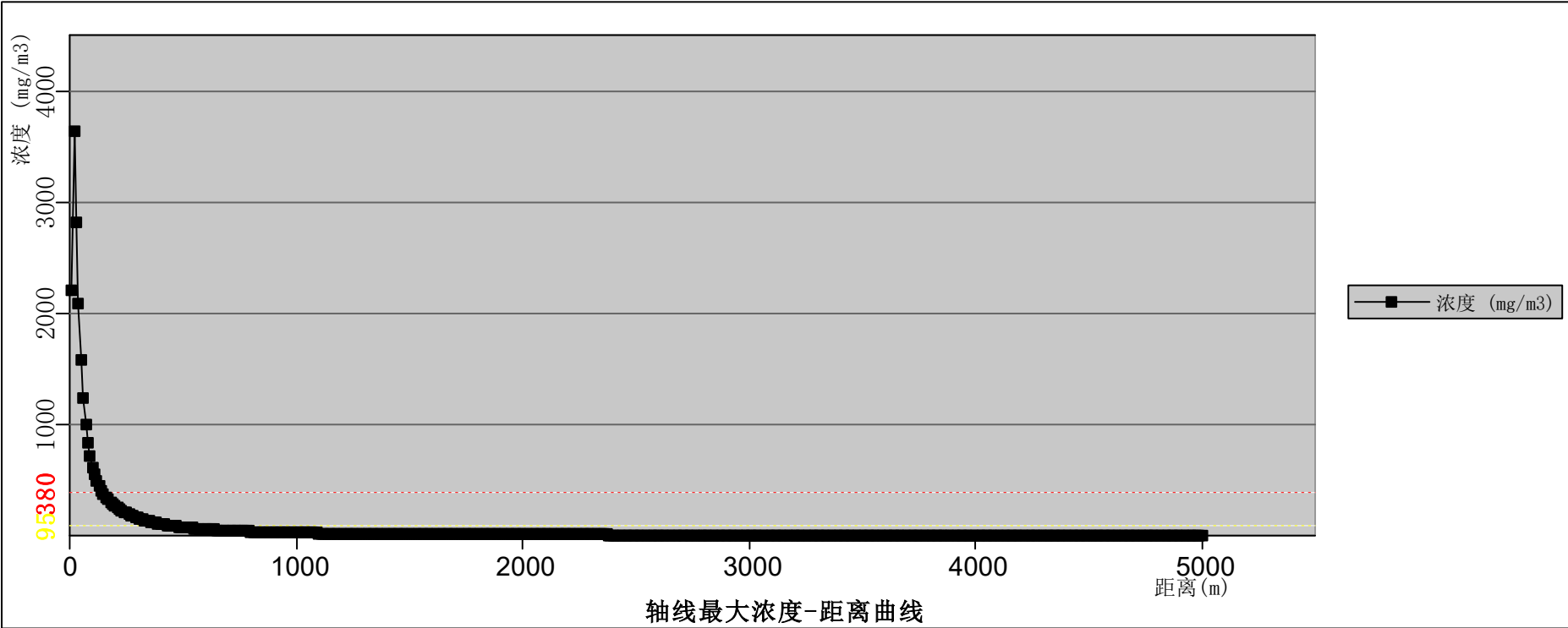
图 12.6-29 回流罐火灾爆炸 CO 扩散轴线最大浓度——距离曲线（最不利气象条件下）
