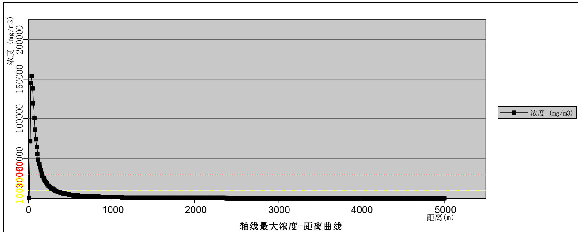
图 12.6-60 粗苯罐泄漏正己烷扩散轴线最大浓度——距离曲线（最常见气象条件）
