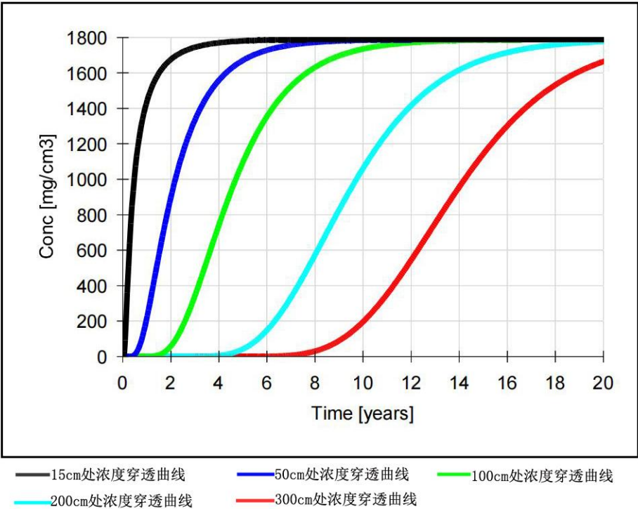
图 10.3-1 土壤不同深度处苯浓度变化曲线
