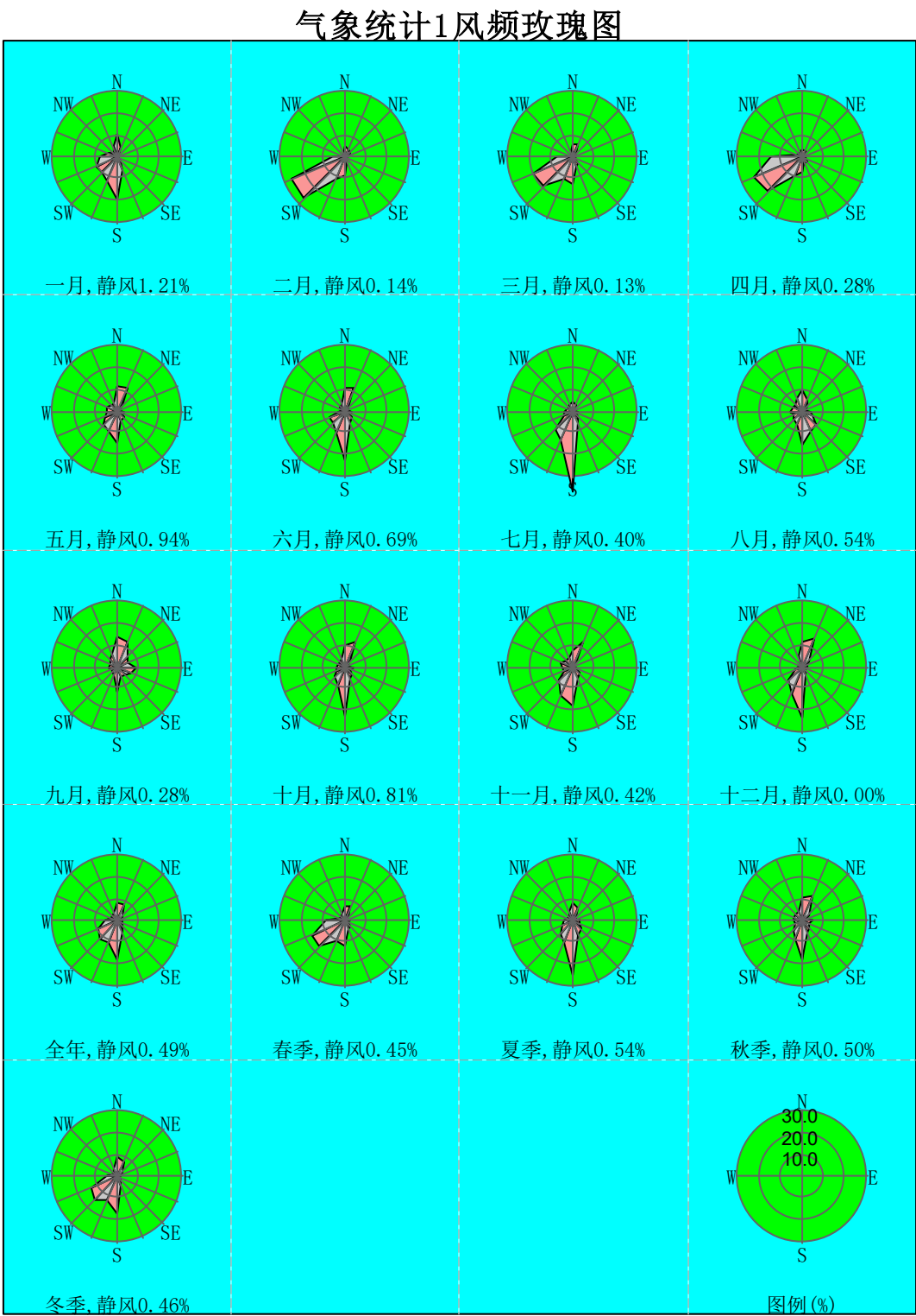
图 5.2-1 沾益区 2024 年风向频率月、季、年均玫瑰图
