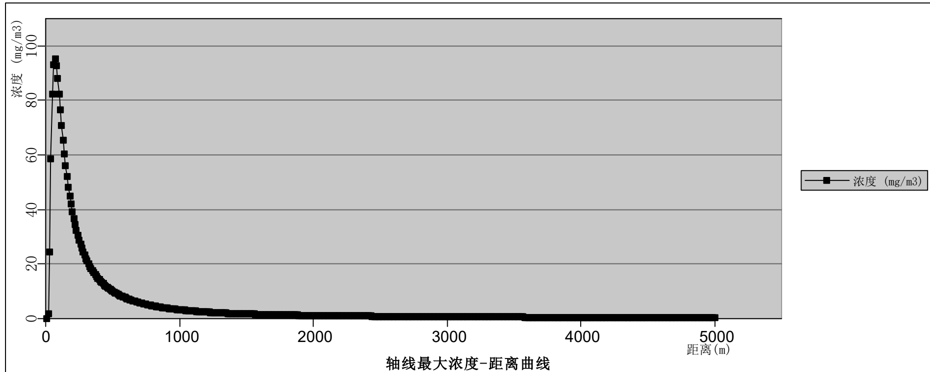
图 12.6-1 回流罐泄漏苯扩散轴线最大浓度—距离曲线（最不利气象条件下）
