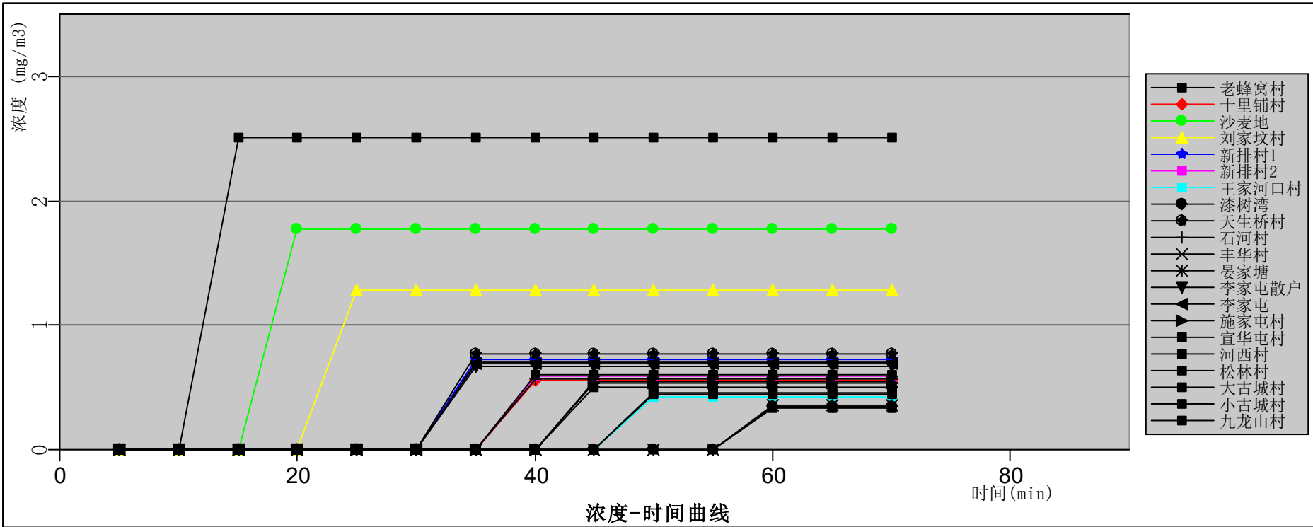
图12.6-23 回流罐泄漏最不利气象条件各敏感点处环己烷浓度随时间变化曲线图
