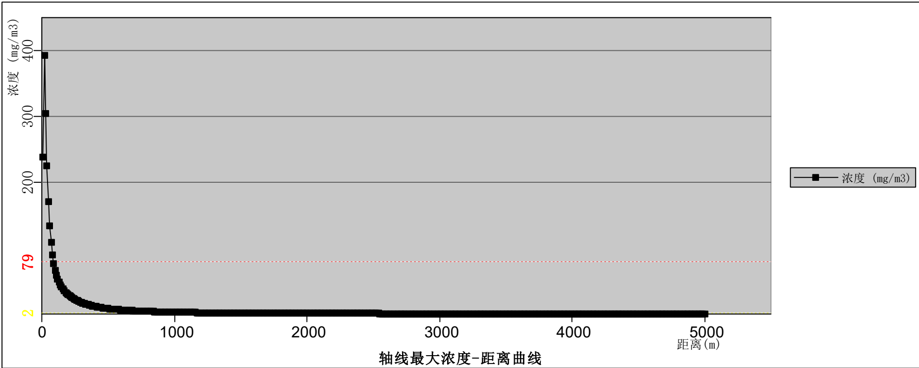
图 12.6-35 回流罐火灾爆炸 SO 2 扩散轴线最大浓度——距离曲线（最不利气象条件下）
