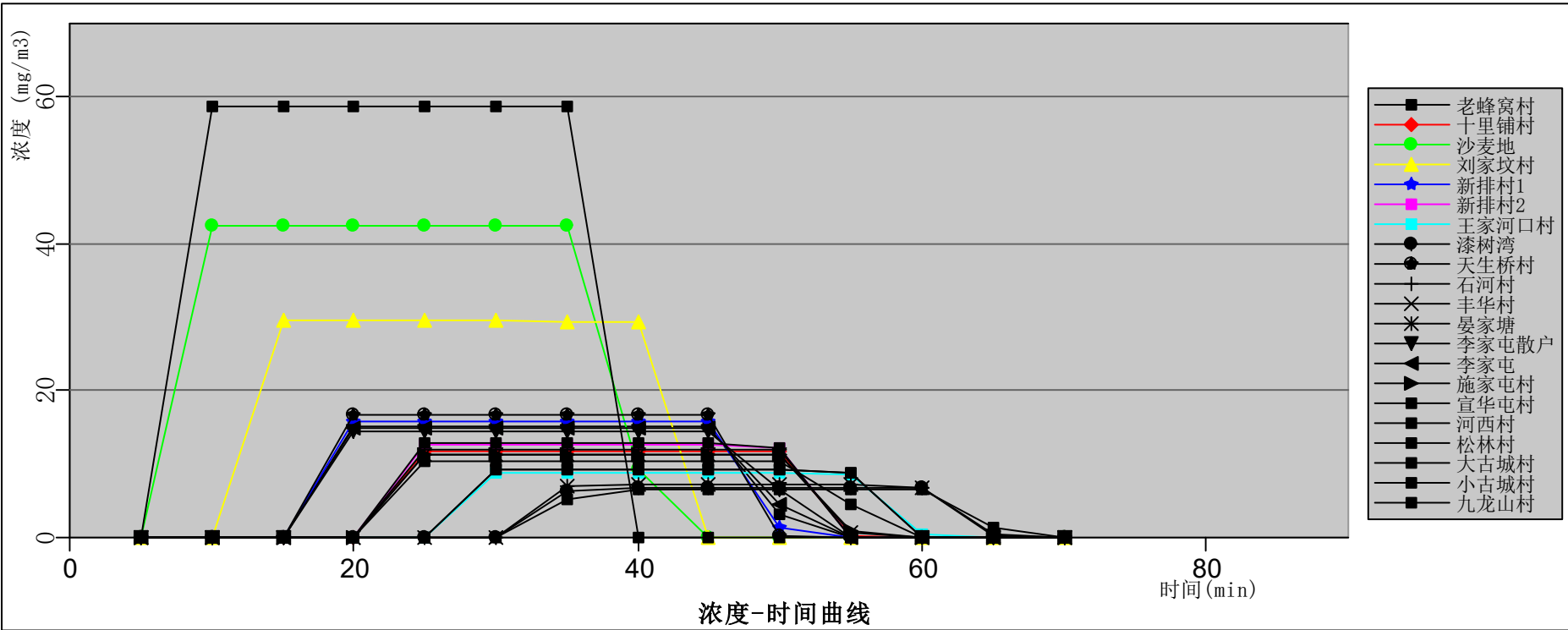
图12.6-54 粗苯罐泄漏最常见气象条件各敏感点处二甲苯浓度随时间变化曲线图
