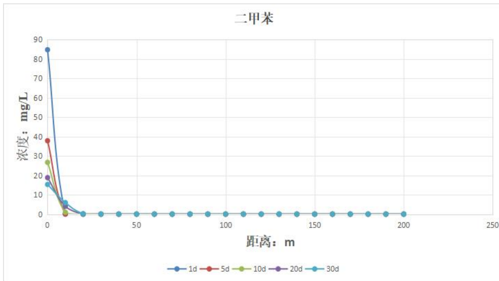
图12.6-92 回流罐泄漏甲苯下渗后浓度变化图（标准值为0.5mg/L）
