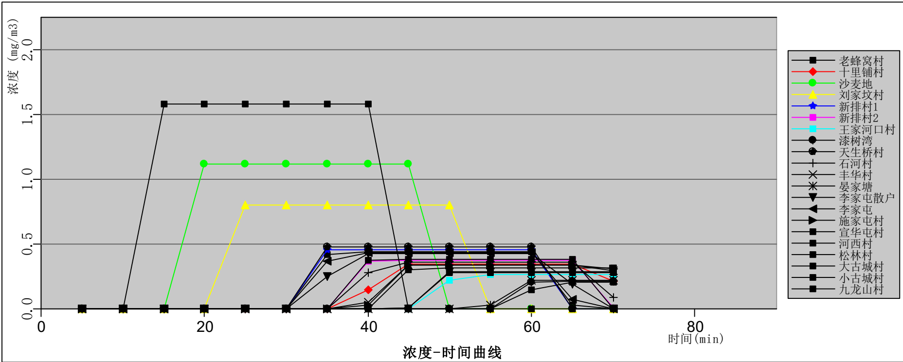
图12.6-71 粗苯罐泄漏最不利气象条件各敏感点处苯浓度随时间变化曲线图
