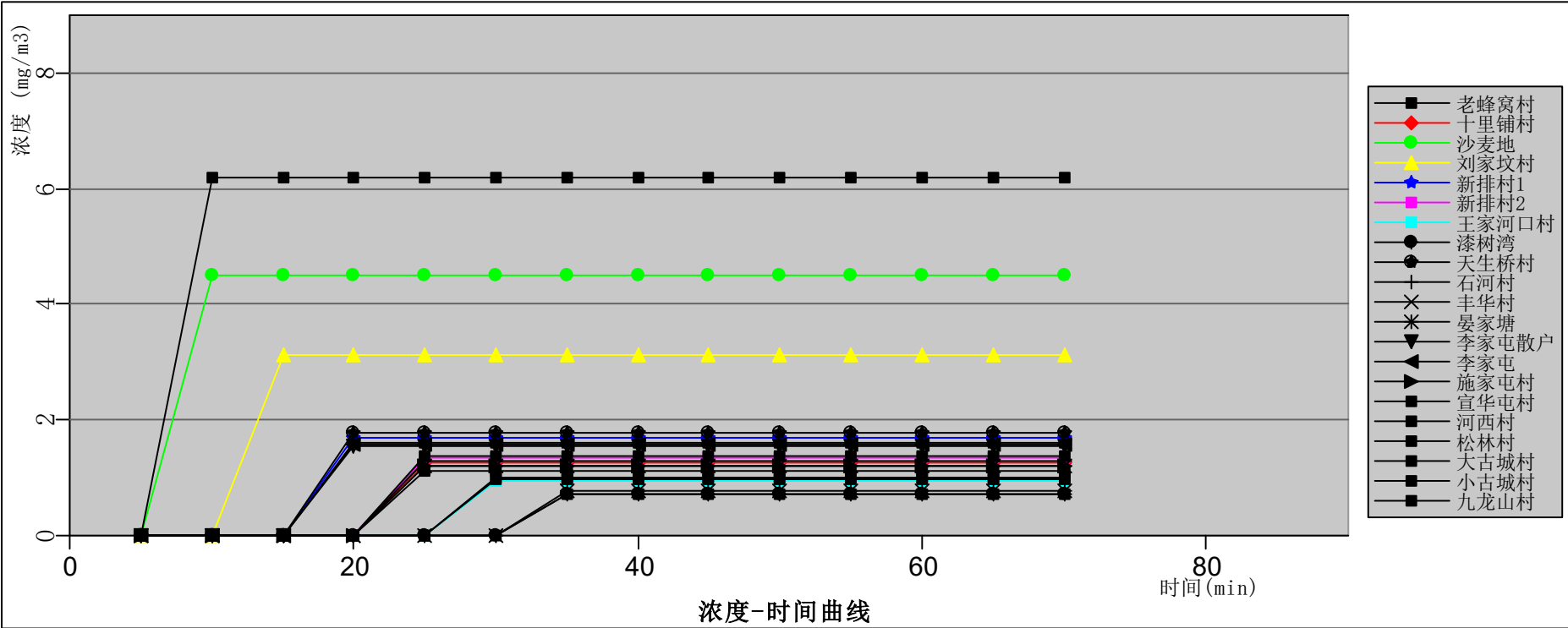
图12.6-68 粗苯罐泄漏最常见气象条件各敏感点处环己烷浓度随时间变化曲线图
