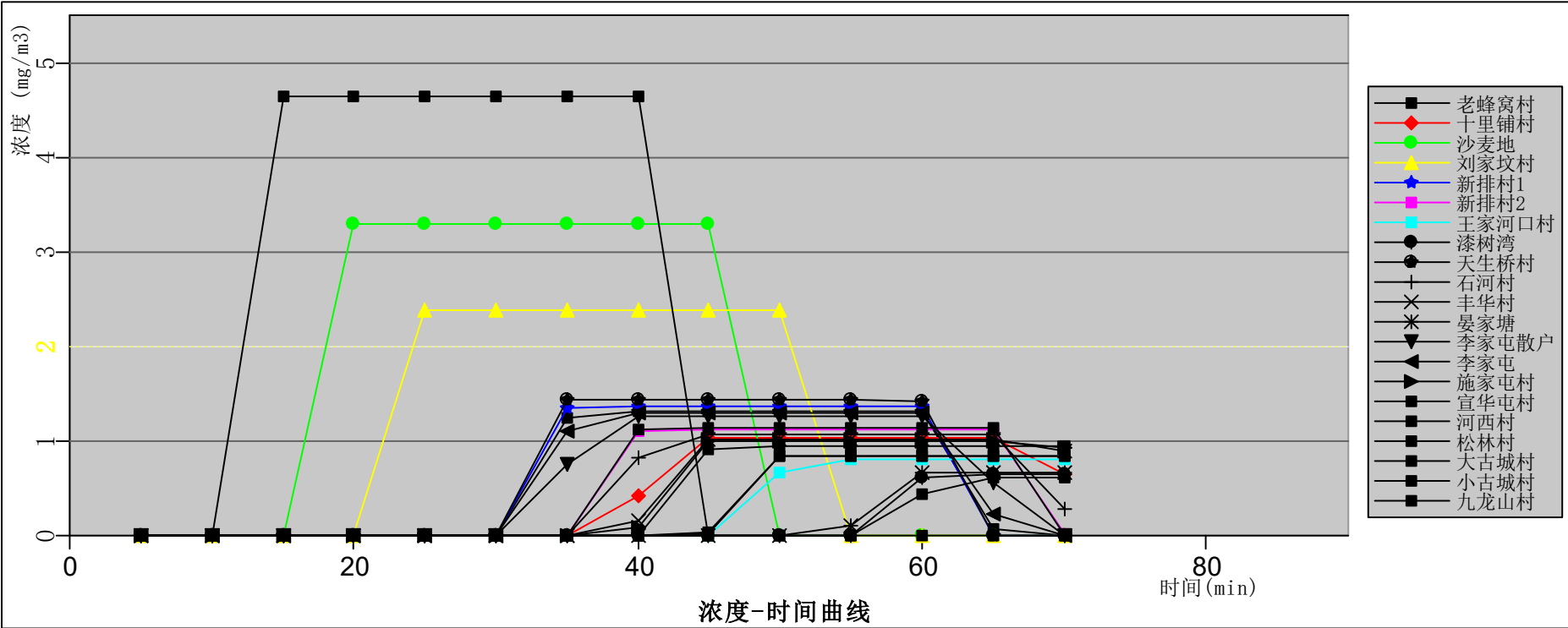
图12.6-83 粗苯罐火灾爆炸最不利气象条件各敏感点处SO 2 浓度随时间变化曲线图
