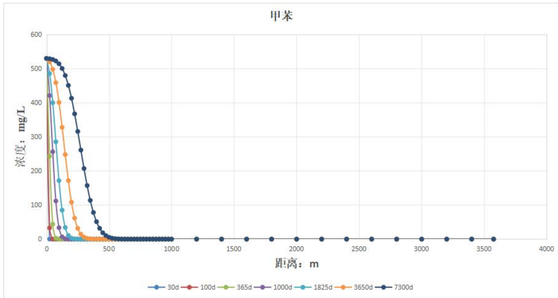
图7.9-2 管道渗漏后甲苯浓度变化图（标准值为0.7mg/L）
