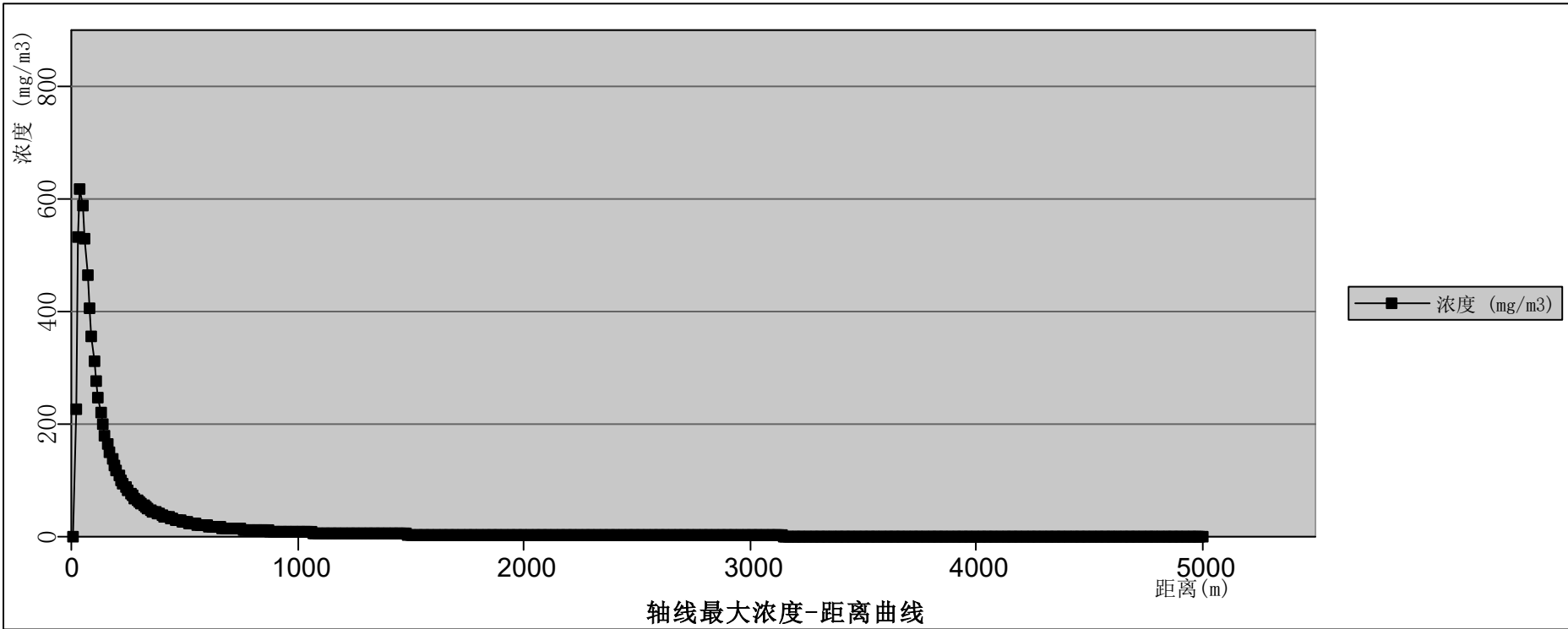
图 12.6-42 粗苯罐泄漏苯扩散轴线最大浓度——距离曲线（最常见气象条件下）
