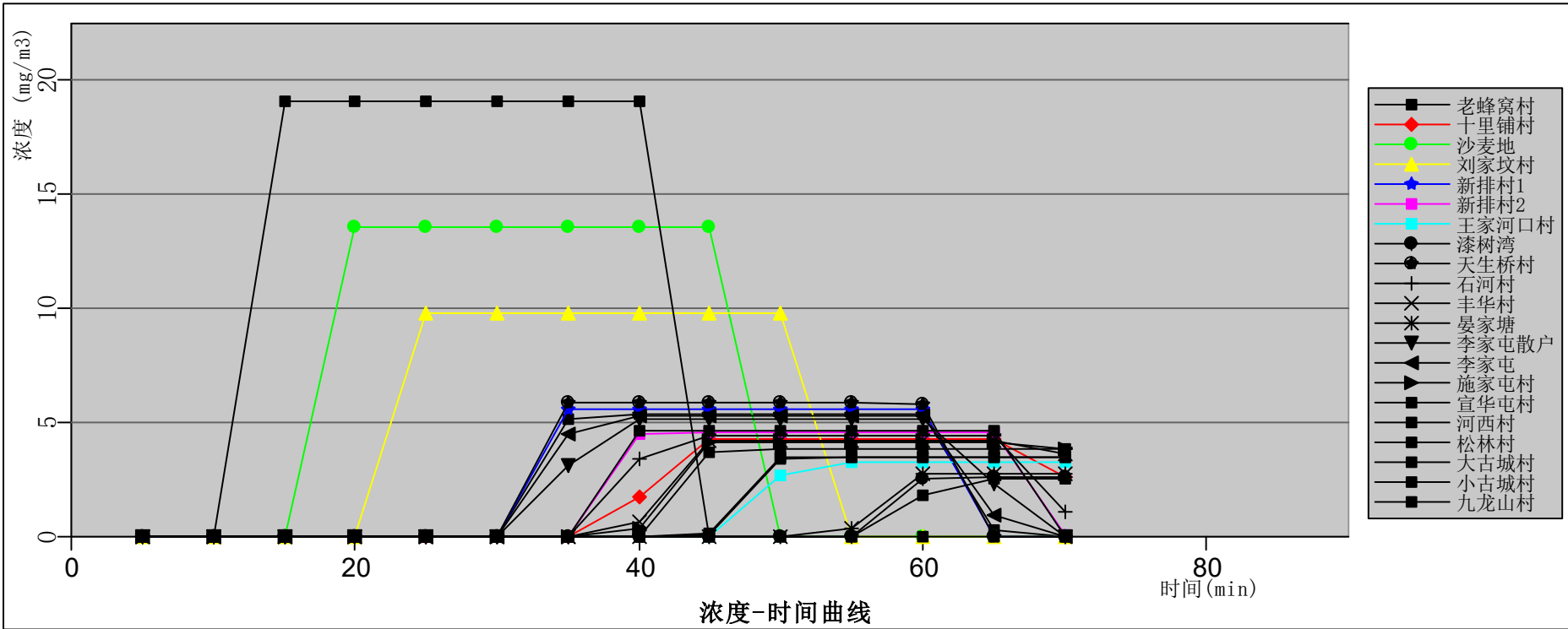
图12.6-33 回流罐火灾爆炸最不利气象条件各敏感点处CO浓度随时间变化曲线图
