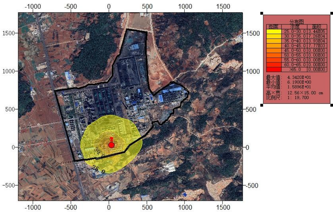
图 8.2-1 昼夜间噪声贡献值等值线图
