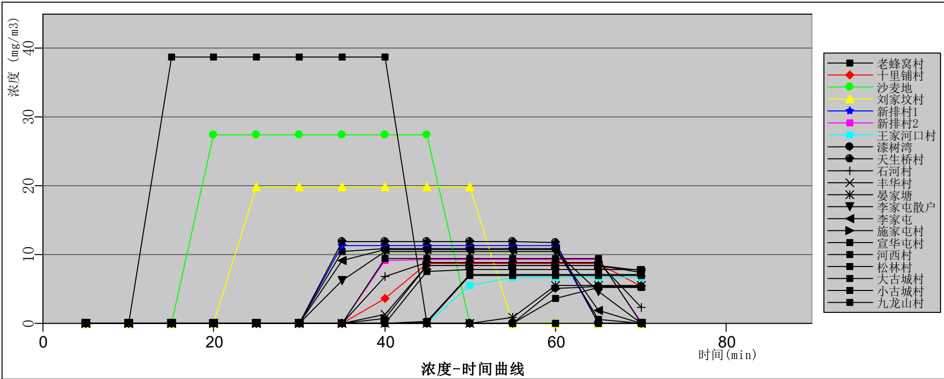
图12.6-77 粗苯罐火灾爆炸最不利气象条件各敏感点处CO浓度随时间变化曲线图
