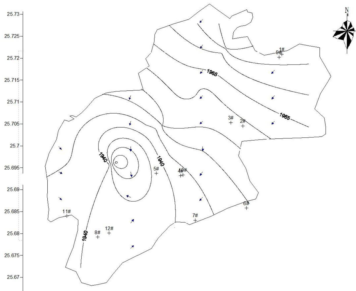
图 7.3-3 项目所在区域地下水水位及地下水流向图
