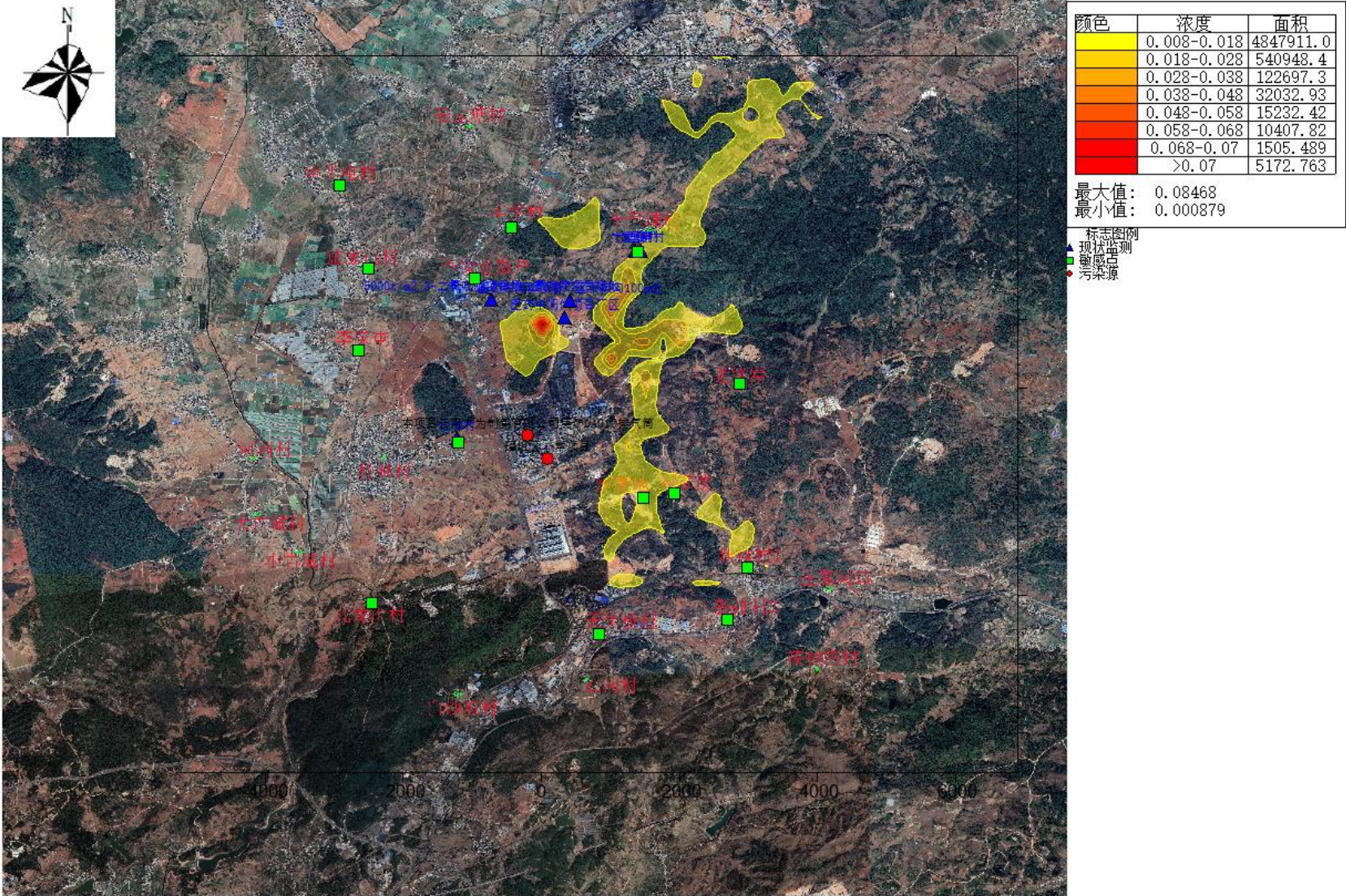
图5.2-11 甲苯1h平均质量浓度分布图
