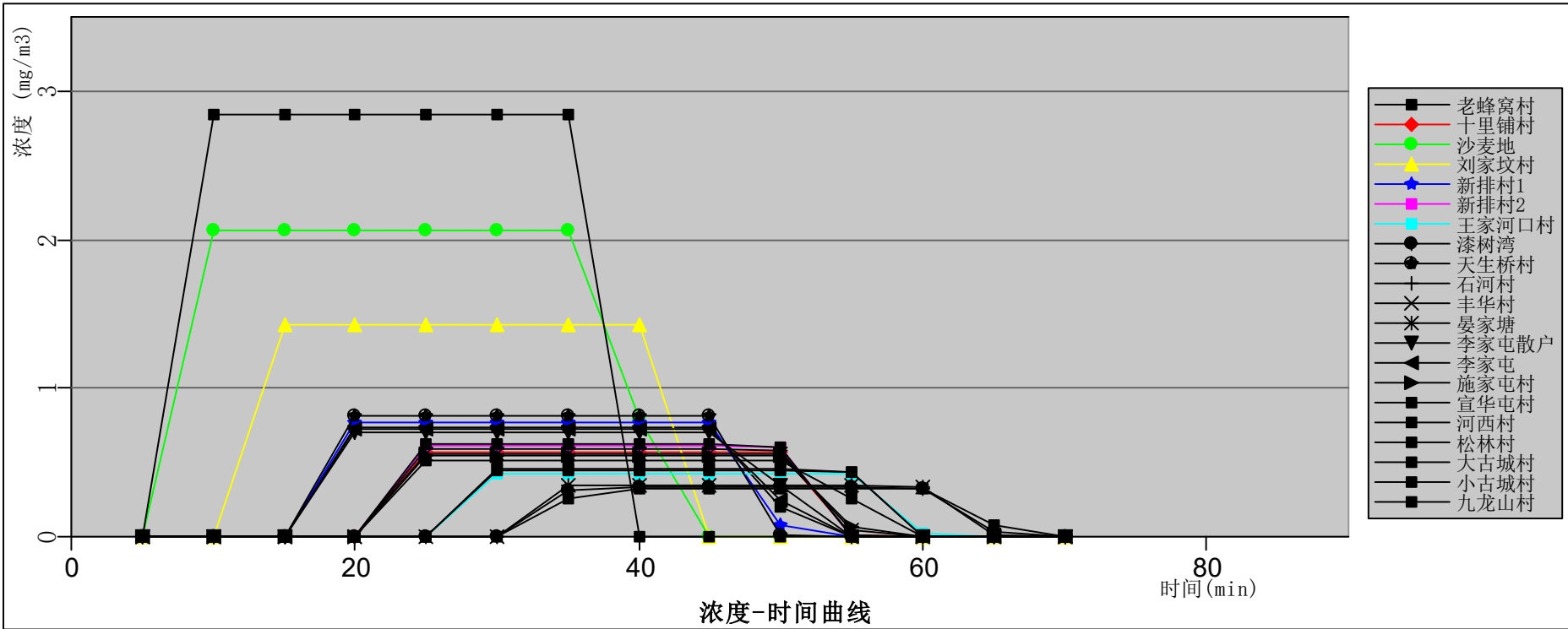
图12.6-34 回流罐火灾爆炸最常见气象条件各敏感点处CO浓度随时间变化曲线图
