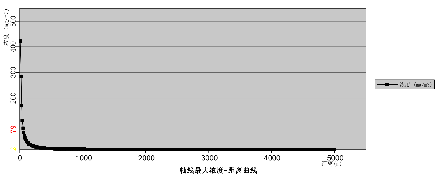
图 12.6-80 粗苯罐火灾爆炸 SO 2 扩散轴线最大浓度——距离曲线（最常见气象条件）
