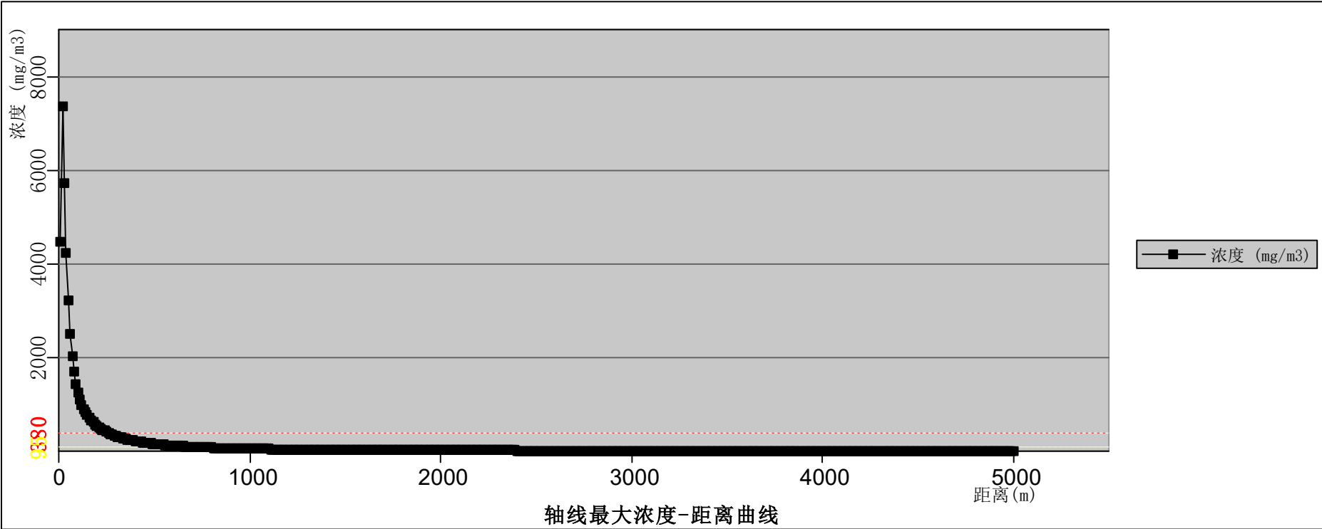
图 12.6-73 粗苯罐火灾爆炸 CO 扩散轴线最大浓度——距离曲线（最不利气象条件下）
