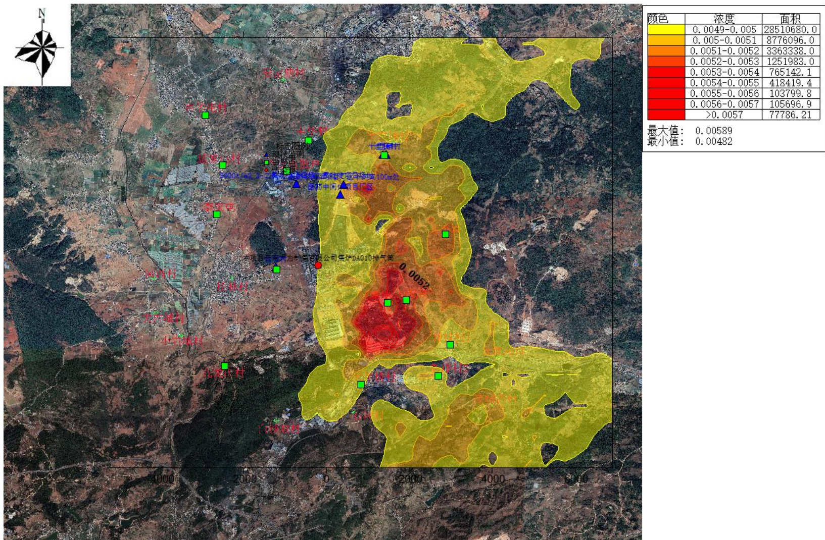
图5.2-14 全时段质量浓度分布图
