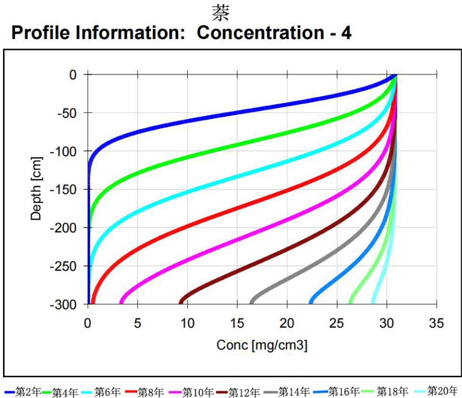
图 10.3-8 土壤不同年份不同深度萘浓度变化曲线
