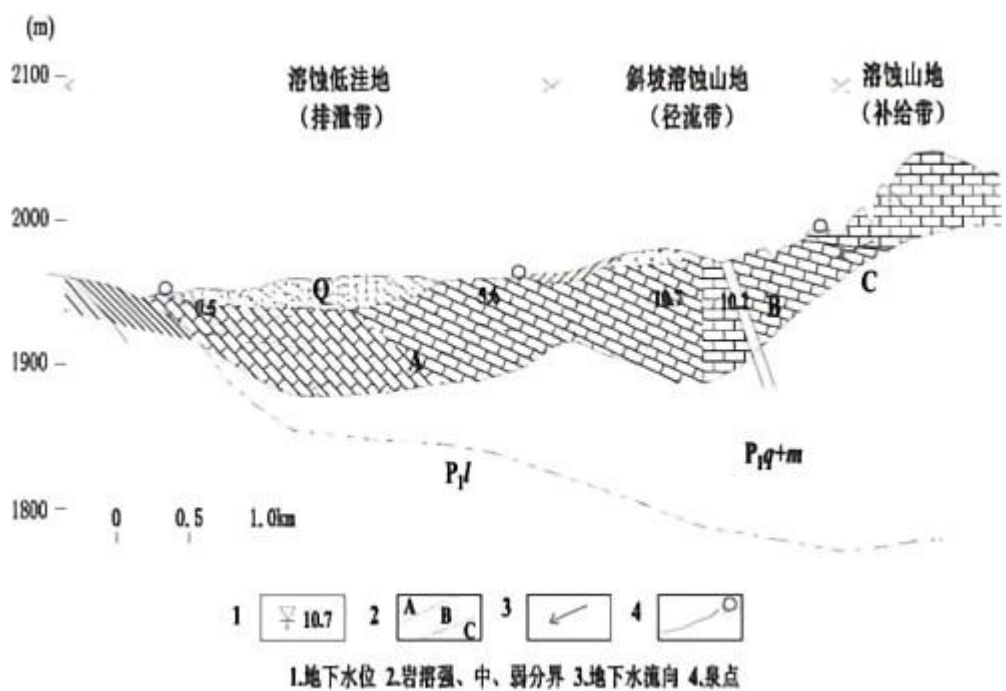
图 7.3-2 调查区水文地质图
