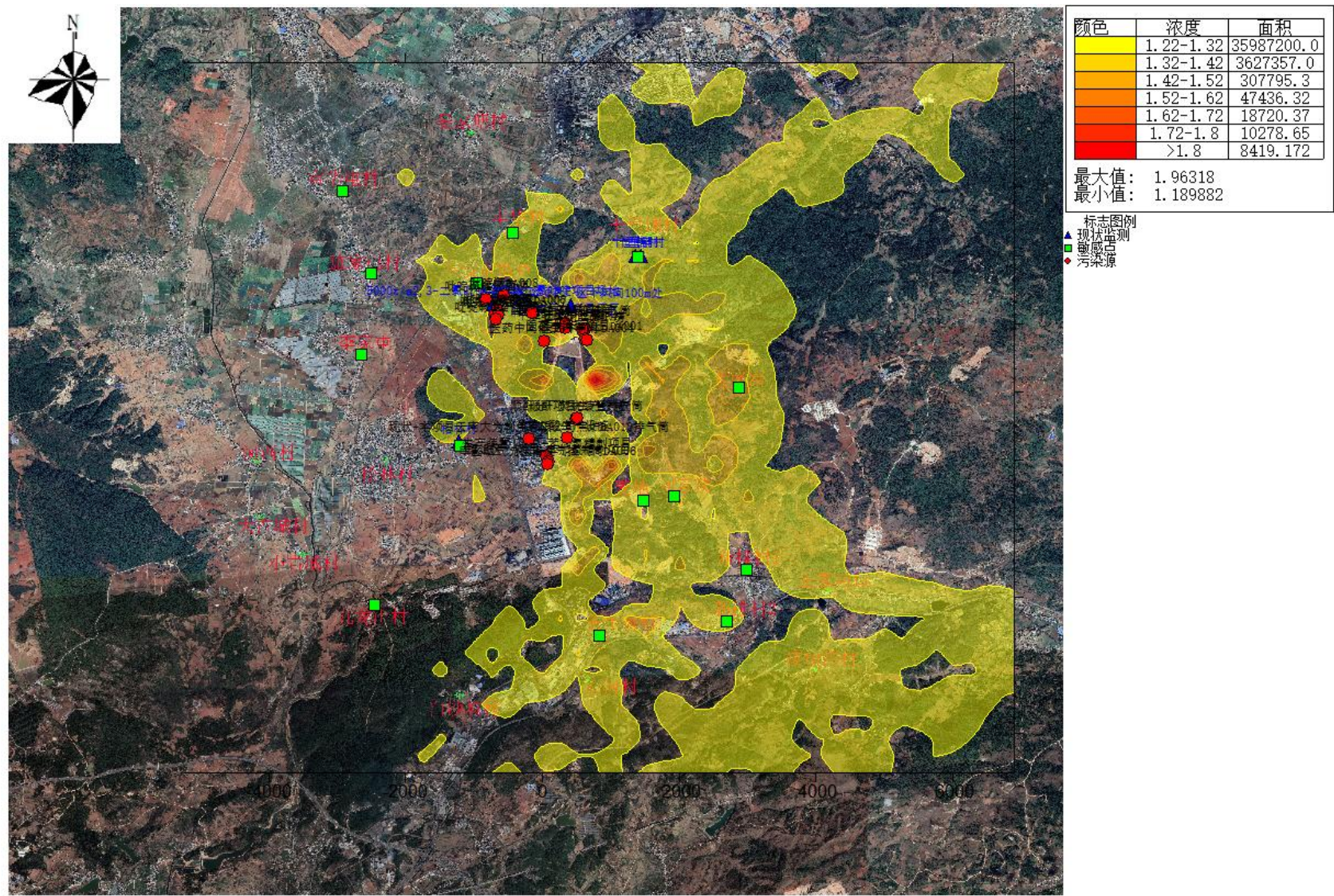
图5.2-9 非甲烷总烃1h平均质量浓度分布图
