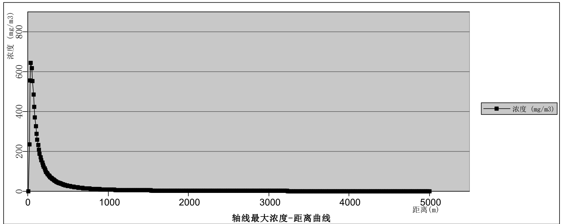
图 12.6-66 粗苯罐泄漏环己烷扩散轴线最大浓度——距离曲线（最常见气象条件）
