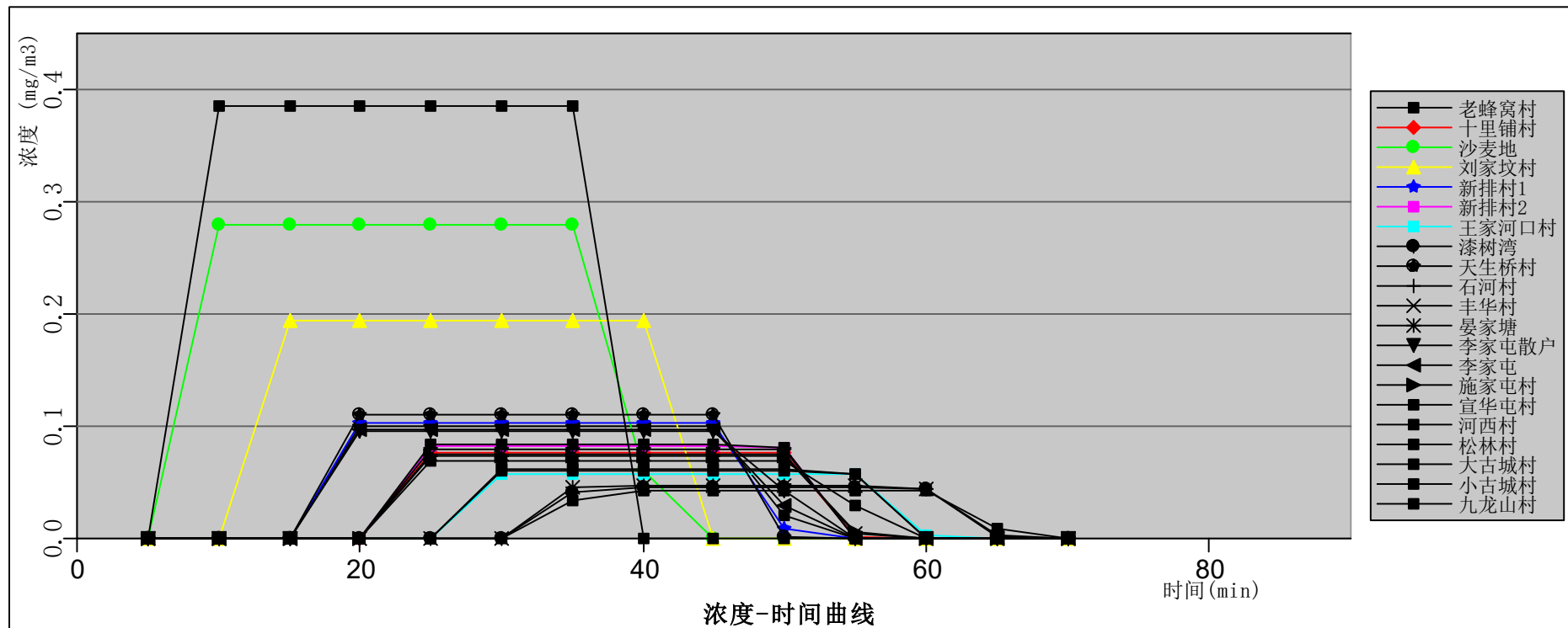
图12.6-72 粗苯罐泄漏最常见气象条件各敏感点处苯浓度随时间变化曲线图
