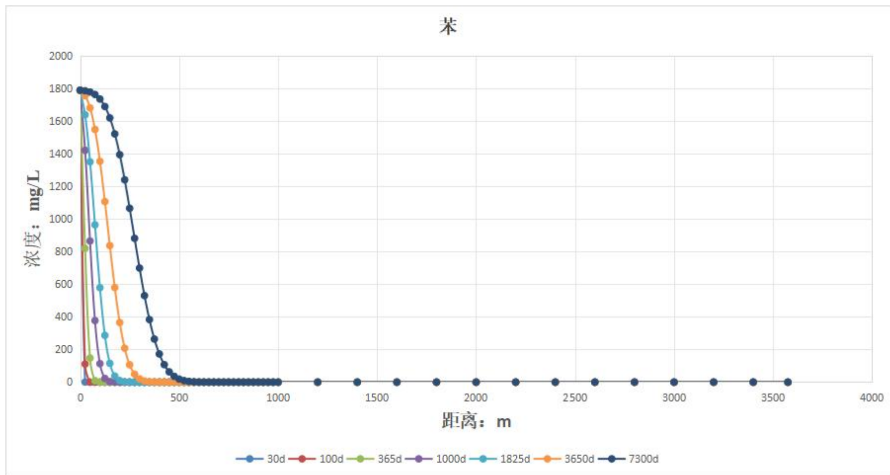
图7.9-1 管道渗漏后苯浓度变化图（标准值为0.01mg/L）
