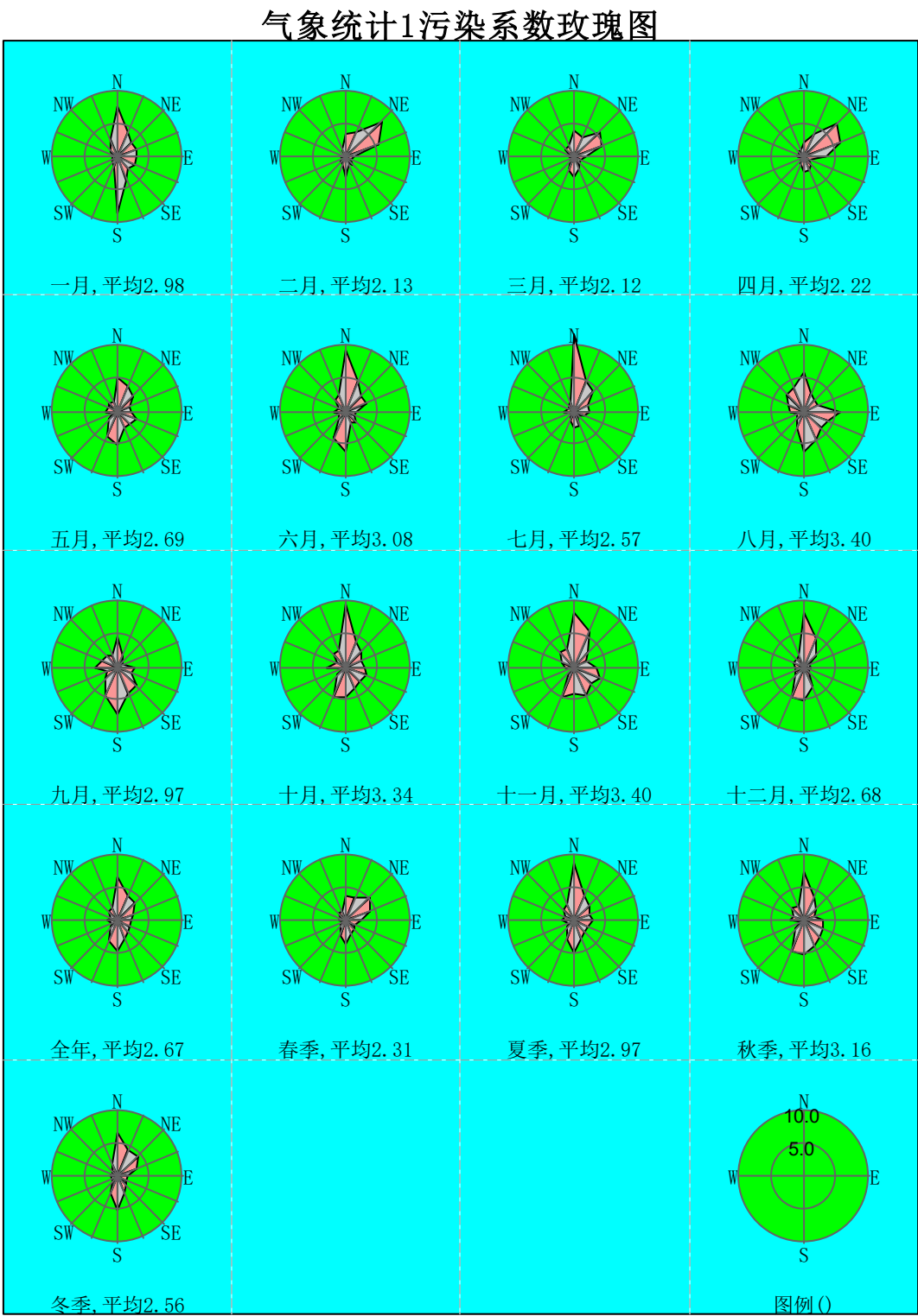
图 5.2-5 沾益区 2024 年全年和各季污染系数玫瑰图
