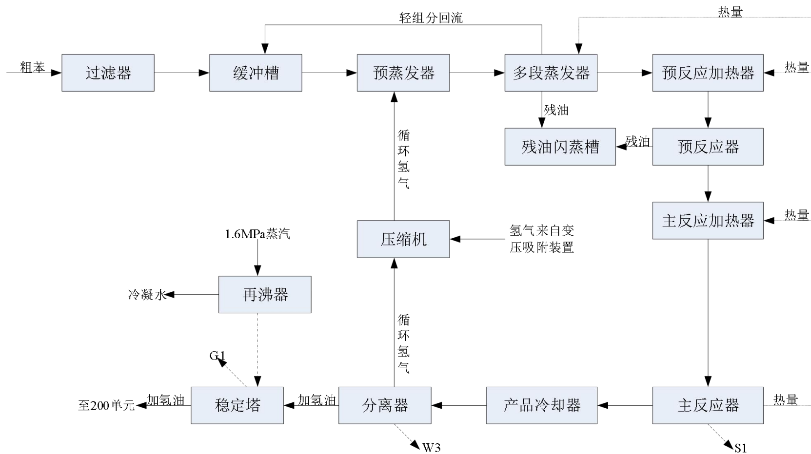
图2.2-1 100单元工艺流程图
