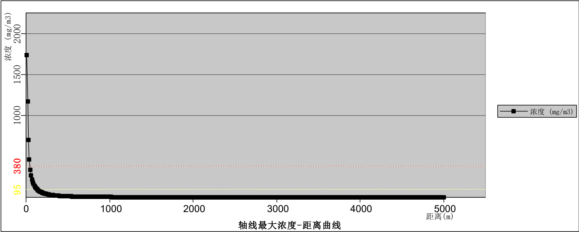
图 12.6-30 回流罐火灾爆炸 CO 扩散轴线最大浓度——距离曲线（最常见气象条件）
