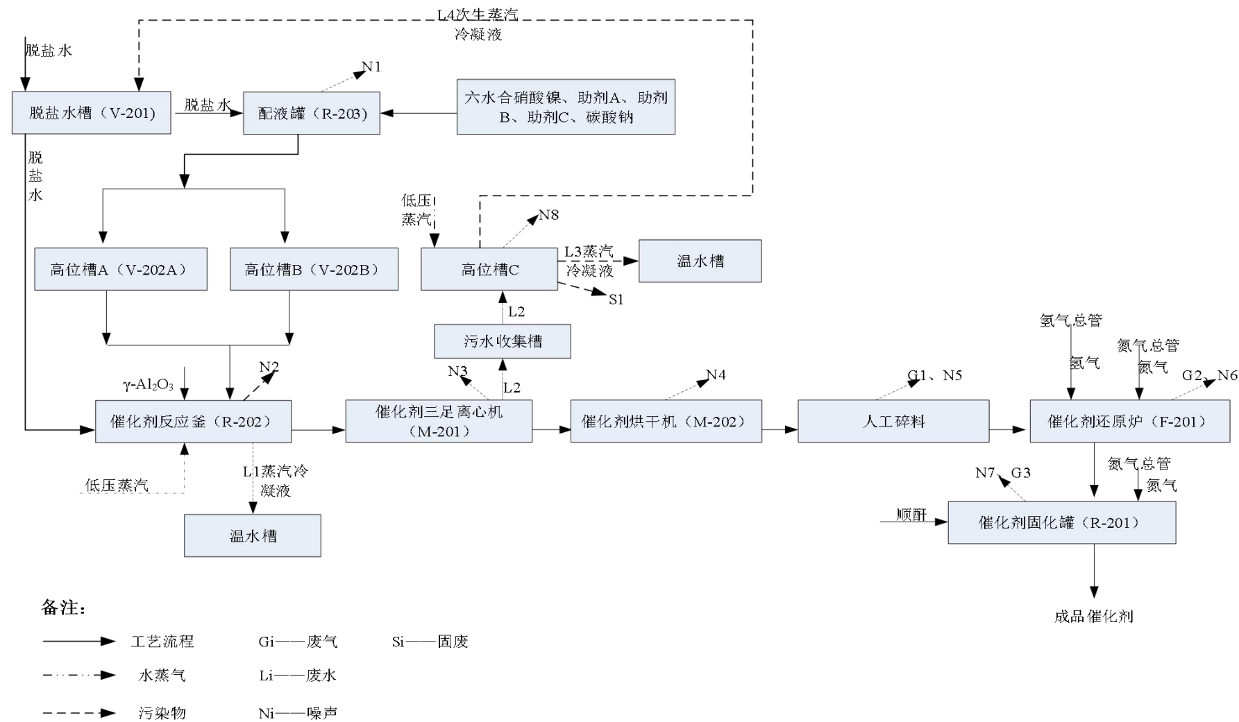
图2.2-12 催化剂生产工艺流程图
