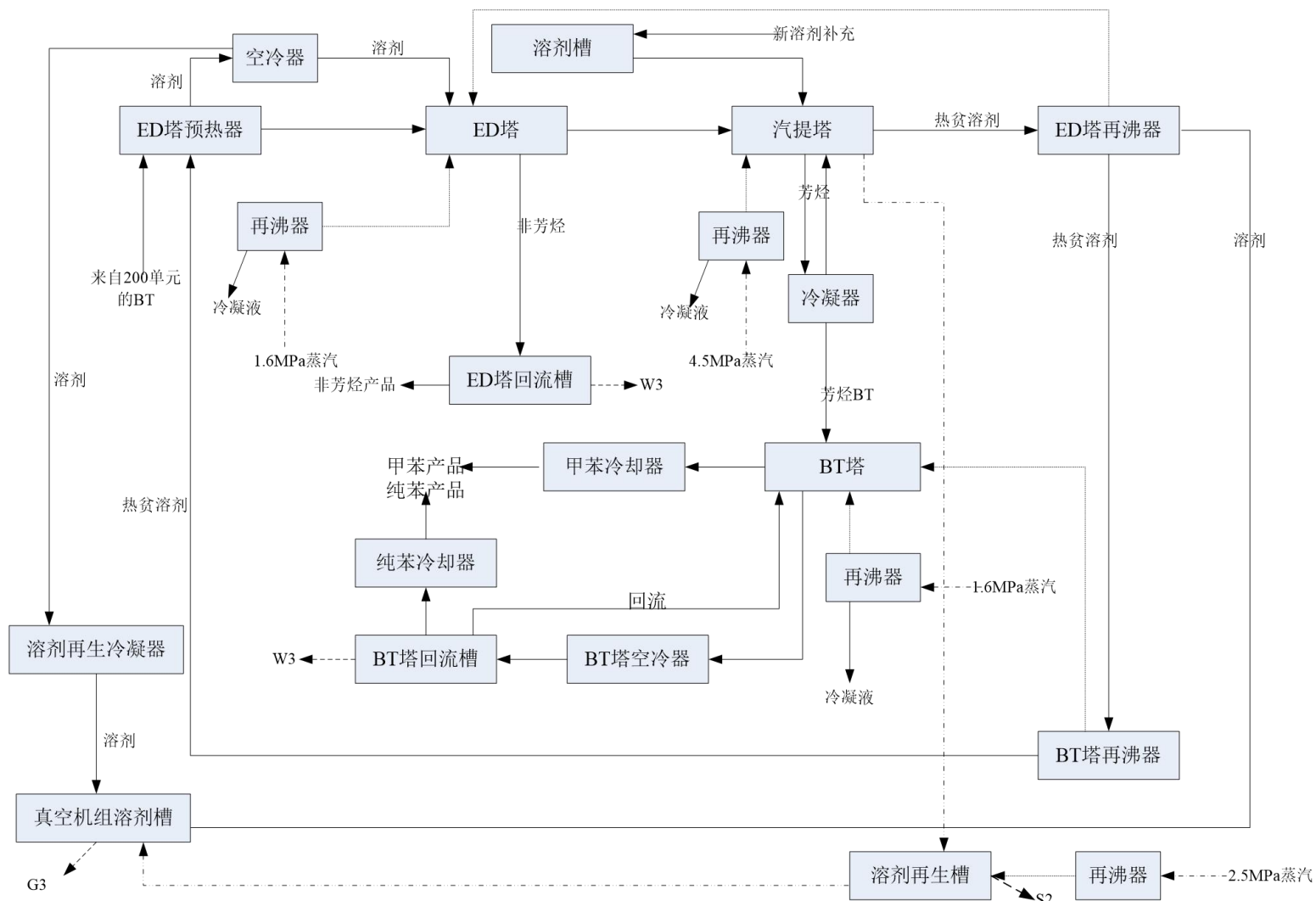
图2.2-3 300单元工艺流程图
