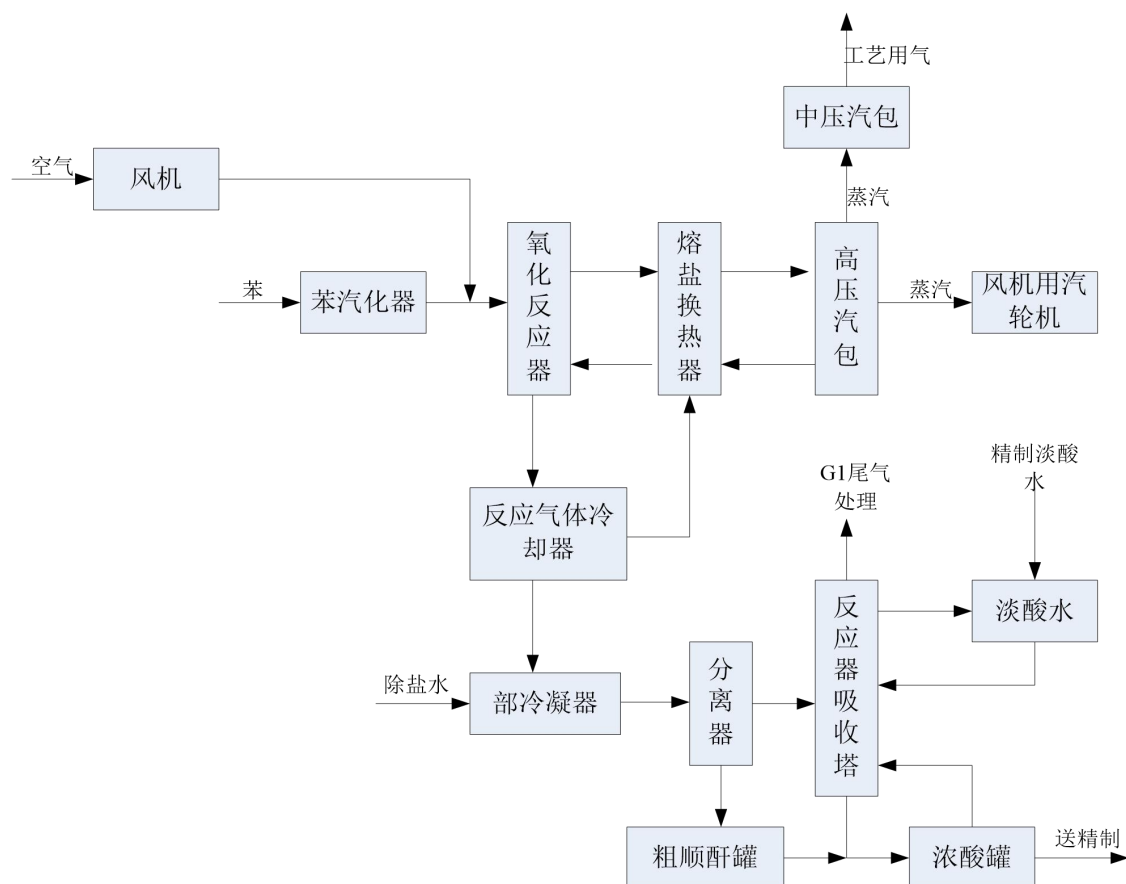
图2.2-5 顺酐苯氧化排污节点工艺流程示意图
