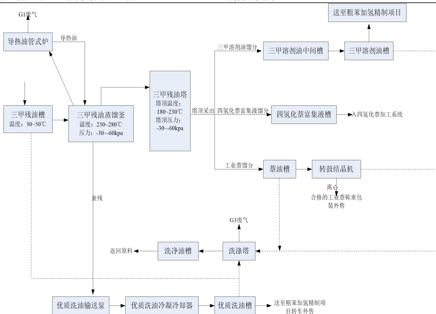
图2.2-9 三甲残油系统工艺流程图
