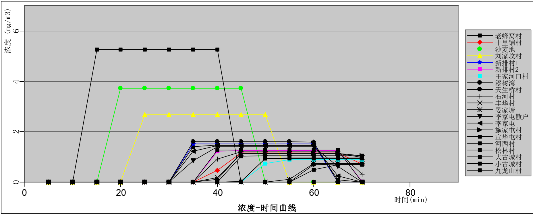
图12.6-11 回流罐泄漏最不利气象条件各敏感点处二甲苯浓度随时间变化曲线图
