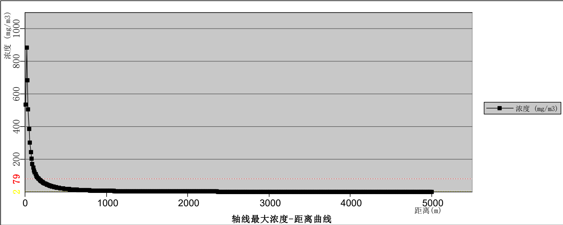
图 12.6-79 粗苯罐火灾爆炸 SO 2 扩散轴线最大浓度——距离曲线（最不利气象条件下）
