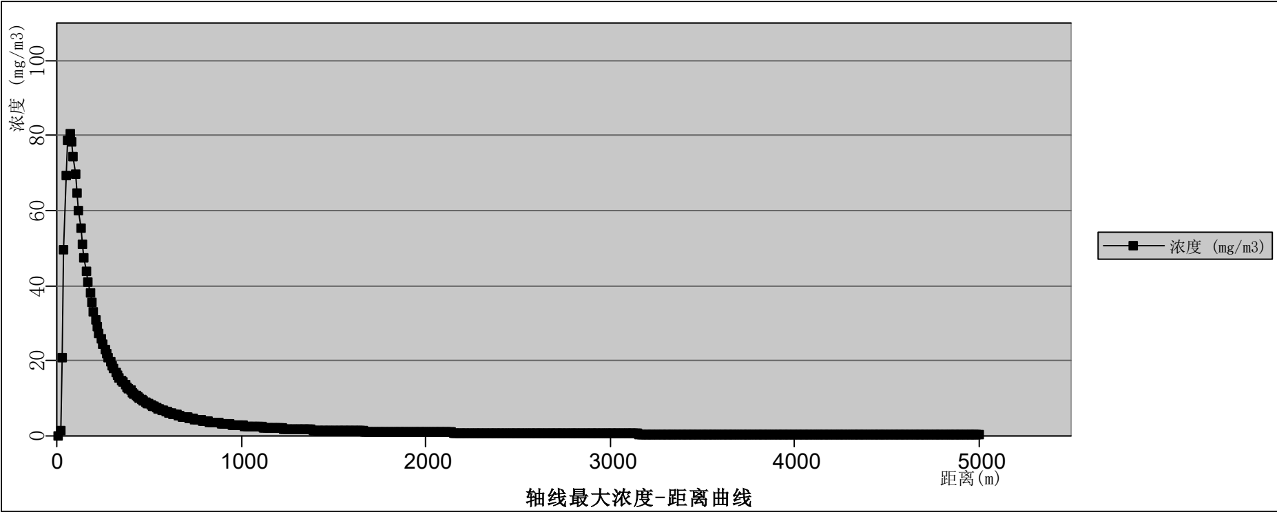
图 12.6-2 回流罐泄漏苯扩散轴线最大浓度——距离曲线（最常见气象条件下）
