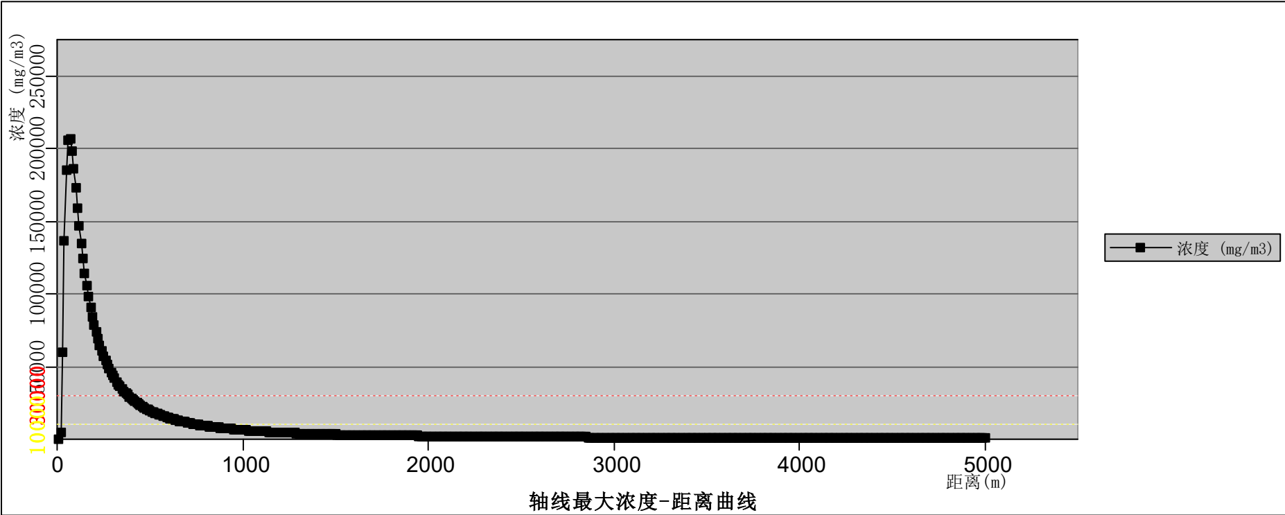
图 12.6-59 粗苯罐泄漏正己烷扩散轴线最大浓度——距离曲线（最不利气象条件下）
