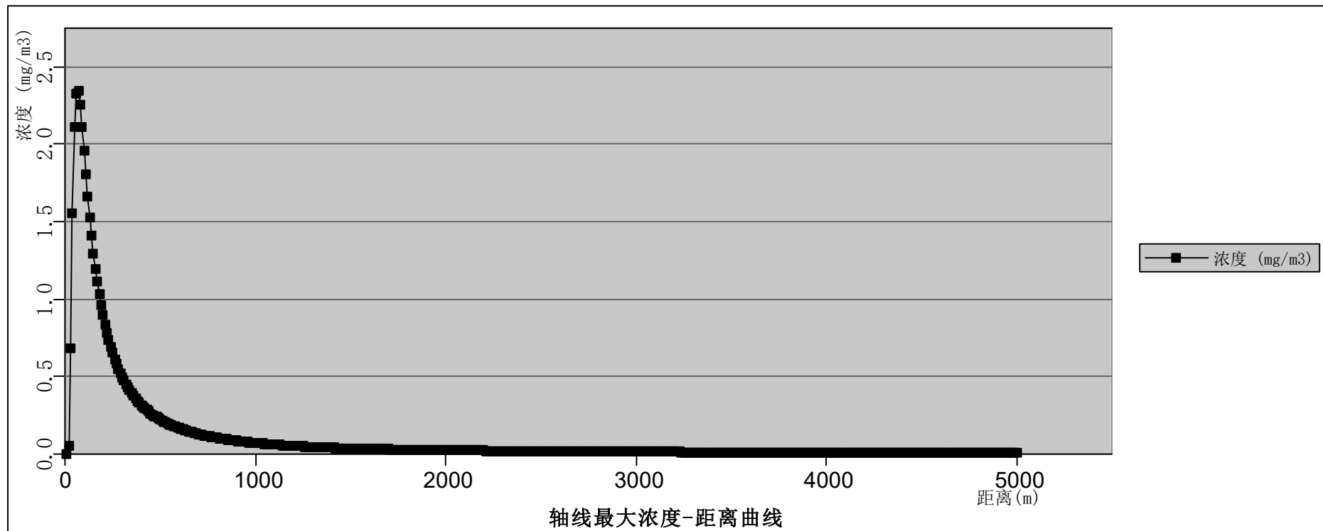
图 12.6-25 回流罐泄漏苯扩散轴线最大浓度——距离曲线（最不利气象条件下）
