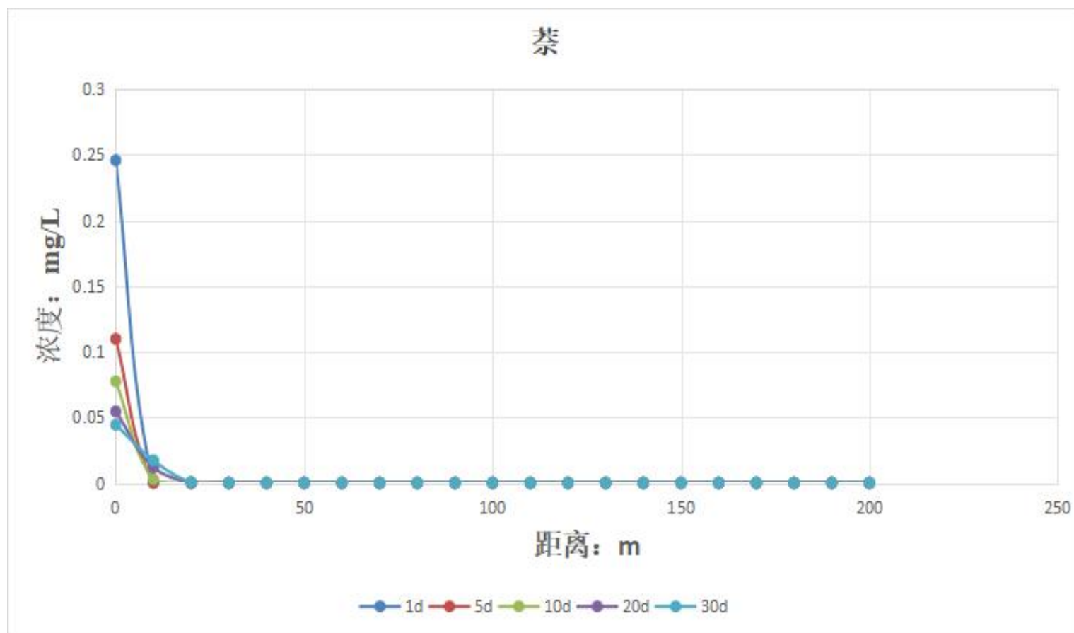
图12.6-89 粗苯罐泄漏萘下渗后浓度变化图（标准值为0.1mg/L）
