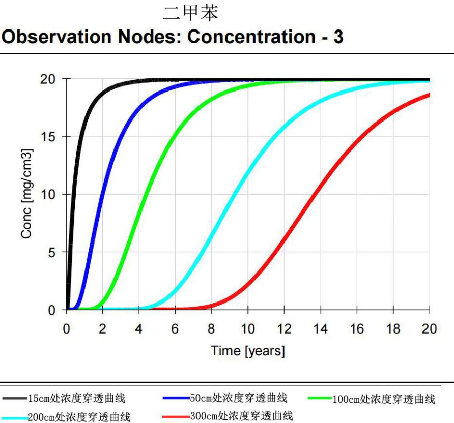
图 10.3-5 土壤不同深度处二甲苯浓度变化曲线
