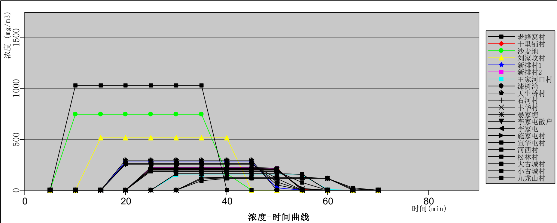
图12.6-64 粗苯罐泄漏最常见气象条件各敏感点处正己烷浓度随时间变化曲线图
