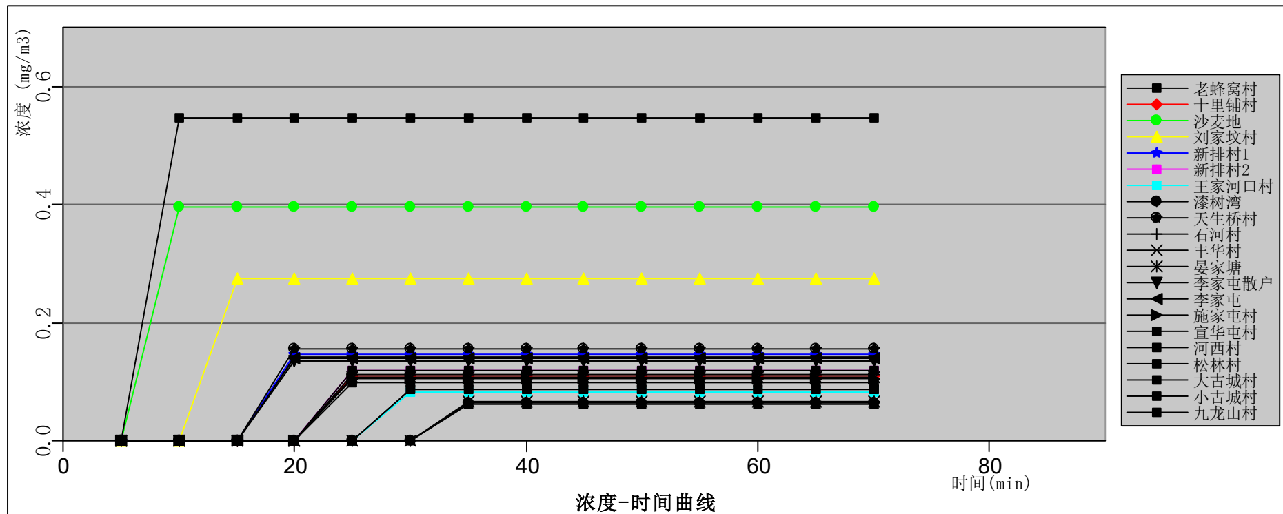
图12.6-24 回流罐泄漏最常见气象条件各敏感点处环己烷浓度随时间变化曲线图
