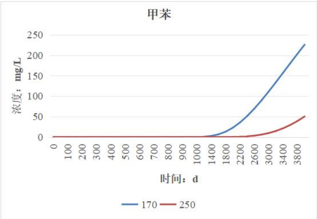
图 7.9-6 固定位置甲苯（监测井和最近厂界处）污染物浓度穿透曲线图
