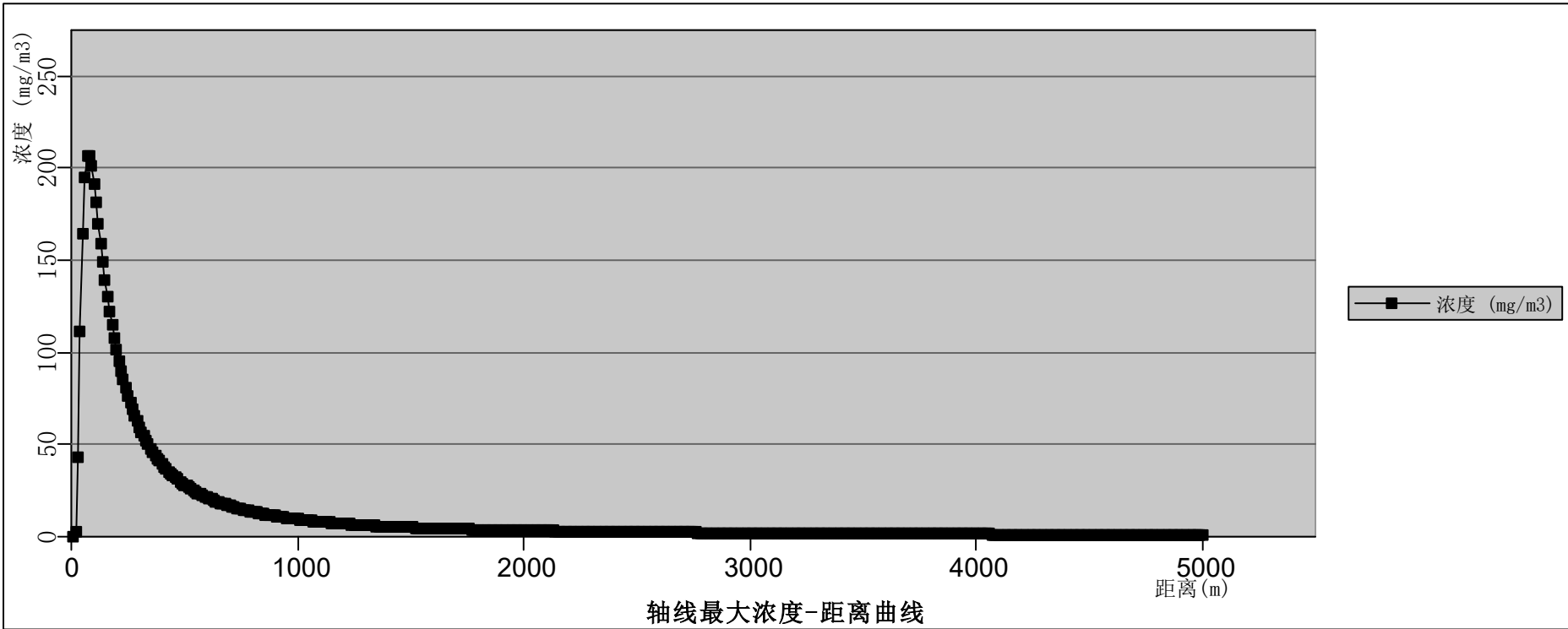
图 12.6-45 粗苯罐泄漏甲苯扩散轴线最大浓度——距离曲线（最不利气象条件下）
