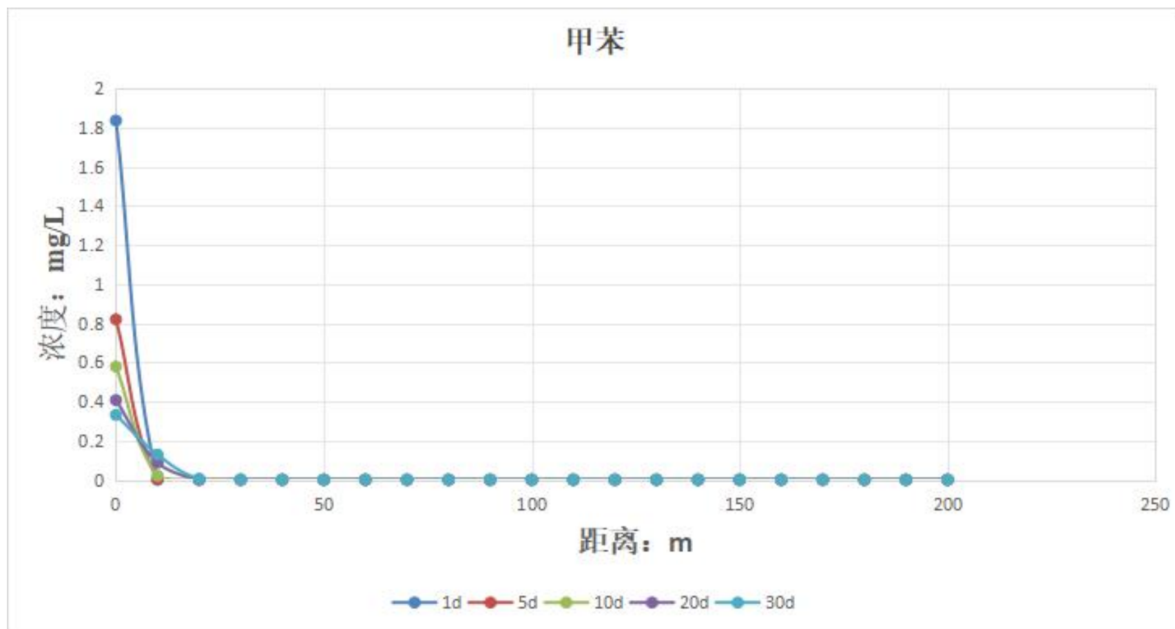
图12.6-87 粗苯罐泄漏甲苯下渗后浓度变化图（标准值为0.7mg/L）
