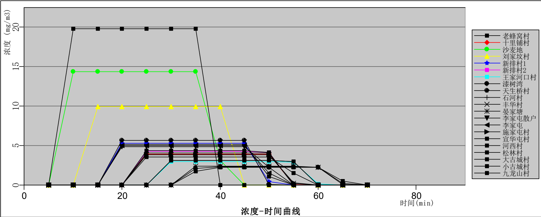
图12.6-20 回流罐泄漏最常见气象条件各敏感点处正己烷浓度随时间变化曲线图
