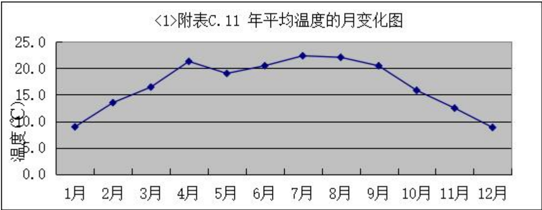
图 5.2-6 沾益区 2024 年月平均气温变化曲线
