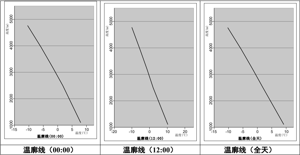
图 5.2-7 00:00, 12:00 及全天温廓线图
