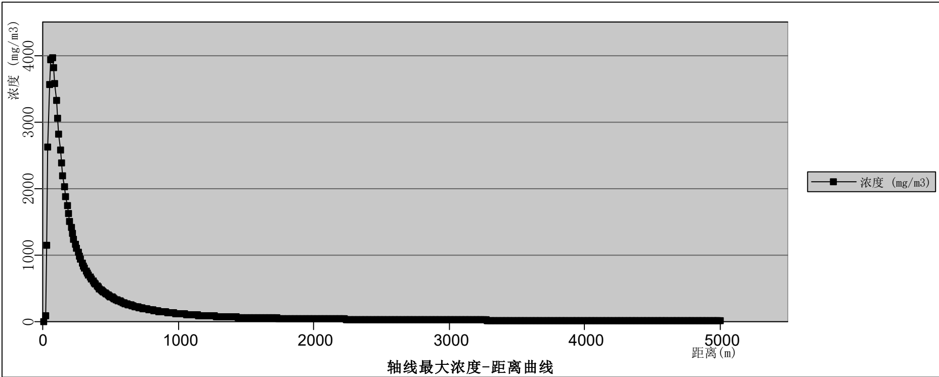
图 12.6-17 回流罐泄漏正己烷扩散轴线最大浓度——距离曲线（最不利气象条件下）
