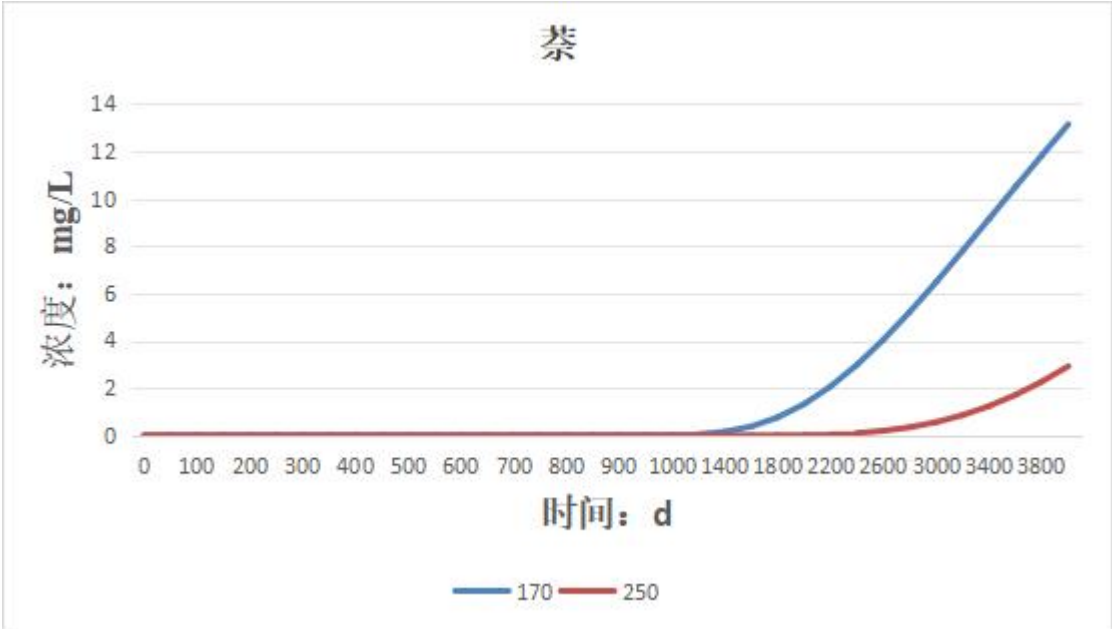
图 7.9-8 固定位置萘（监测井和最近厂界处）污染物浓度穿透曲线图
