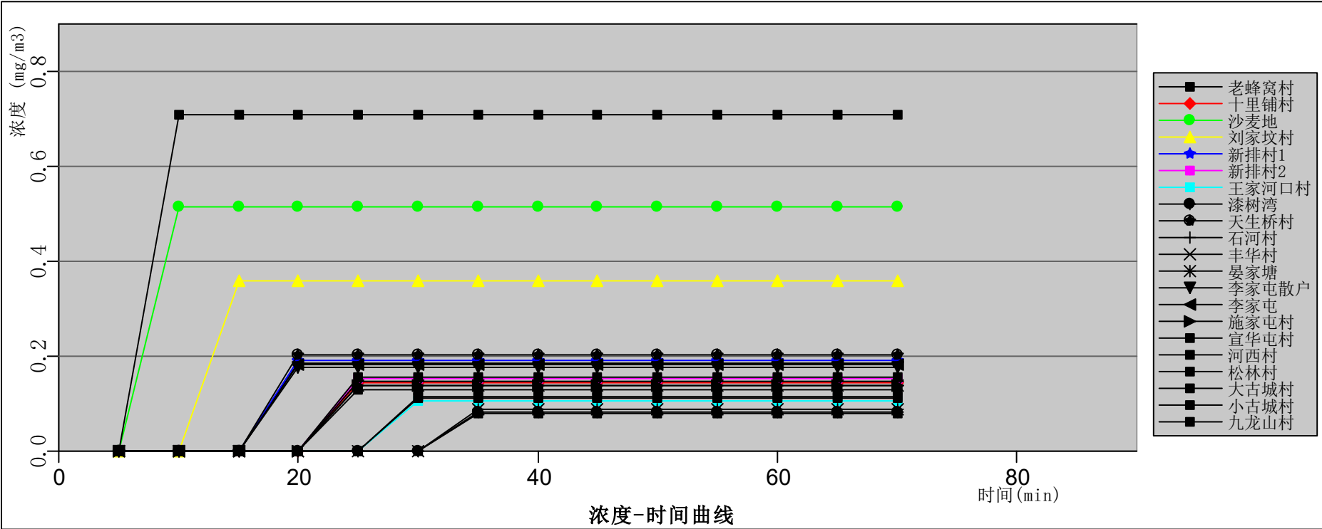
图12.6-58 粗苯罐泄漏最常见气象条件各敏感点处乙苯浓度随时间变化曲线图
