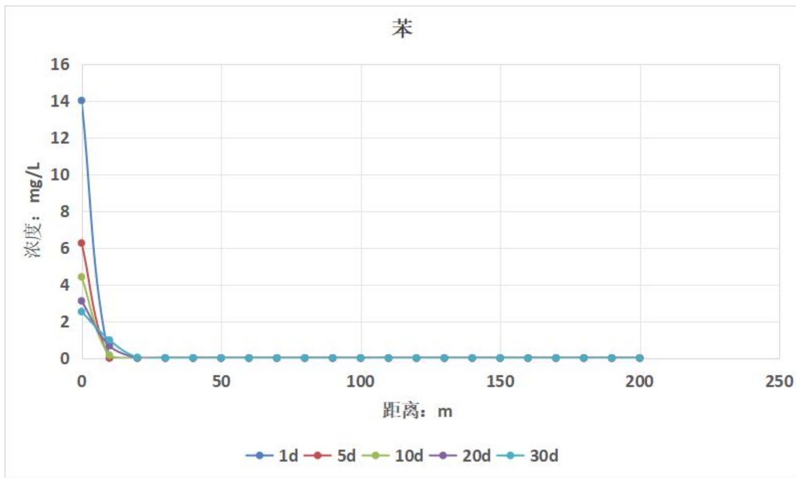
图12.6-86 粗苯罐泄漏苯下渗后苯浓度变化图（标准值为0.01mg/L）
