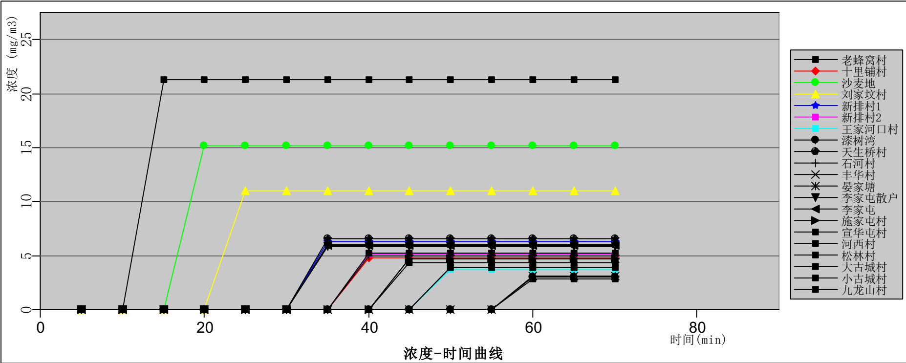
图 12.6-43 粗苯罐泄漏最不利气象条件各敏感点处苯浓度随时间变化曲线图
