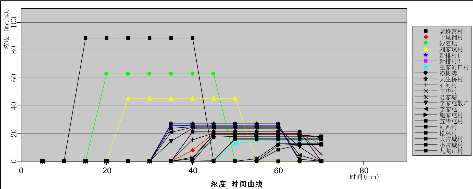
图12.6-19 回流罐泄漏最不利气象条件各敏感点处正己烷浓度随时间变化曲线图
