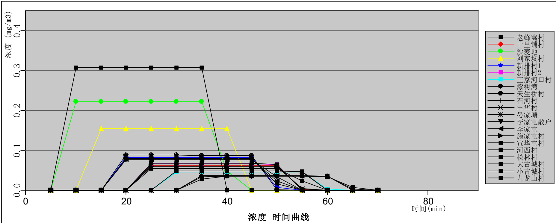
图12.6-40 回流罐火灾爆炸最常见气象条件各敏感点处SO 2 浓度随时间变化曲线图
