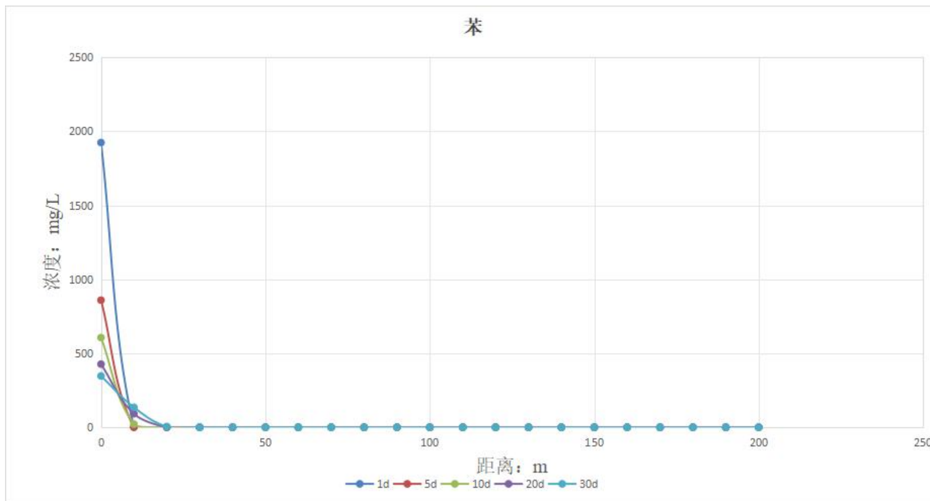
图12.6-90 回流罐泄漏苯下渗后苯浓度变化图（标准值为0.01mg/L）
