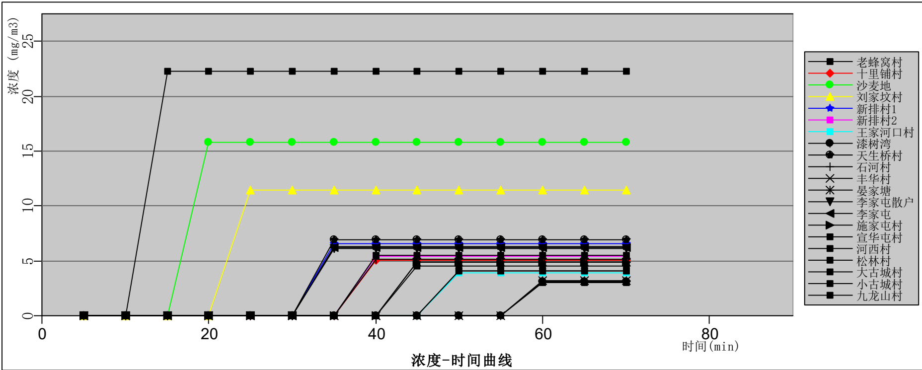
图12.6-67 粗苯罐泄漏最不利气象条件各敏感点处环己烷浓度随时间变化曲线图
