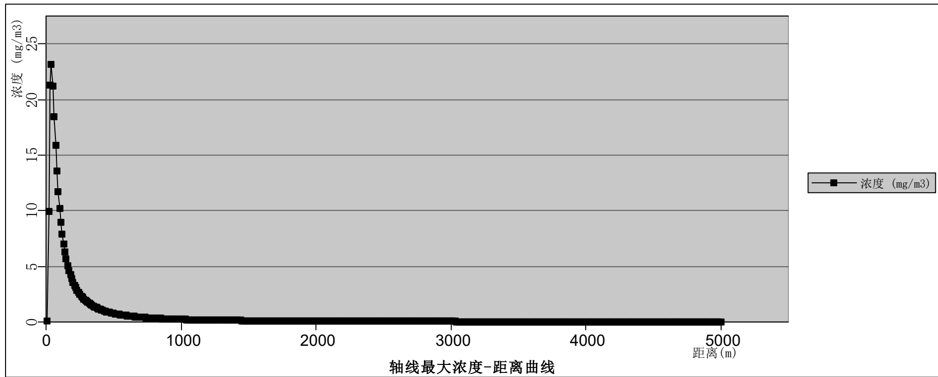
图 12.6-6 回流罐泄漏甲苯扩散轴线最大浓度——距离曲线（最常见气象条件）
