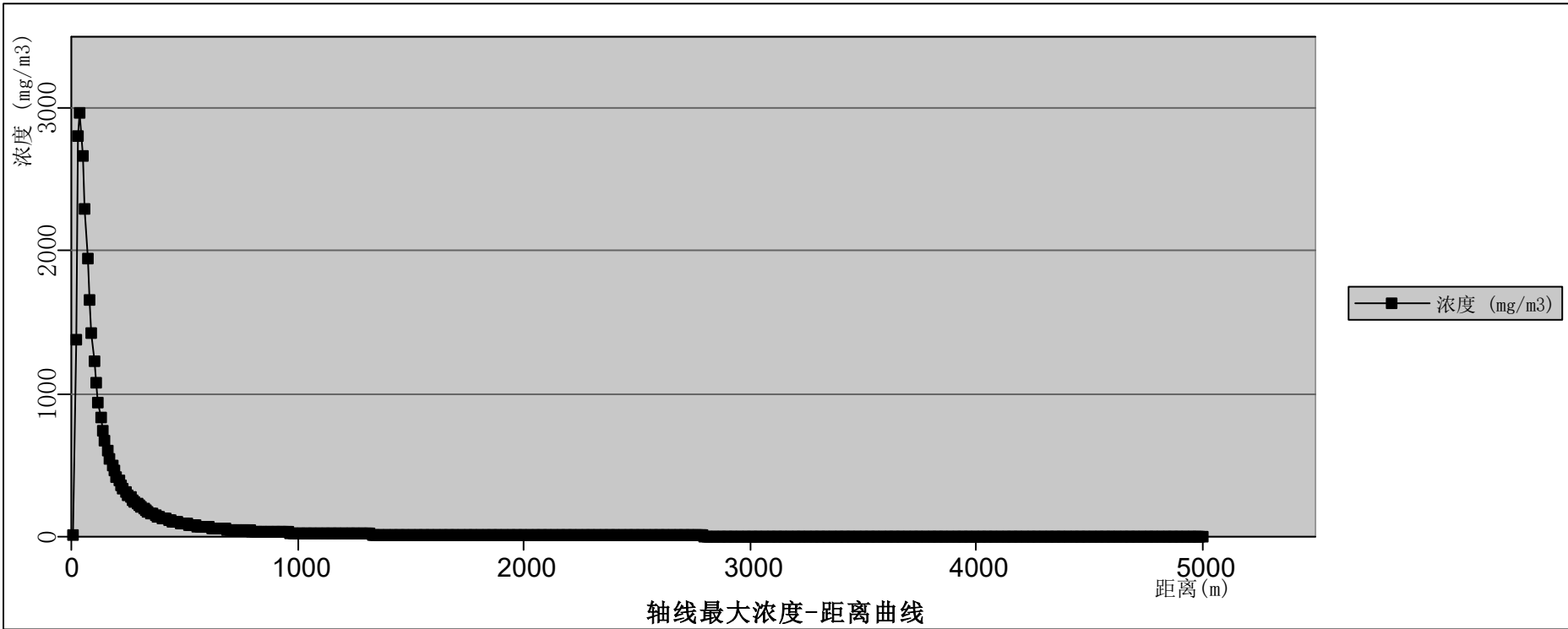
图 12.6-18 回流罐泄漏正己烷扩散轴线最大浓度——距离曲线（最常见气象条件）
