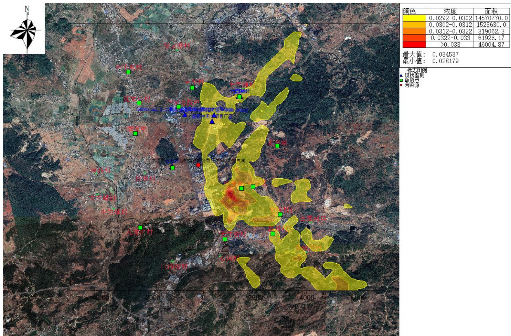
图 5.2-13 98%保证率日平均质量浓度分布图
