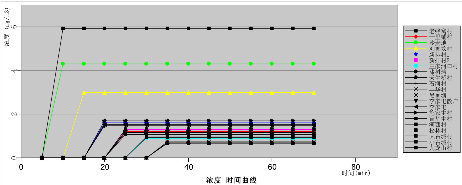
图 12.6-44 粗苯罐泄漏最常见气象条件各敏感点处苯浓度随时间变化曲线图
