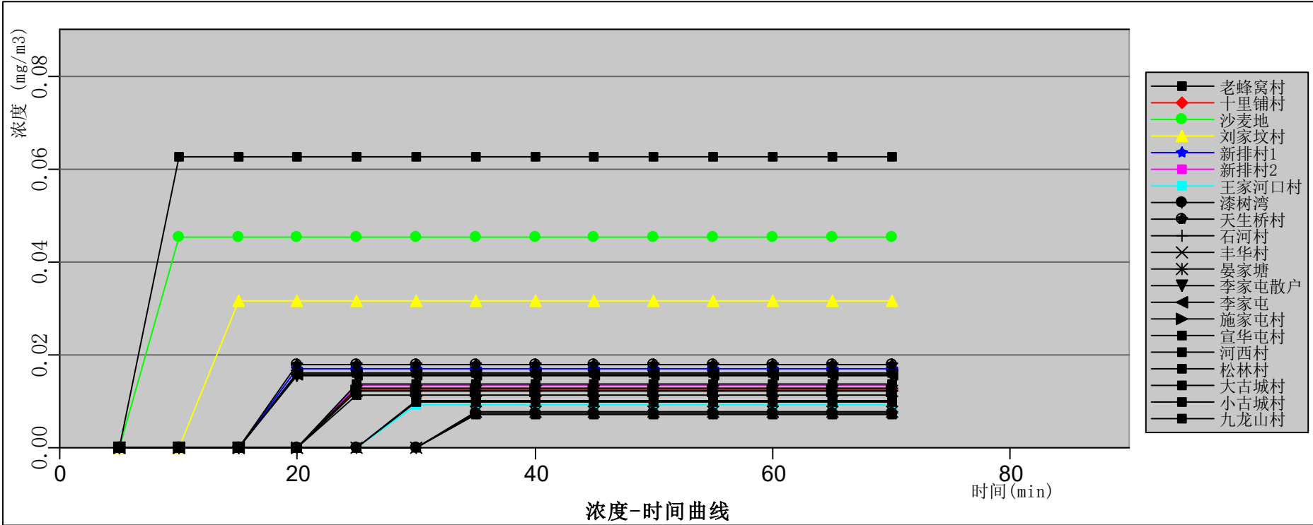
图12.6-16 回流罐泄漏最常见气象条件各敏感点处乙苯浓度随时间变化曲线图
