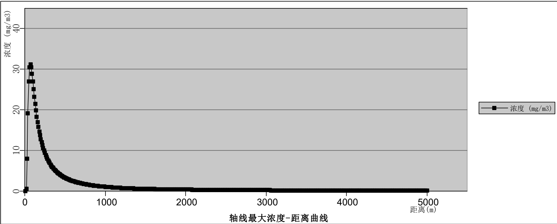
图 12.6-5 回流罐泄漏甲苯扩散轴线最大浓度——距离曲线（最不利气象条件下）
