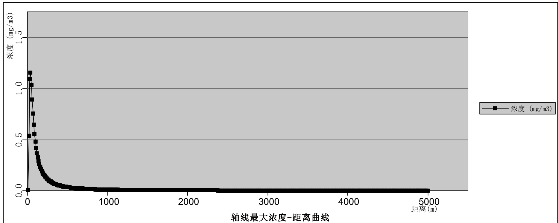
图 12.6-26 回流罐泄漏萘扩散轴线最大浓度——距离曲线（最常见气象条件）
