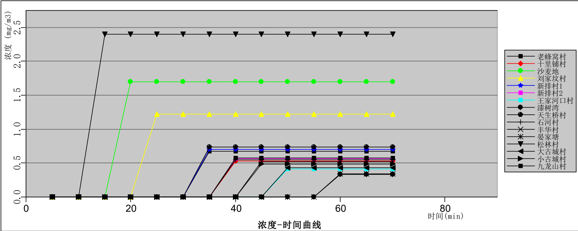
图 12.6-3 回流罐泄漏最不利气象条件各敏感点处苯浓度随时间变化曲线图
