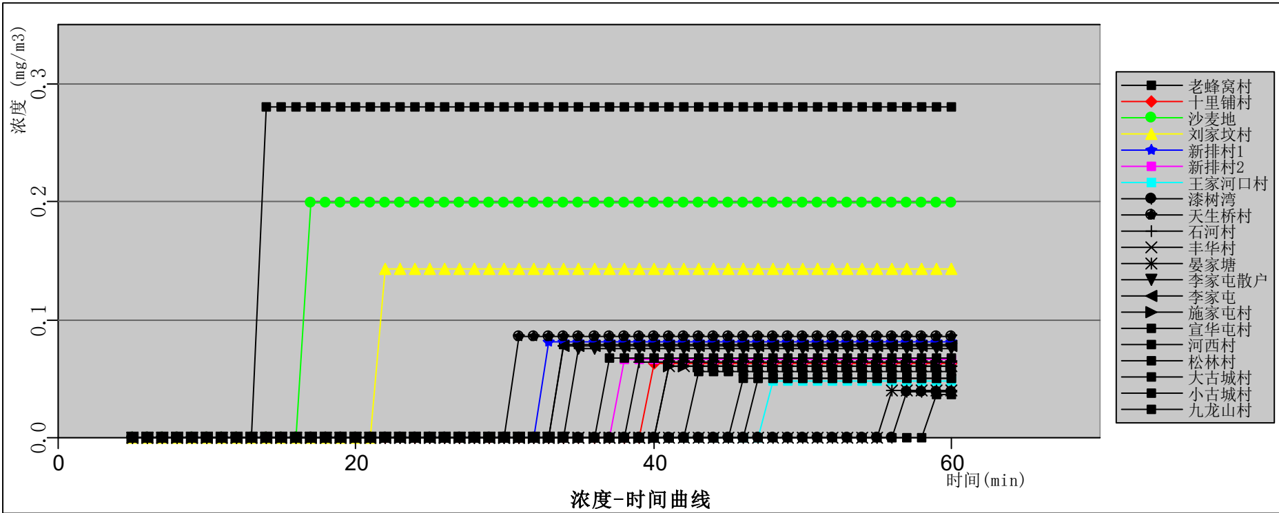
图12.6-15 回流罐泄漏最不利气象条件各敏感点处乙苯浓度随时间变化曲线图
