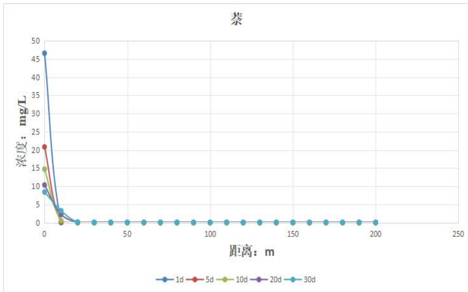
图12.6-93 回流罐泄漏萘下渗后浓度变化图（标准值为0.1mg/L）
