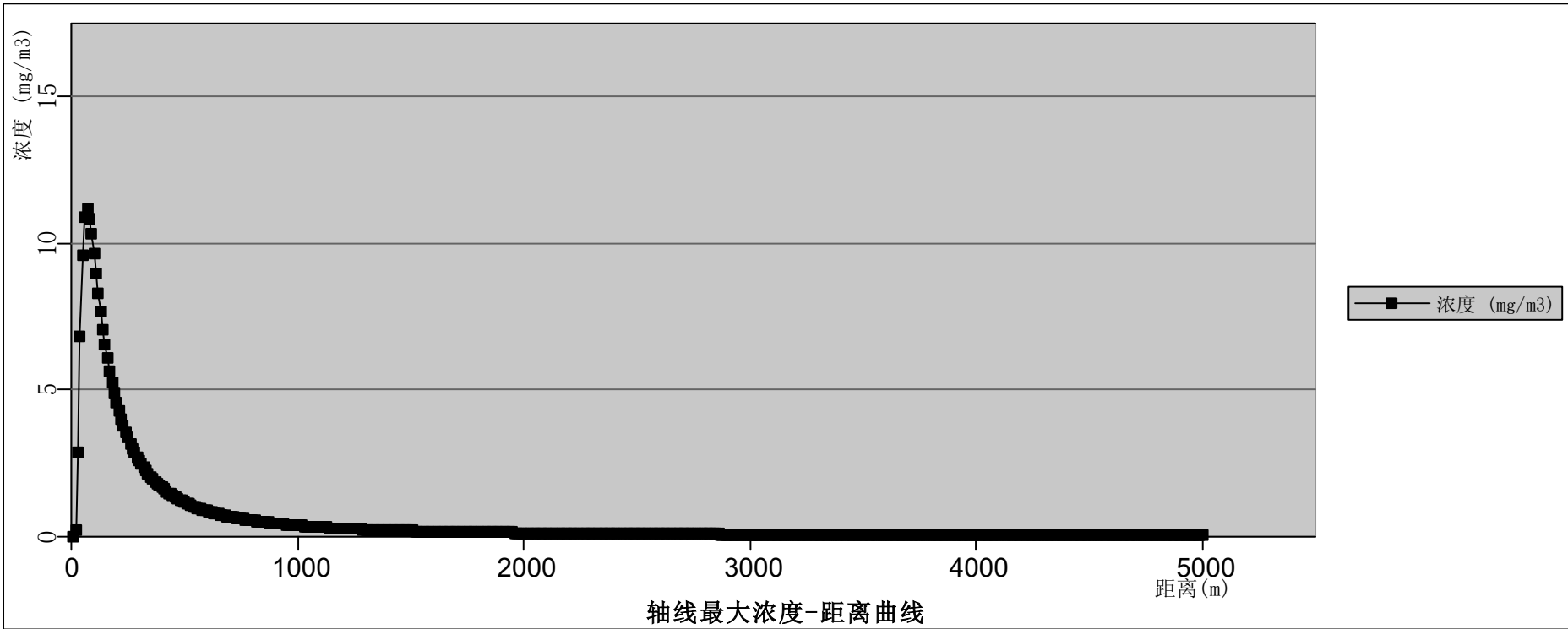
图 12.6-13 回流罐泄漏乙苯扩散轴线最大浓度——距离曲线（最不利气象条件下）
