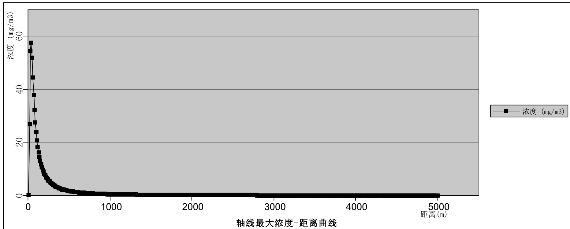
图 12.6-70 粗苯罐泄漏苯扩散轴线最大浓度——距离曲线（最常见气象条件）
