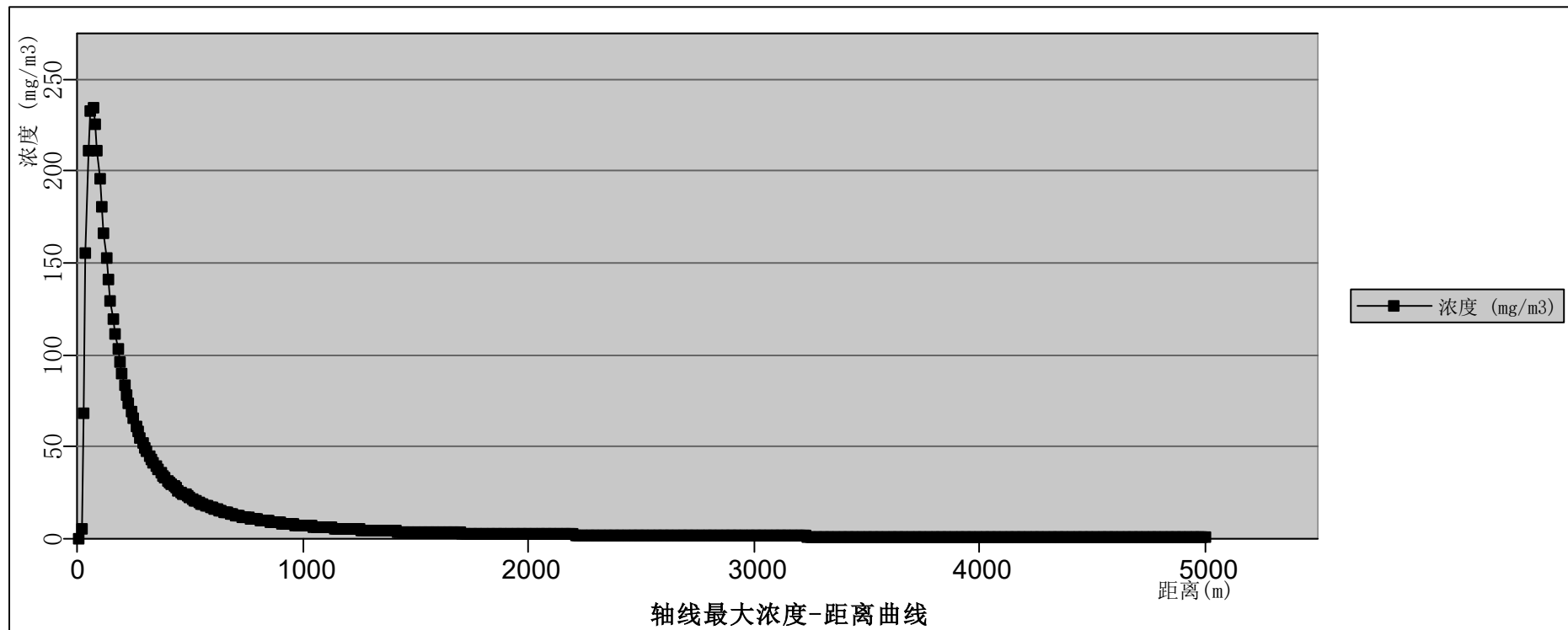
图 12.6-9 回流罐泄漏二甲苯扩散轴线最大浓度——距离曲线（最不利气象条件下）
