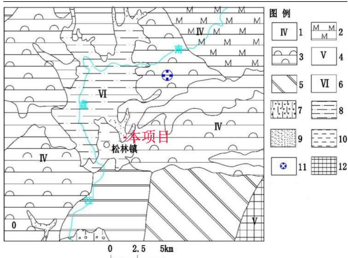
1. 岩溶地貌 2. 峰丛洼地 3. 垅岗谷地 4. 构造溶蚀地貌 5. 中山 6. 湖泊堆积地貌 7. 断拗（陷）盆地 8. 溶蚀盆地 9. 侵蚀（溶蚀）谷地 10. 湖积台地 11. 有水溶 洞 12. 残留高原面
