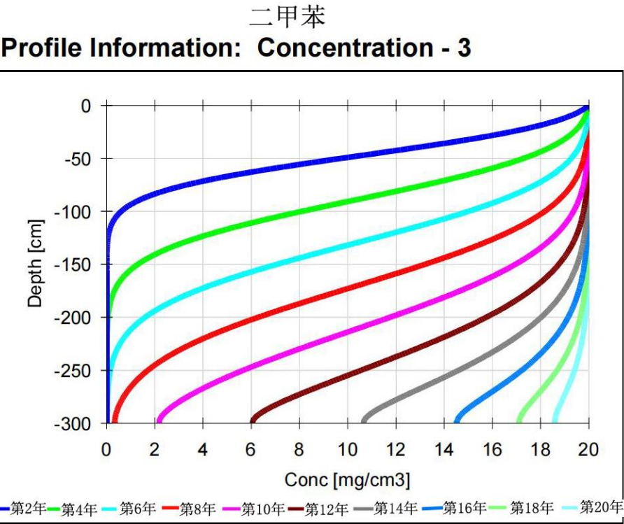
图 10.3-6 土壤不同年份不同深度二甲苯浓度变化曲线
