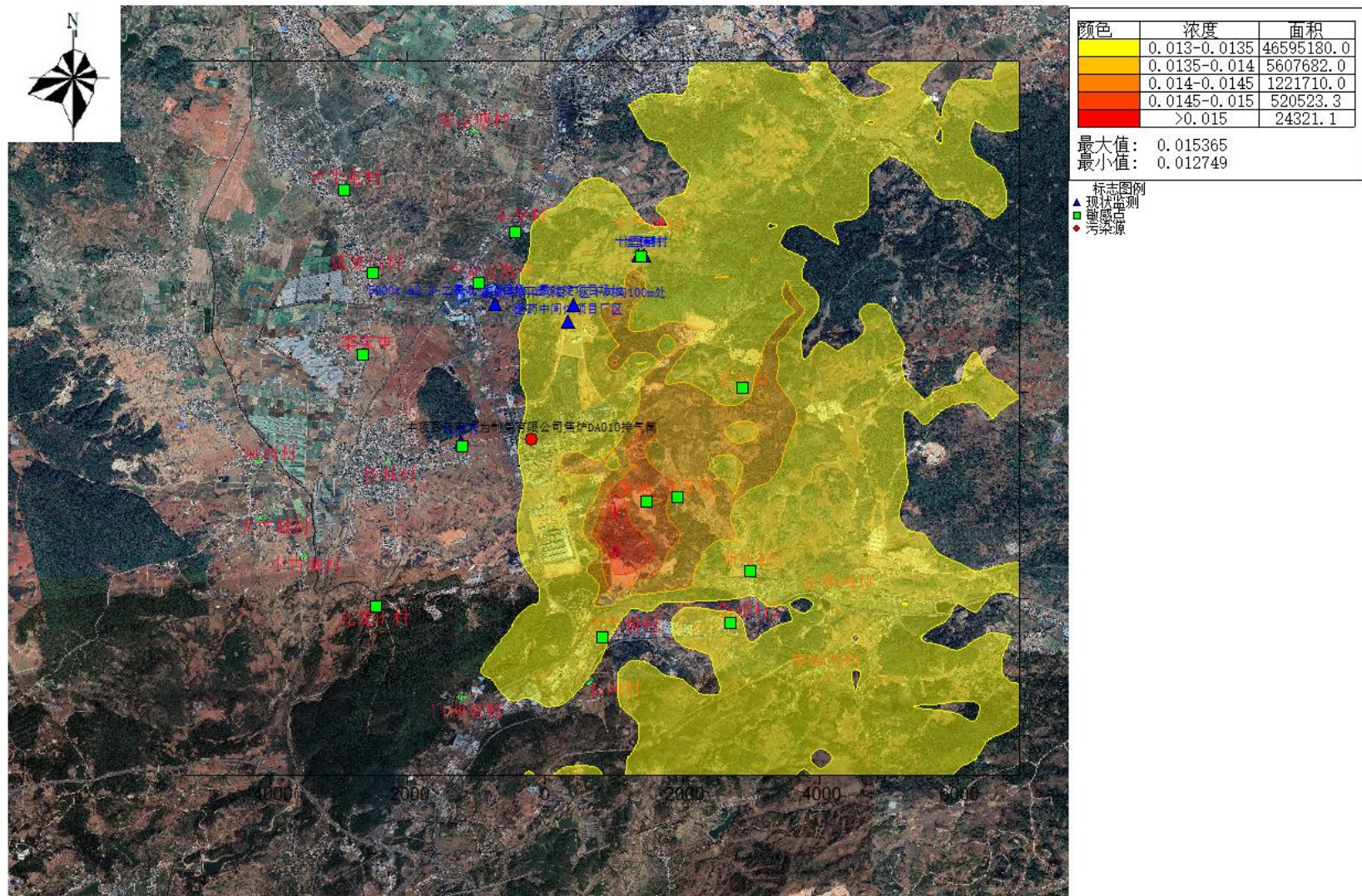
图5.2-14 全时段质量浓度分布图
