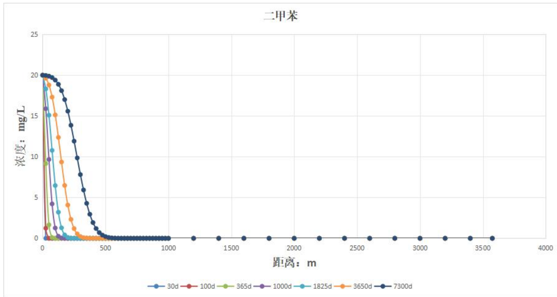
图7.9-3 管道渗漏后二甲苯浓度变化图（标准值为0.5mg/L）
