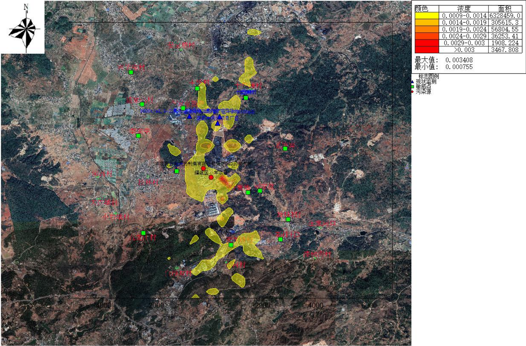
图5.2-12 二甲苯1h平均质量浓度分布图
