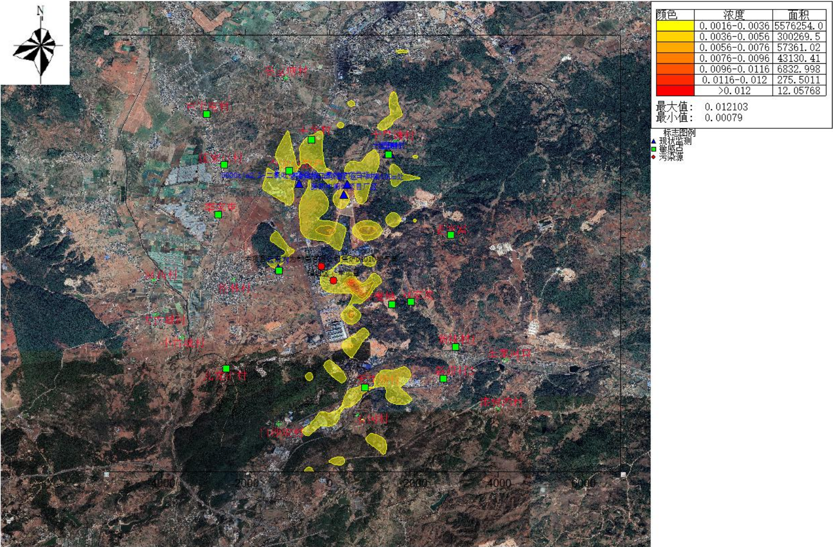
图5.2-10 苯1h平均质量浓度分布图
