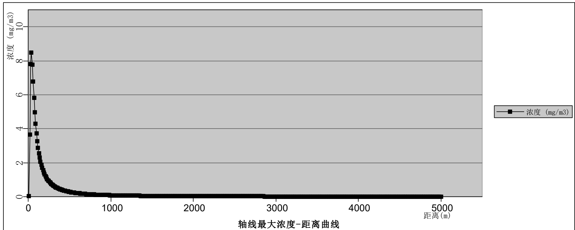
图 12.6-14 回流罐泄漏乙苯扩散轴线最大浓度——距离曲线（最常见气象条件）
