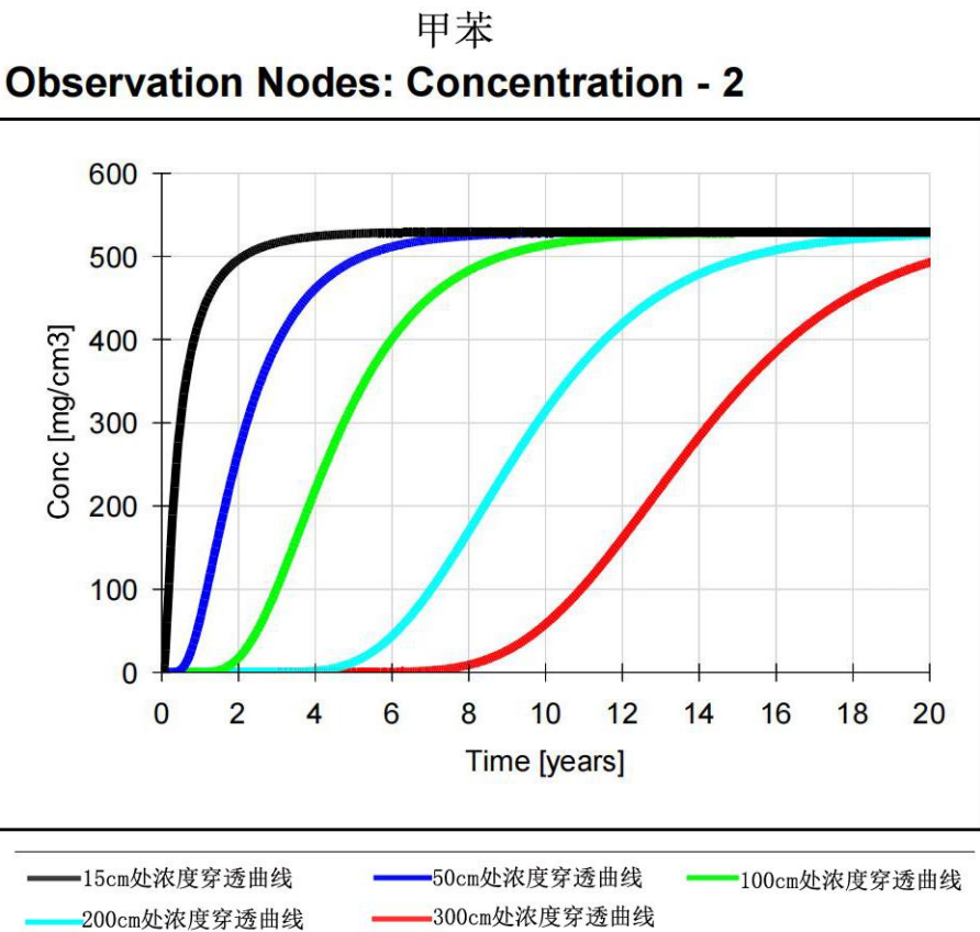
图 10.3-3 土壤不同深度处甲苯浓度变化曲线
