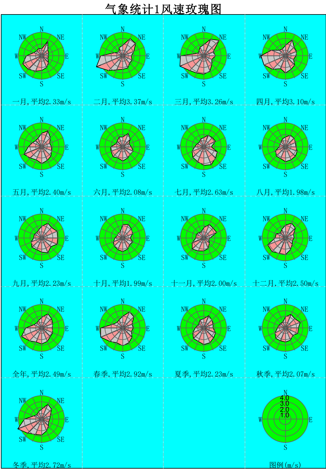
图 5.2-2 沾益区 2024 年风向风速月、季、年均玫瑰图 (1) 平均风速的月变化
