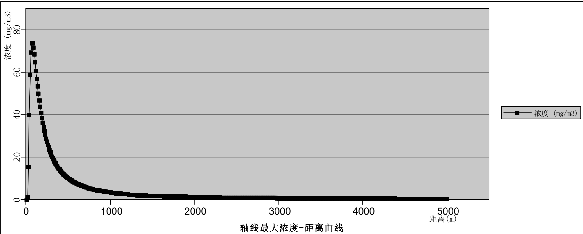
图 12.6-55 粗苯罐泄漏乙苯扩散轴线最大浓度——距离曲线（最不利气象条件下）
