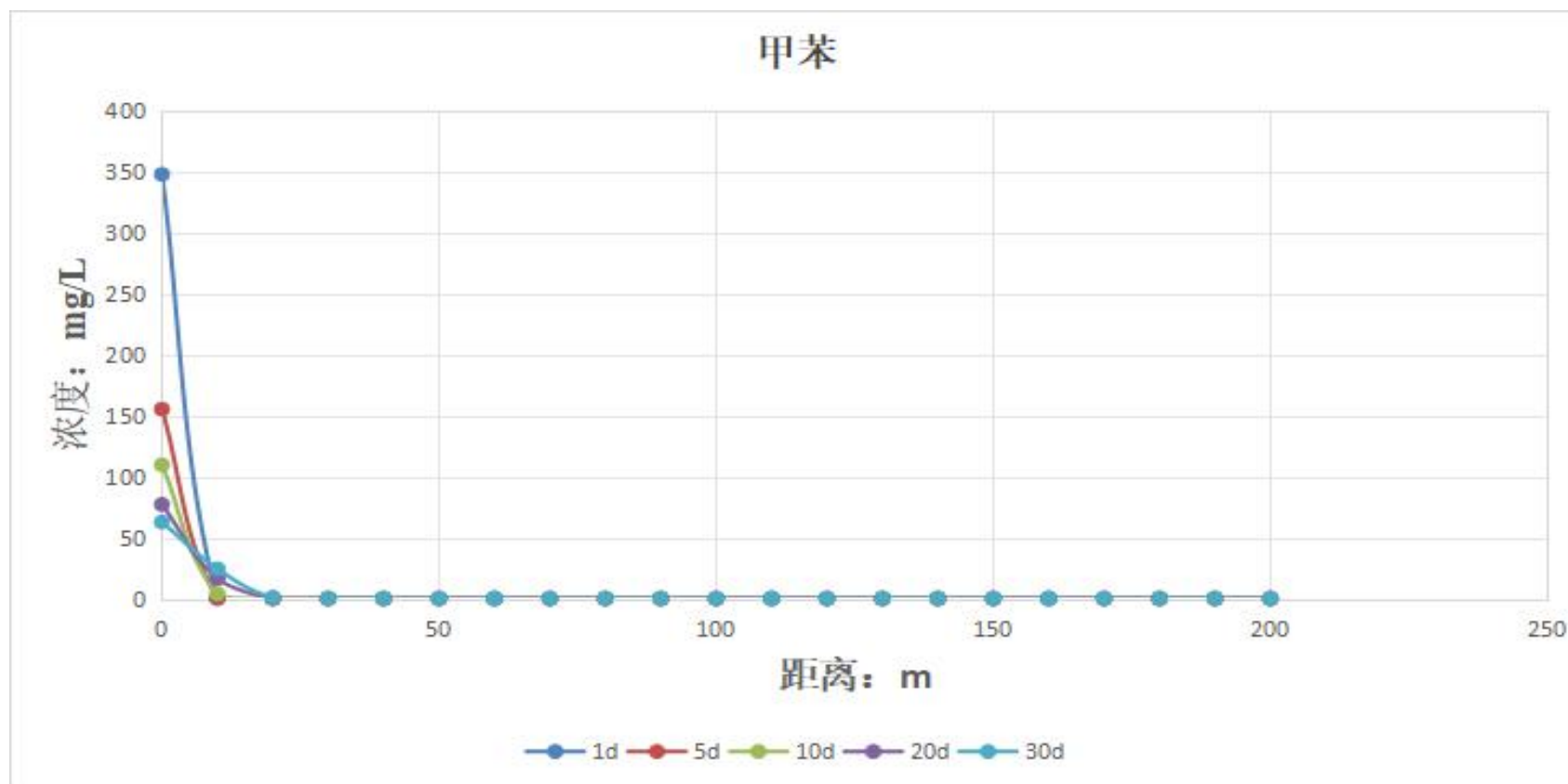
图12.6-91 回流罐泄漏甲苯下渗后浓度变化图（标准值为0.7mg/L）
