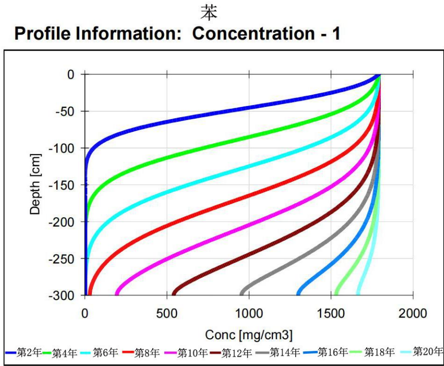
图 10.3-2 土壤不同年份不同深度苯浓度变化曲线
