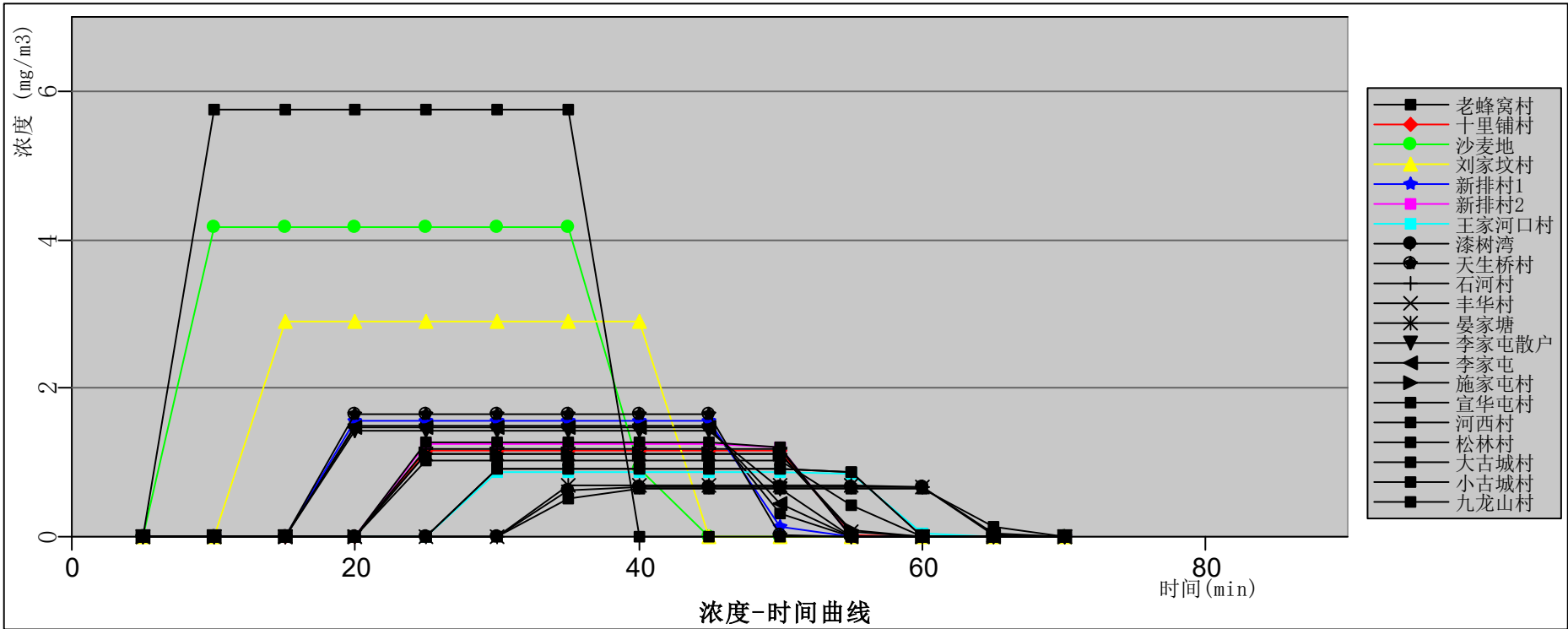
图12.6-78 粗苯罐火灾爆炸最常见气象条件各敏感点处CO浓度随时间变化曲线图
