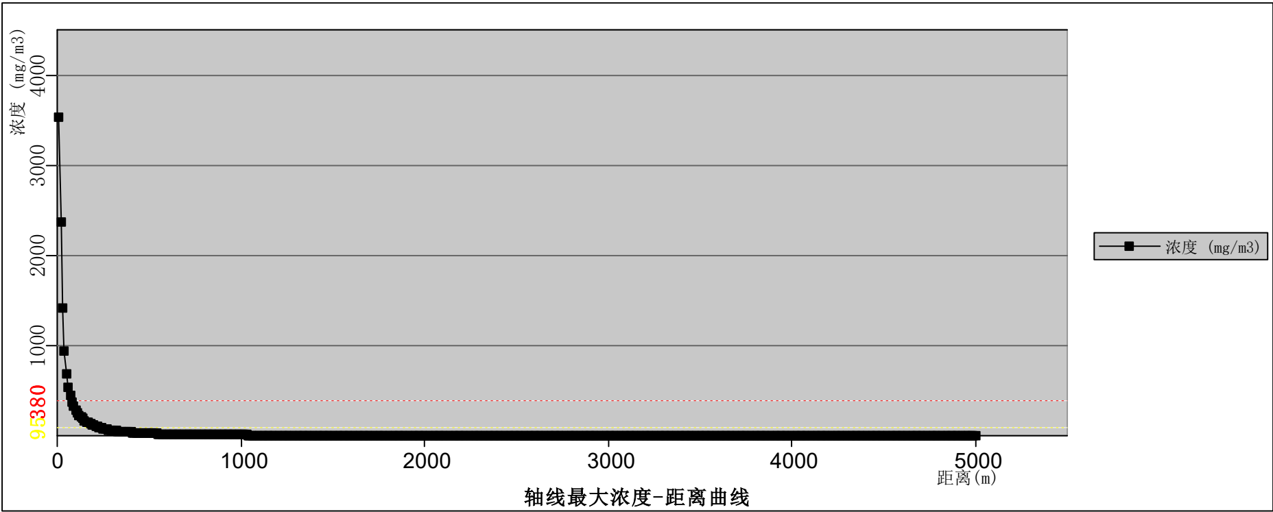
图 12.6-74 粗苯罐火灾爆炸 CO 扩散轴线最大浓度——距离曲线（最常见气象条件）
