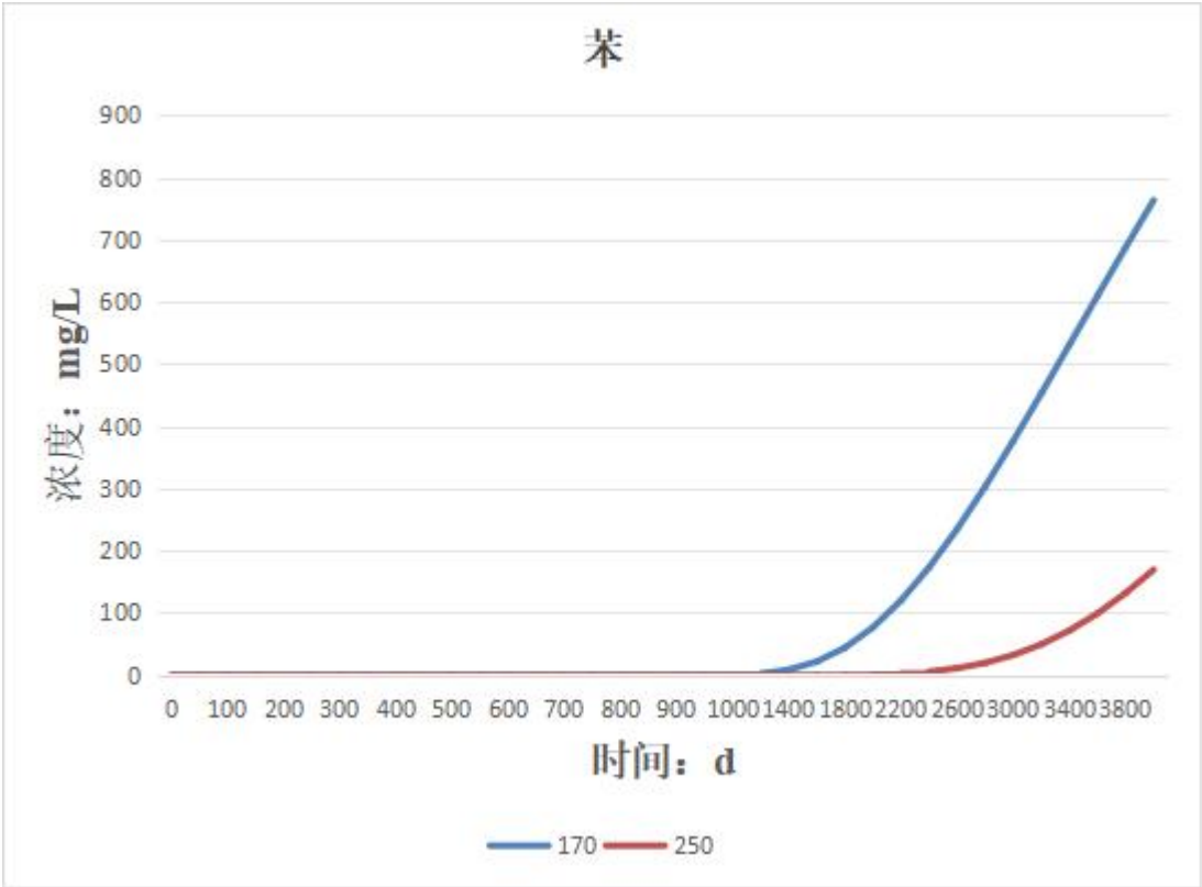
图 7.9-5 固定位置地下水中苯污染物（监测井和最近厂界处）浓度穿透曲线图
