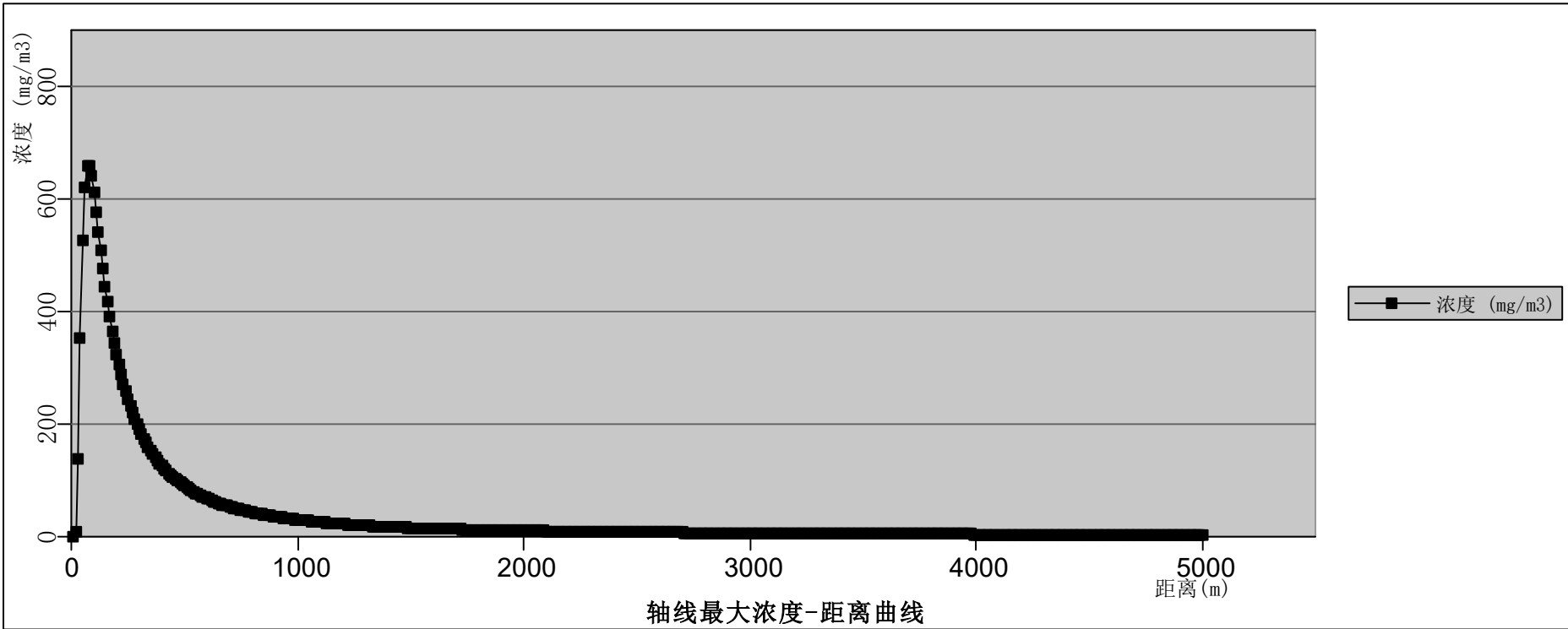
图 12.6-65 粗苯罐泄漏环己烷扩散轴线最大浓度——距离曲线（最不利气象条件下）
