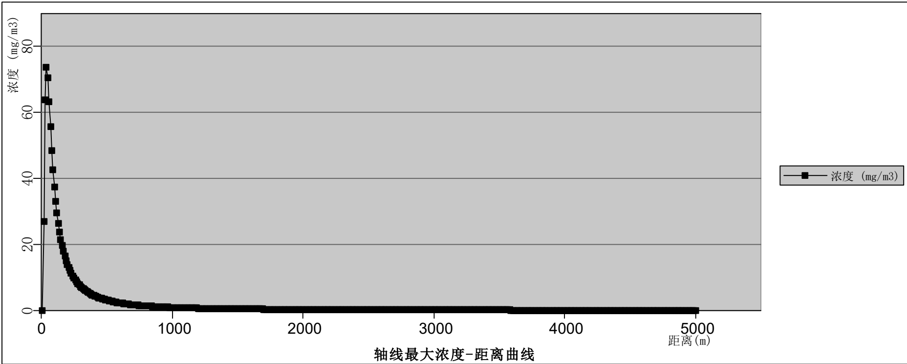
图 12.6-56 粗苯罐泄漏乙苯扩散轴线最大浓度——距离曲线（最常见气象条件）
