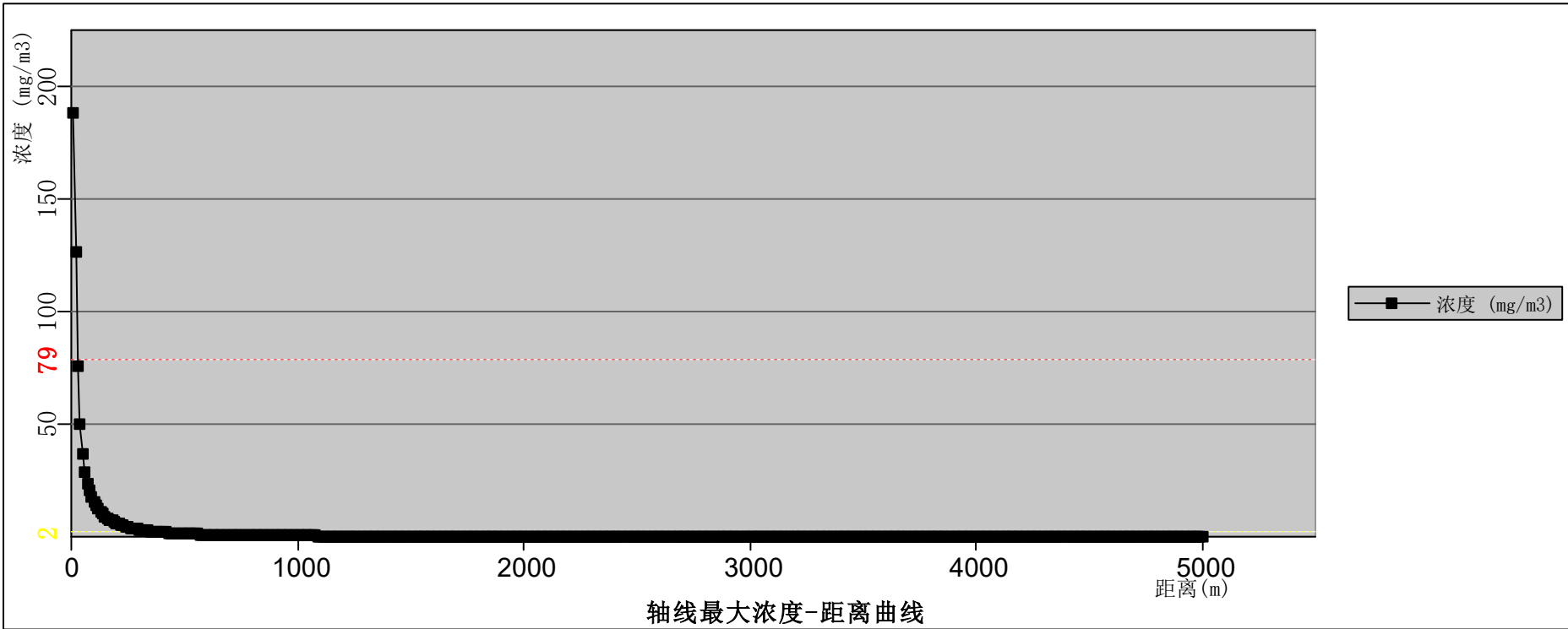
图 12.6-36 回流罐火灾爆炸 SO 2 扩散轴线最大浓度——距离曲线（最常见气象条件）
