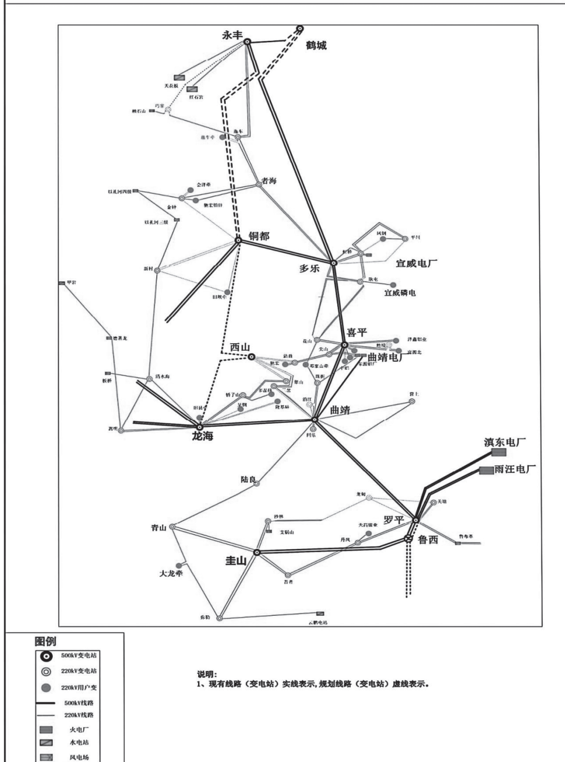
附图2：曲靖市“十四五”电力电网重点项目布局示意图
