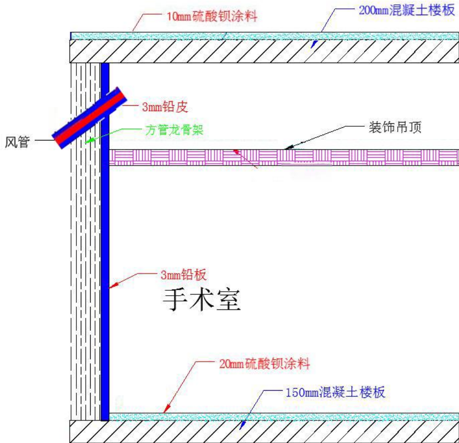
图 10-3 风管穿墙示意图
