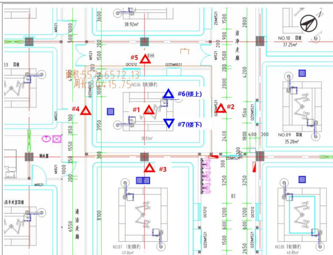
图 8-1 移动式 C 形臂 X 射线机机房及周围 \gamma 辐射空气吸收剂量率监测点位图
