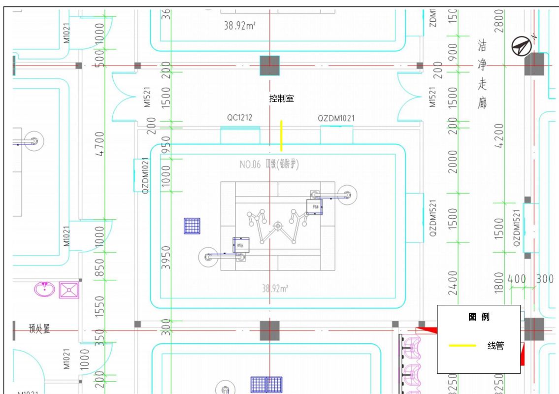
图 10-3 供电线管平面布局示意图
