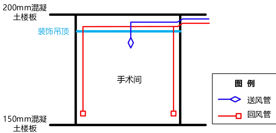
图 10-3 风管布局剖面示意图
