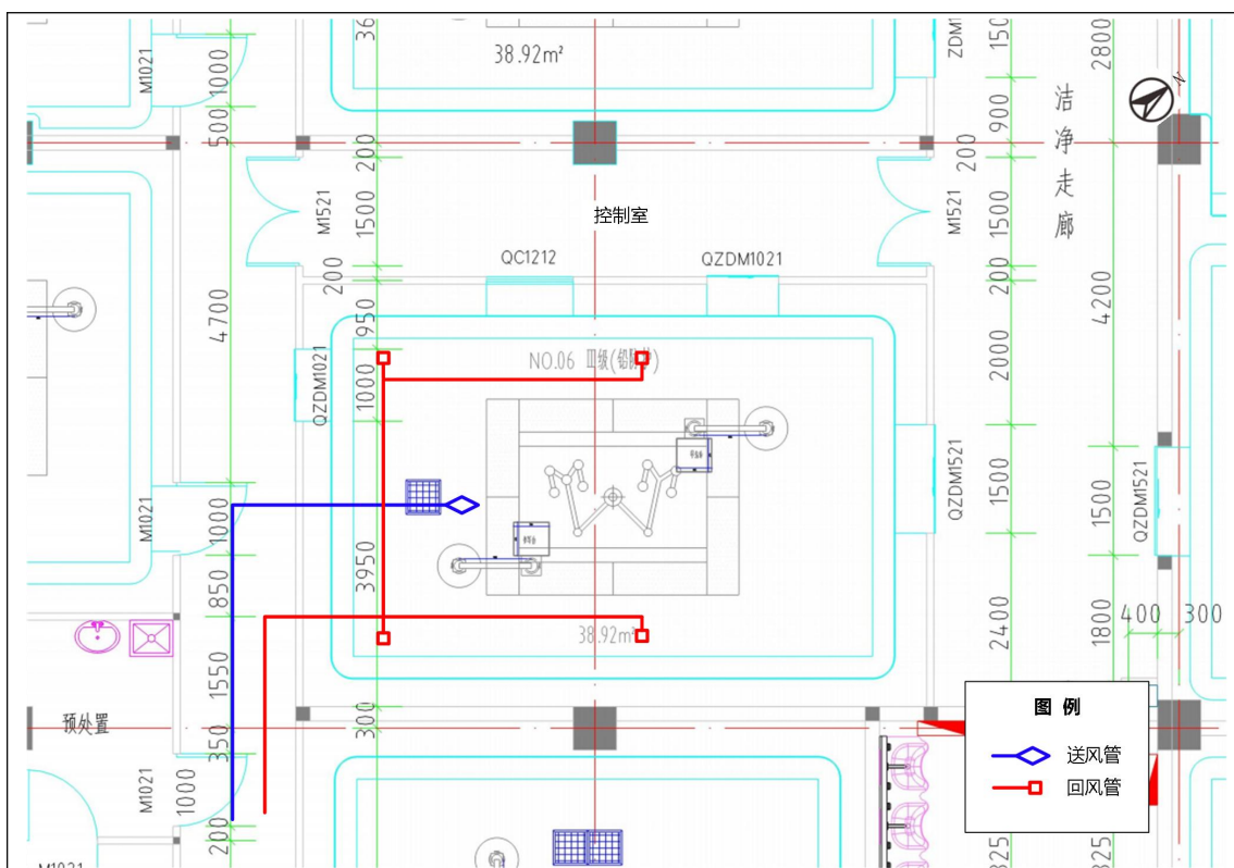
图 10-3 风管平面布局示意图
