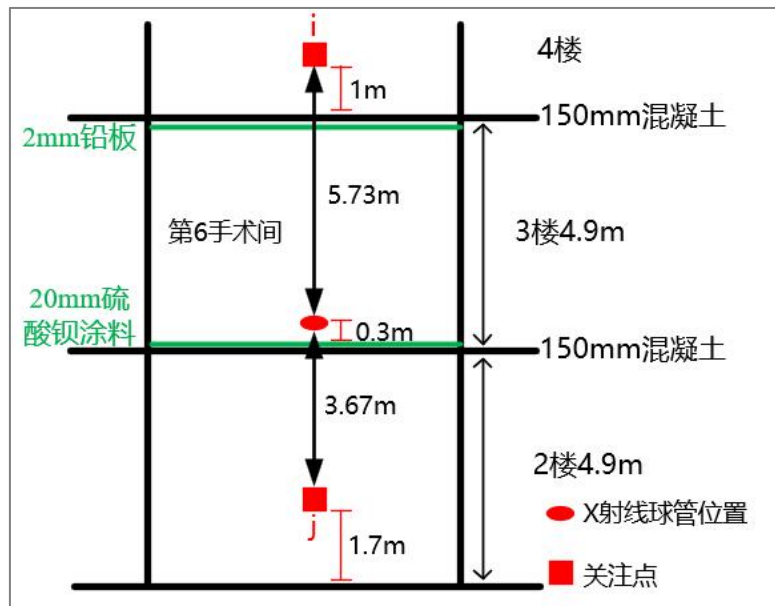
图 11-2 机房楼上楼下关注点位置示意图
