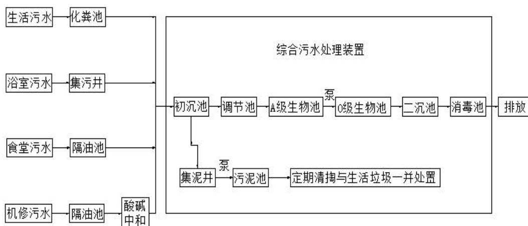
图 14.2-2 生活污水处理工艺流程图
