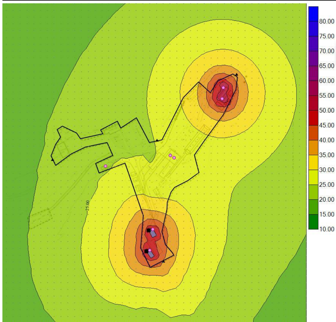
图 10.2-2 主井工业场地夜间噪声贡献值等值线图
