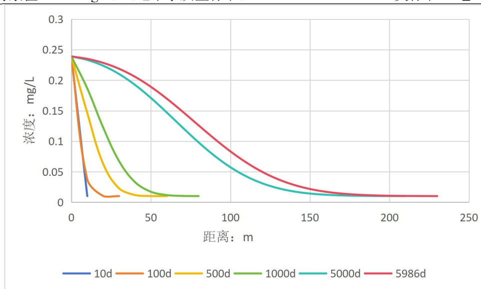
矿井水处理站下游地下水中 Mn 浓度扩散曲线图
