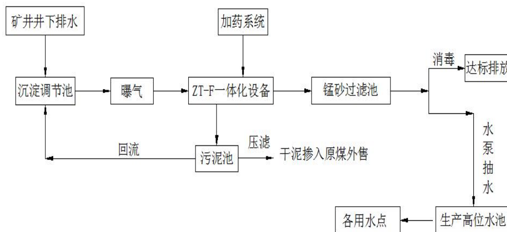
图 14.2-1 矿井水处理工艺流程图
