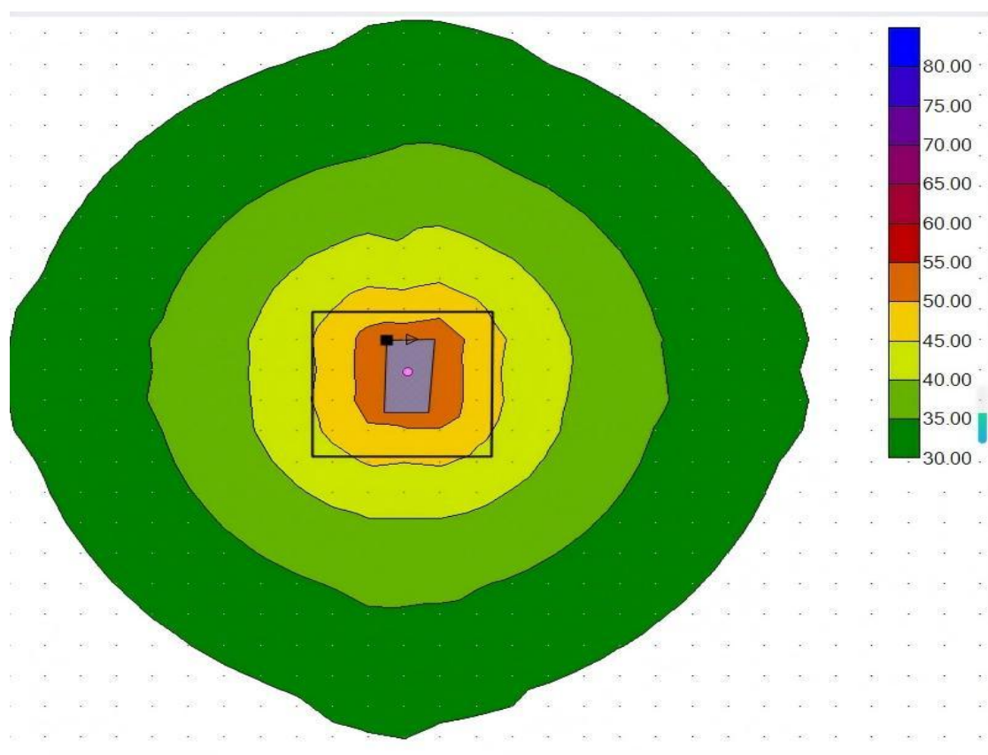
图 10.2-3 前期风井工业场地昼夜噪声贡献值等值线图
