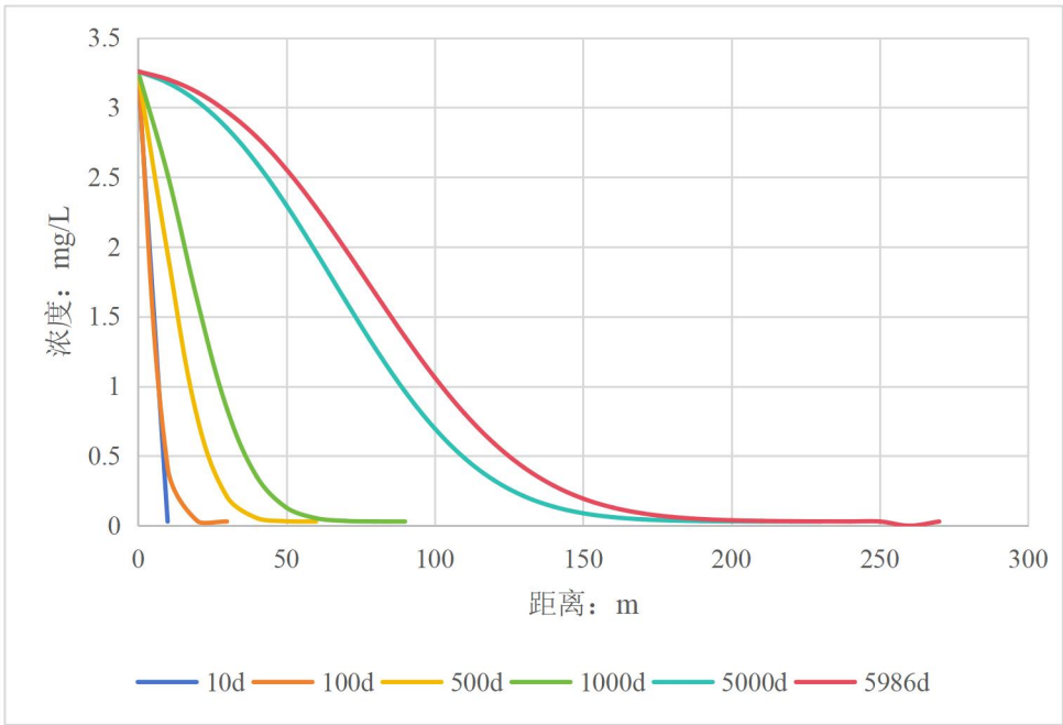
矿井水处理站下游地下水中 Fe 浓度扩散曲线图
