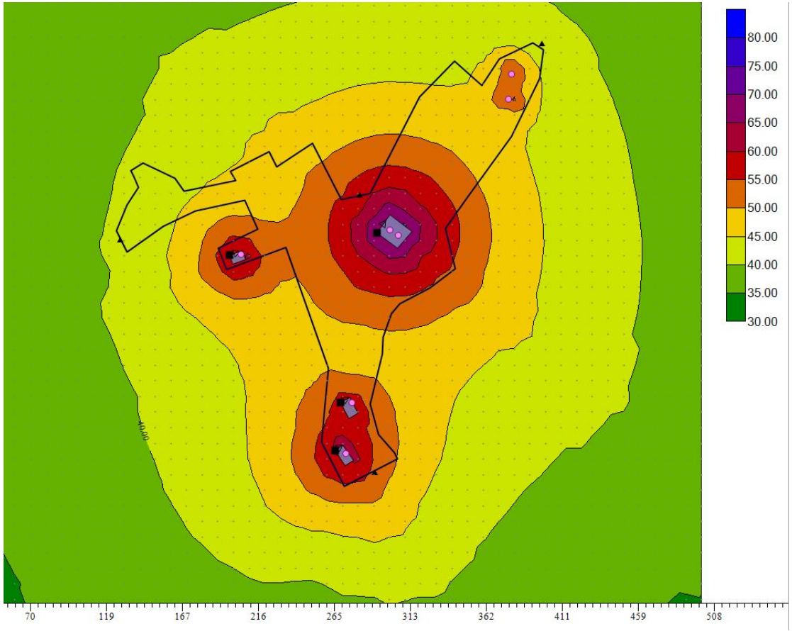
图 10.2-1 主井工业场地昼间噪声贡献值等值线图
