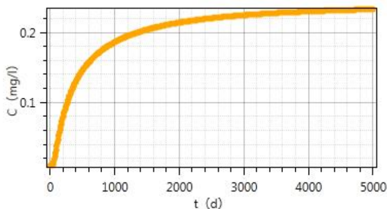
跟踪观测井处 Mn 浓度穿透曲线图
