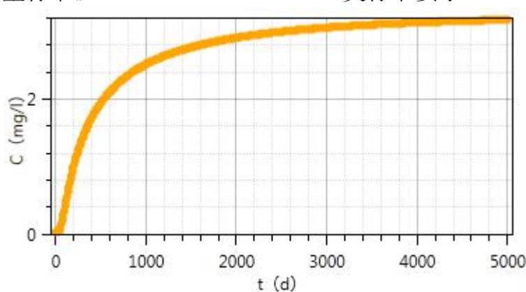
跟踪观测井处 Fe 浓度穿透曲线图
